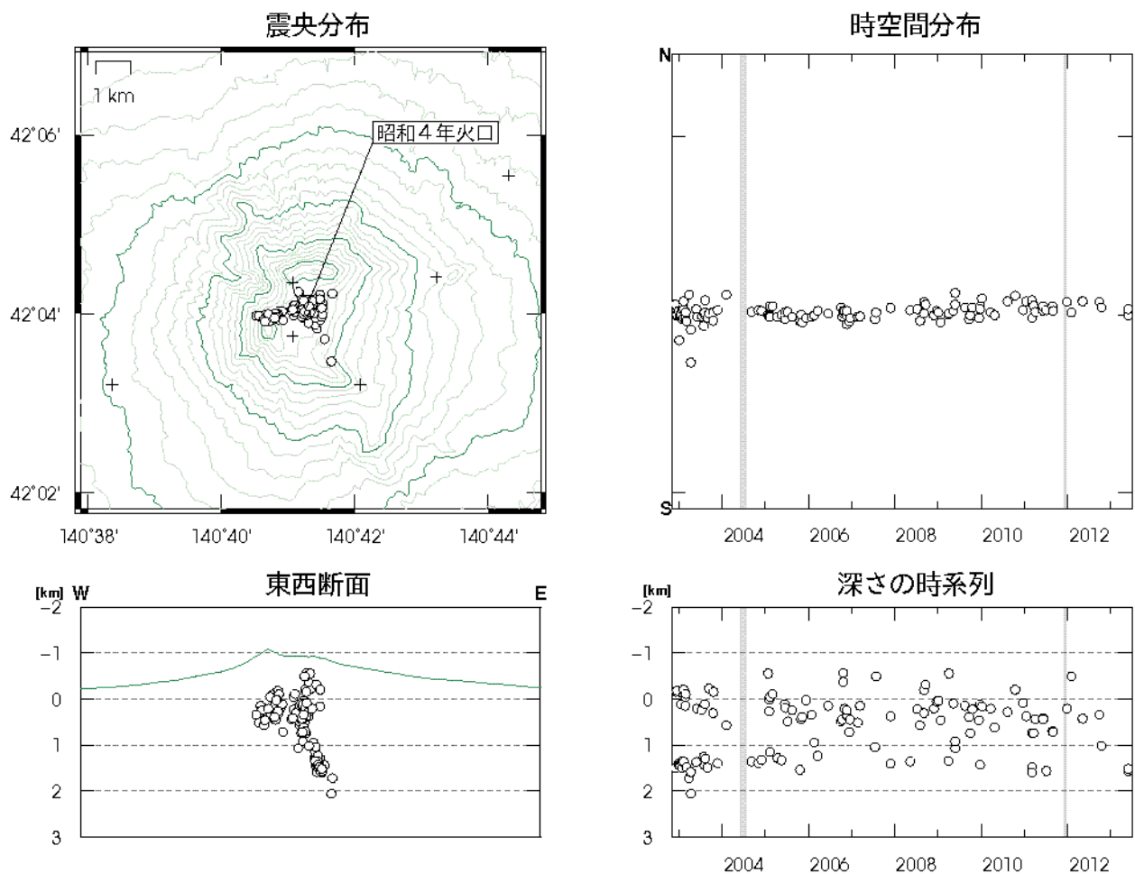
図3 北海道駒ヶ岳 火山性地震の震源分布（2002年11月～2013年6月） 灰色の期間は一部観測点欠測のため震源の決定数減少や精度低下が見られます ○印：2002年11月～2013年5月の震源 +印：地震観測点 ・今期間、震源が決定された地震はありませんでした
