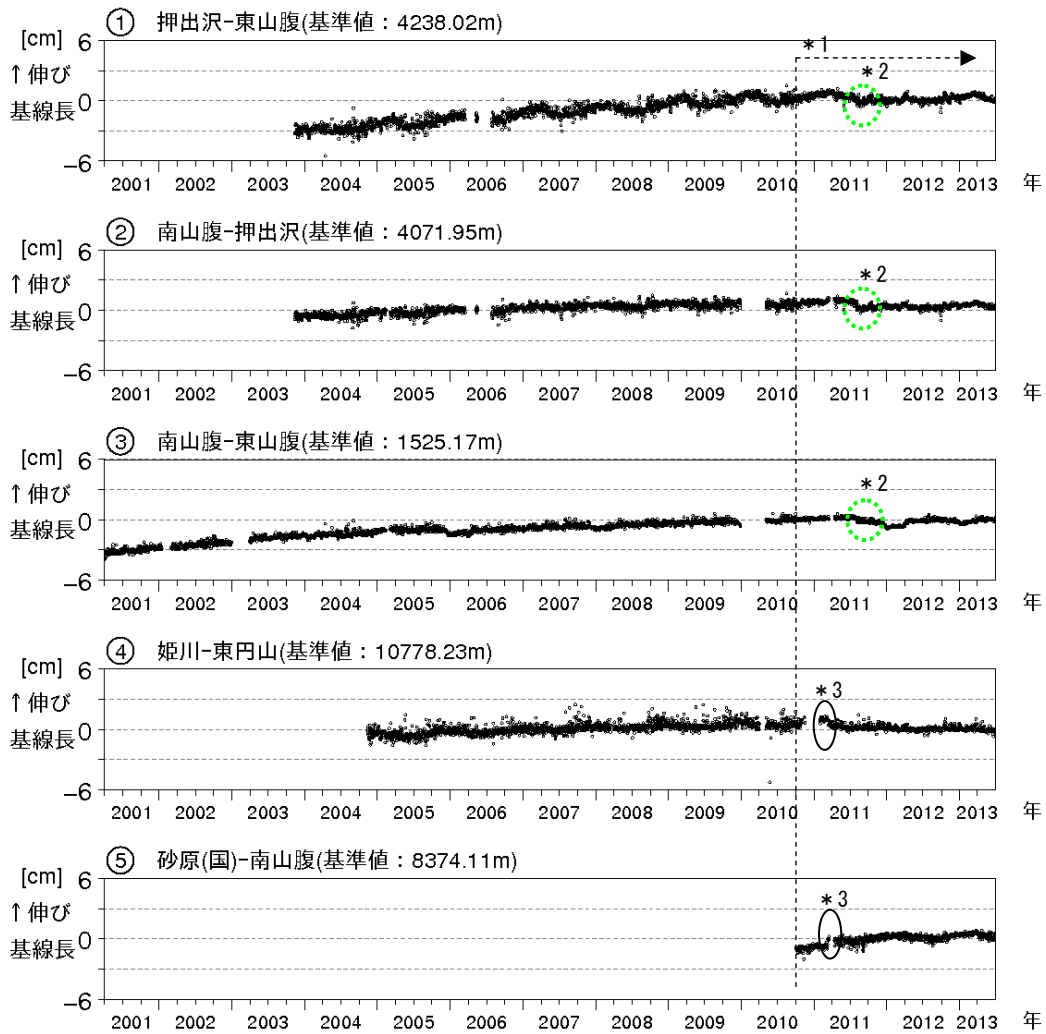
図4 北海道駒ヶ岳 GPS連続観測による基線長変化 (2001年4月~2013年6月) ・グラフの空白部分は欠測 GPS基線①~⑤は図5の①~⑤に対応しています * 1 : 2010年10月以降のデータについては、解析方法を改良して精度を向上させています * 2 : 緑点線円内の変動は、機器更新による * 3 : 楕円内の変動は、2011年3月11日に発生した東北地方太平洋沖地震の影響によるものであり、火山活動によるものではありません
