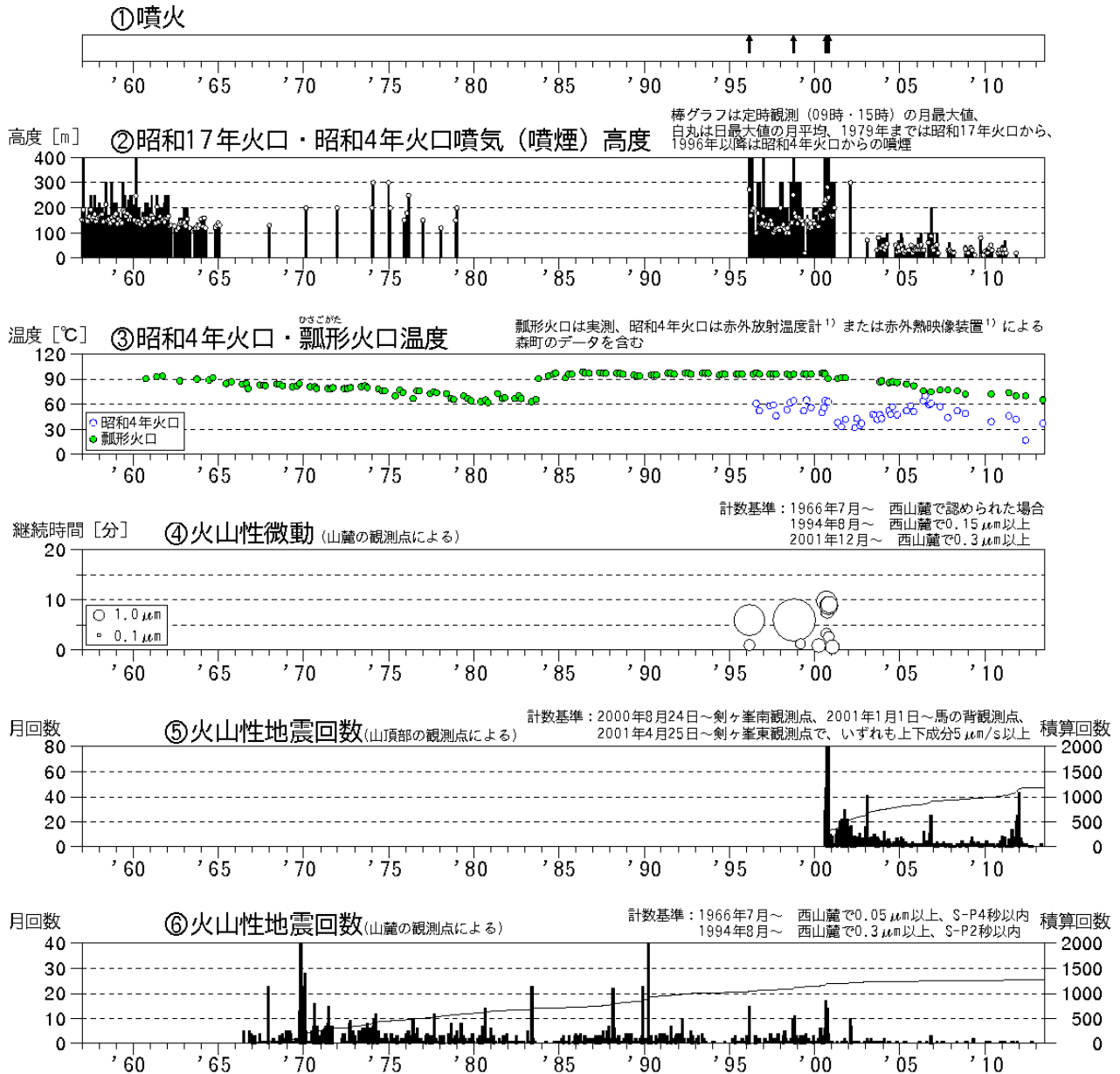
図1 北海道駒ヶ岳 火山活動経過図 (1957年1月～2013年6月)
