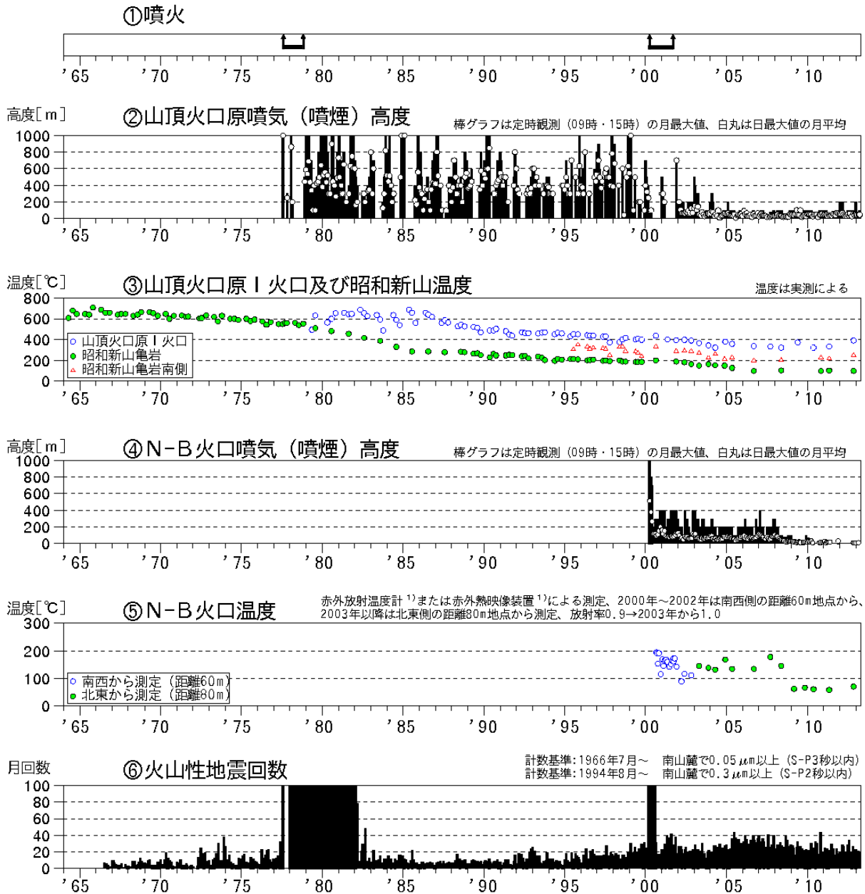
図 1※ 有珠山 火山活動経過図（1964年 1 月～2013年 4 月）
