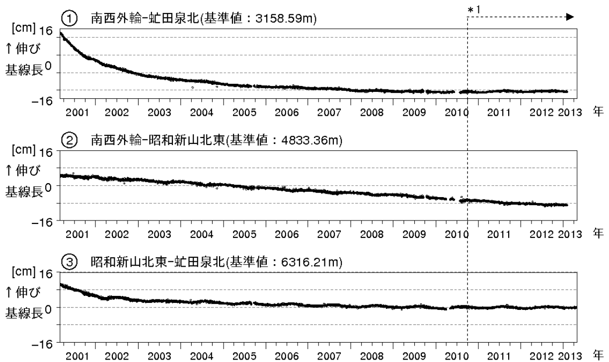
図 4 有珠山 GPS連続観測による基線長変化 (2001年3月~2013年4月)
