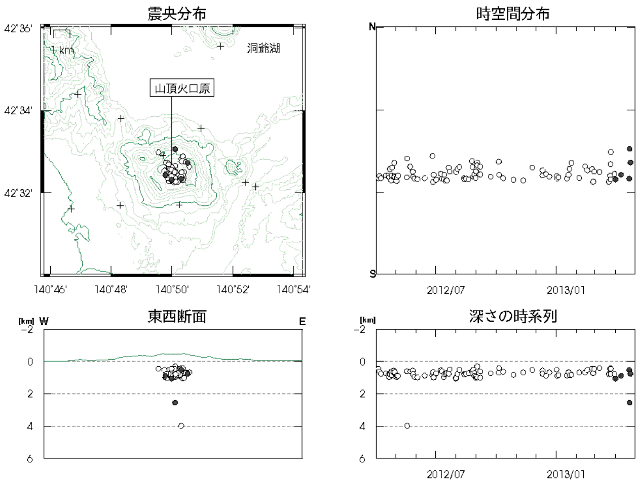
図 3 有珠山 火山性地震の震源分布（2012年4月～2013年4月）
