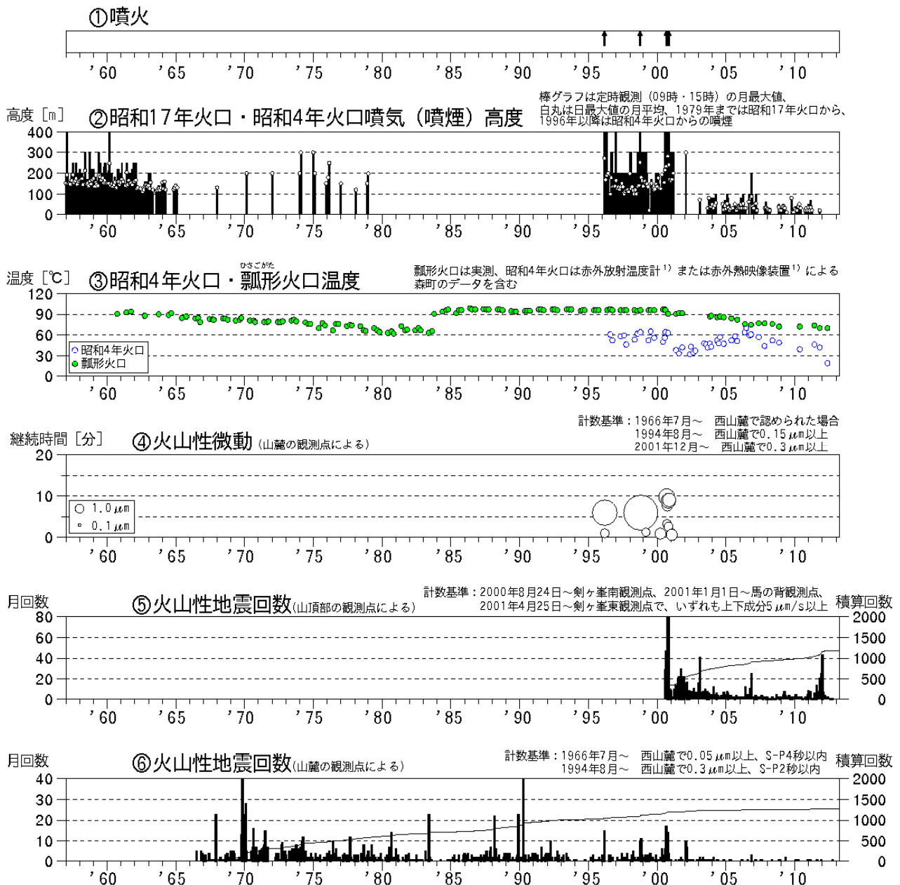
図 1 ※ 北海道駒ヶ岳 火山活動経過図（1957年 1 月～2013年 3 月）
