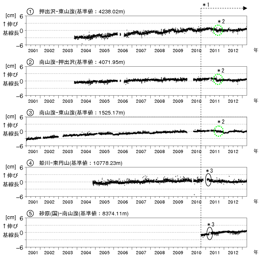
図 4 ※ 北海道駒ヶ岳 GPS連続観測による基線長変化（2001年 4 月～2013年 3 月）
