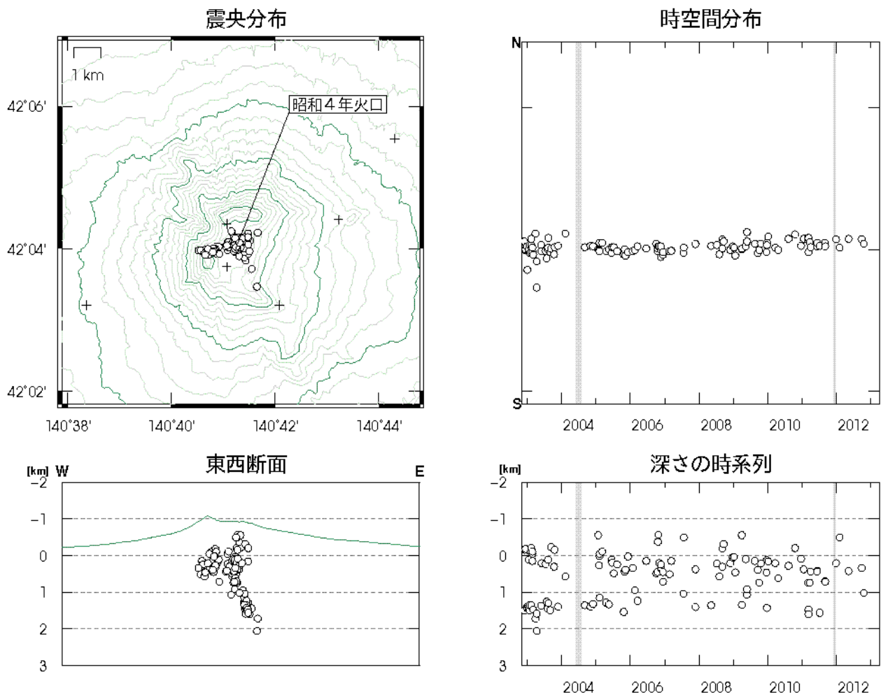
図 3※ 北海道駒ヶ岳 火山性地震の震源分布（2002年11月～2013年3月） 灰色の期間は一部観測点欠測のため震源の決定数減少や精度低下が見られます ○印：2002年11月～2013年2月の震源 ＋印：地震観測点
