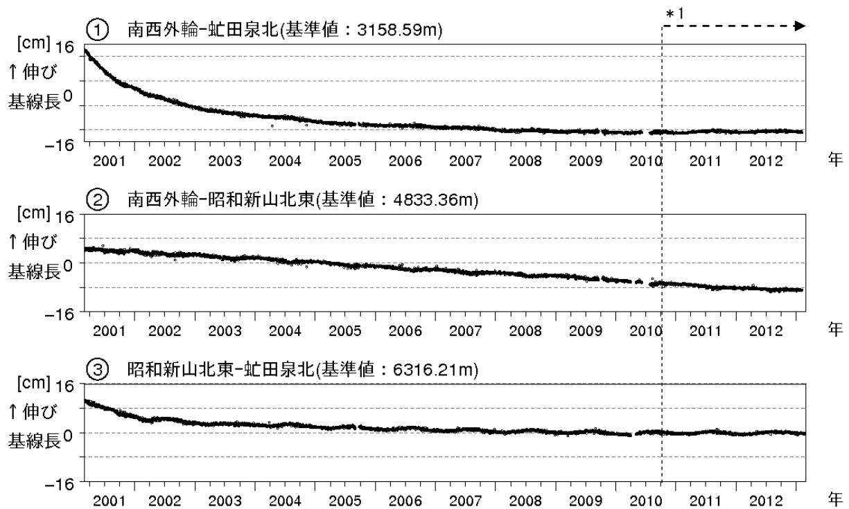
図 4 有珠山 GPS連続観測による基線長変化 (2001年3月~2013年2月) ・グラフの空白部分は欠測 GPS基線①~③は図5の①~③に対応 * 1 : 2010年10月以降のデータについては、解析方法を改良して精度を向上させています
