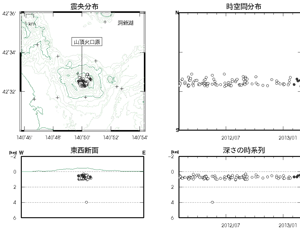
図 3 有珠山 火山性地震の震源分布（2012年2月～2013年2月）
