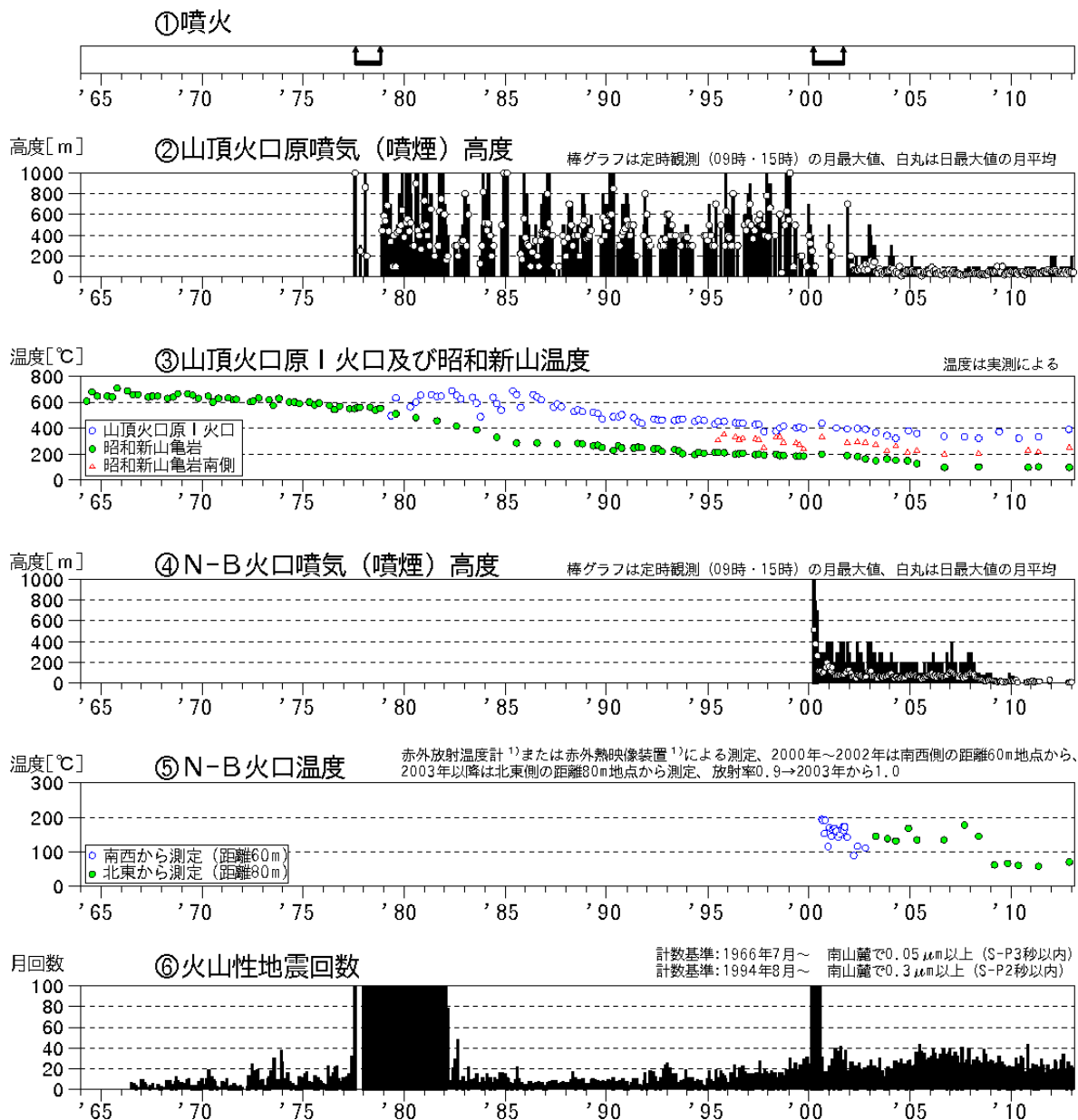
図 1 ※ 有珠山 火山活動経過図（1964年 1 月～2013年 2 月）
