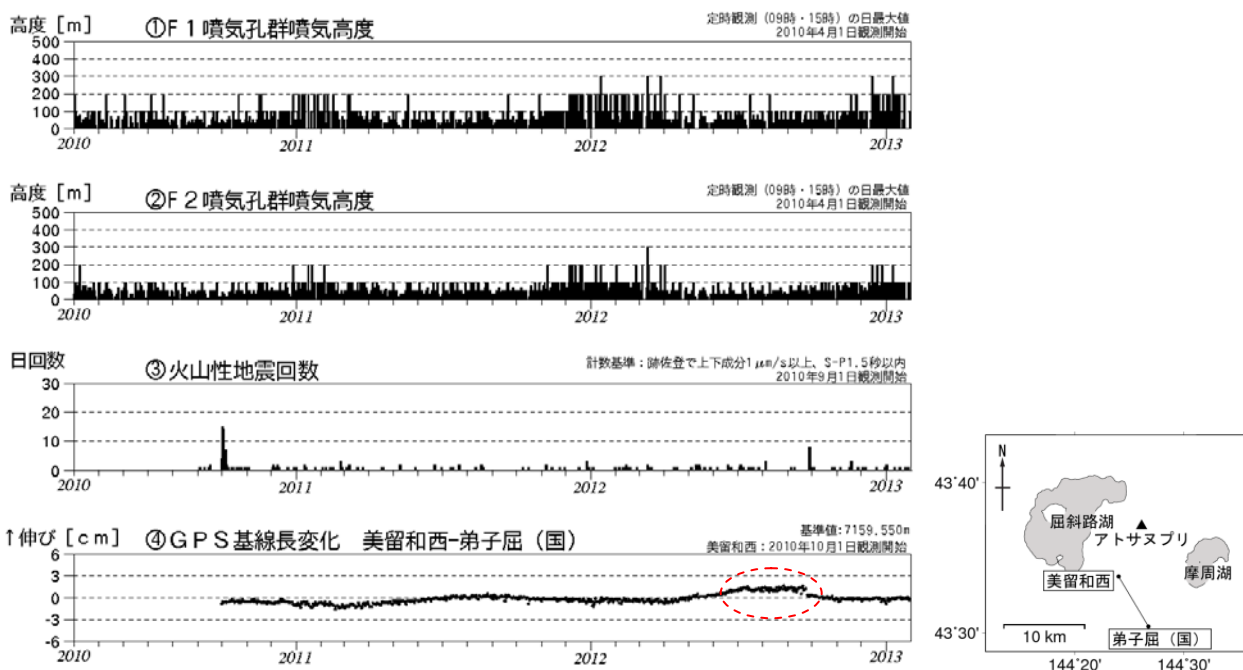
図1※ アトサヌプリ 火山活動経過図（2010年4月～2013年1月）、GPS連続観測点配置図
