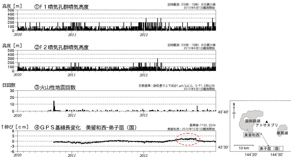
図 1 ※ アトサヌプリ 火山活動経過図（2010年 4 月～2012年12月）、GPS連続観測点配置図
