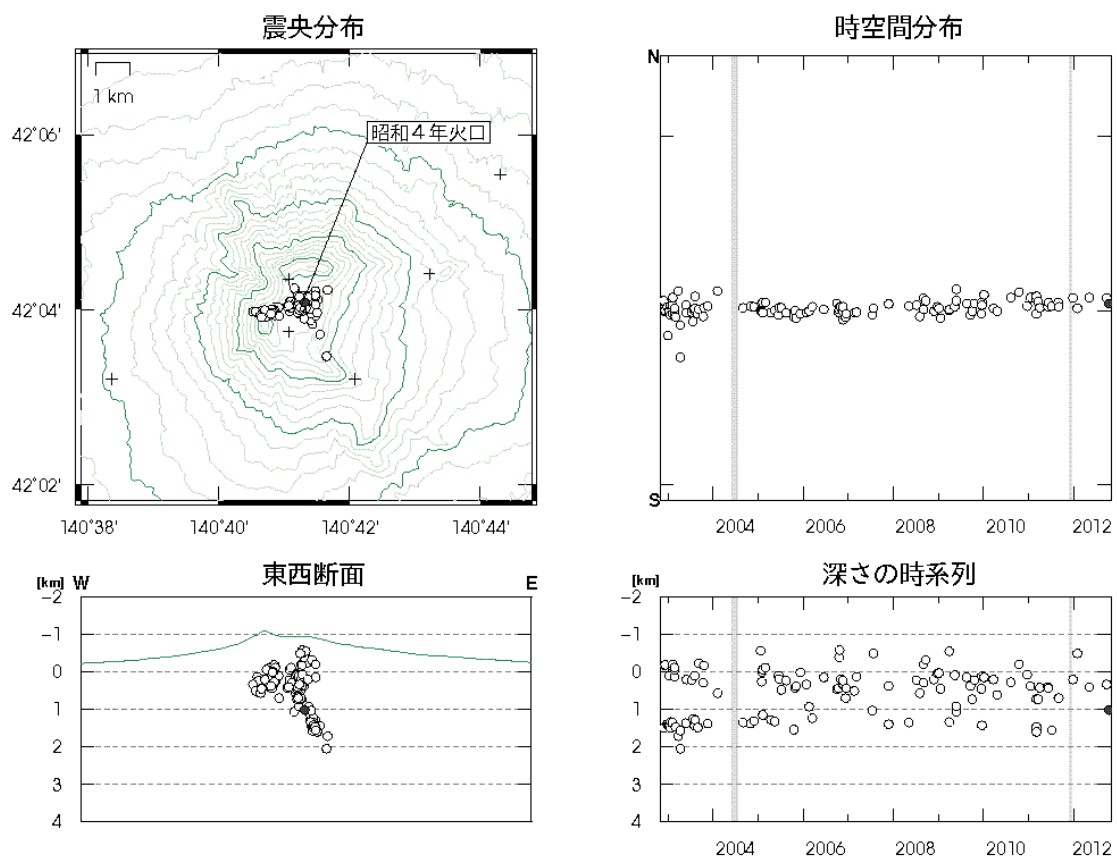
図3※ 北海道駒ヶ岳 火山性地震の震源分布（2002年12月～2012年10月） 灰色の期間は一部観測点欠測のため震源の決定数減少や精度低下が見られます ○印：2002年11月から2012年9月の震源 ●印：2012年10月の震源 +印：地震観測点
