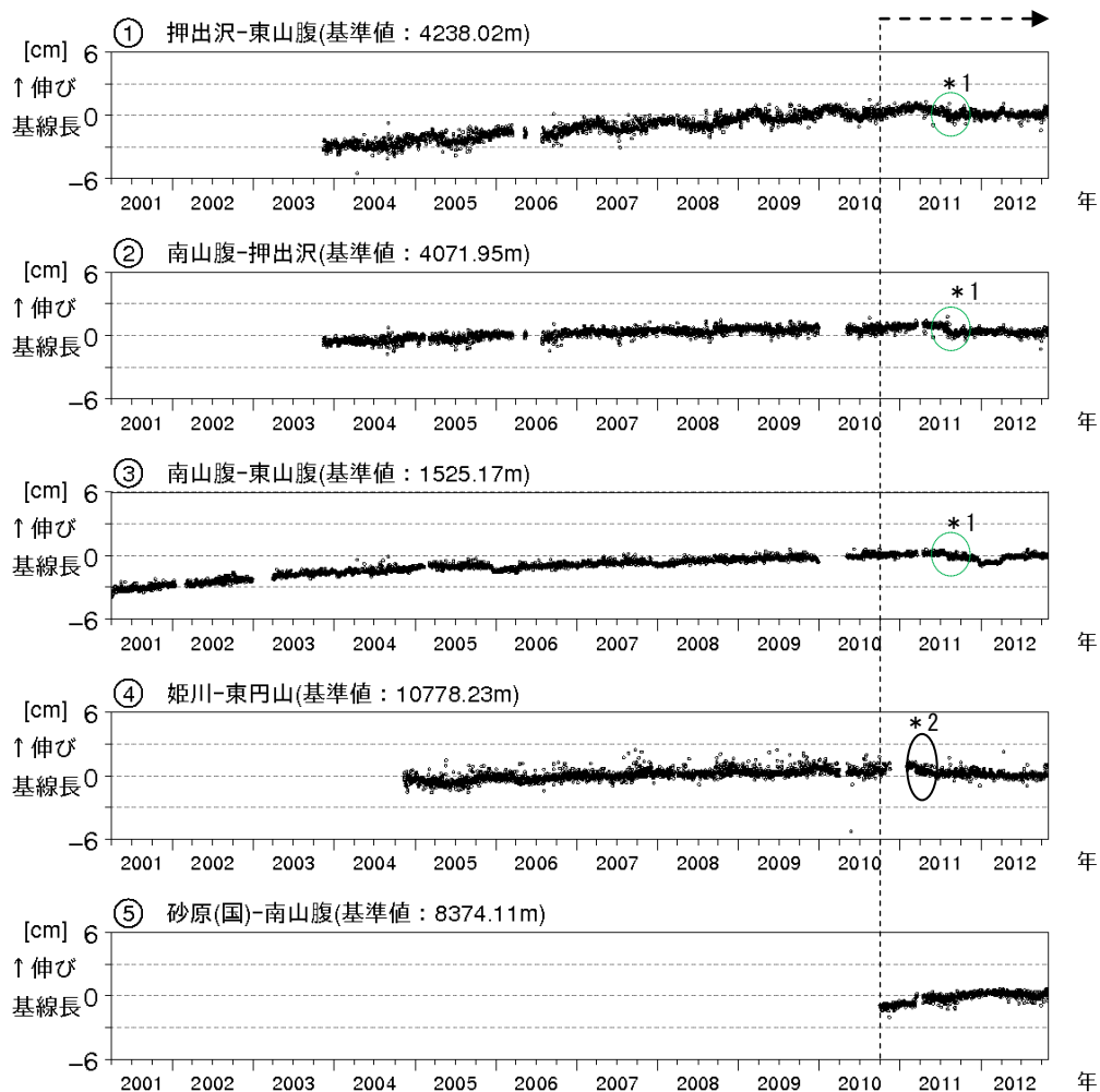
図 4 ※ 北海道駒ヶ岳 GPS連続観測による基線長変化 (2001年 4 月～2012年10月)
