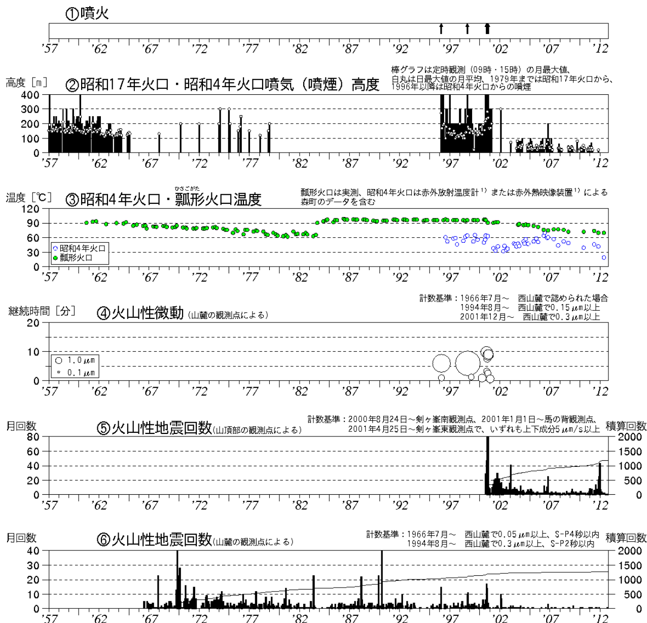
図 1※ 北海道駒ヶ岳 火山活動経過図（1957年 1 月～2012年10月）
