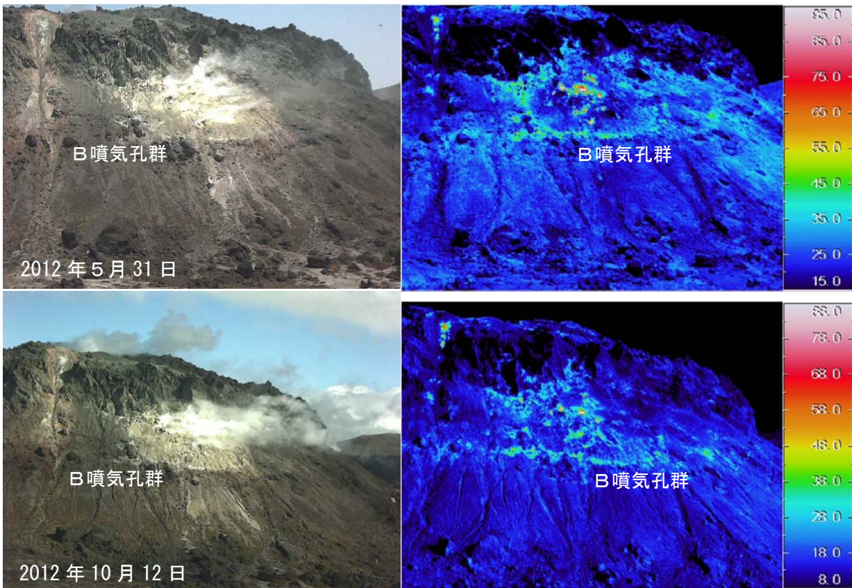
図 5 樽前山 赤外熱映像装置 1) によるB噴気孔群の地表面温度分布 (図3-②より撮影)
