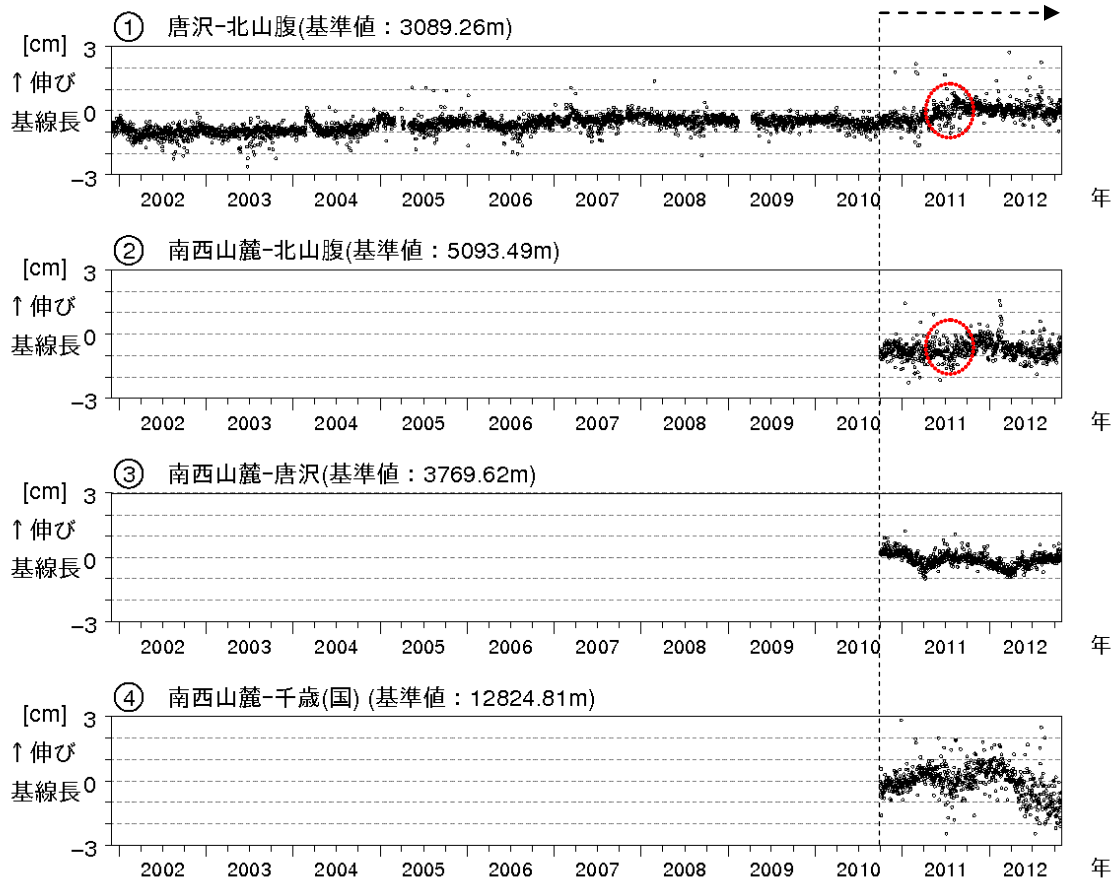
図9※ 樽前山 GPS連続観測による基線長変化(2001年12月～2012年10月) ・グラフの空白部分は欠測 GPS基線①～④は、図10の①～④に対応 ・2010年10月以降のデータについては、電離層の影響を補正する等、解析方法を改良しています。 ・赤点線円内の変動は、機器更新によるものです
