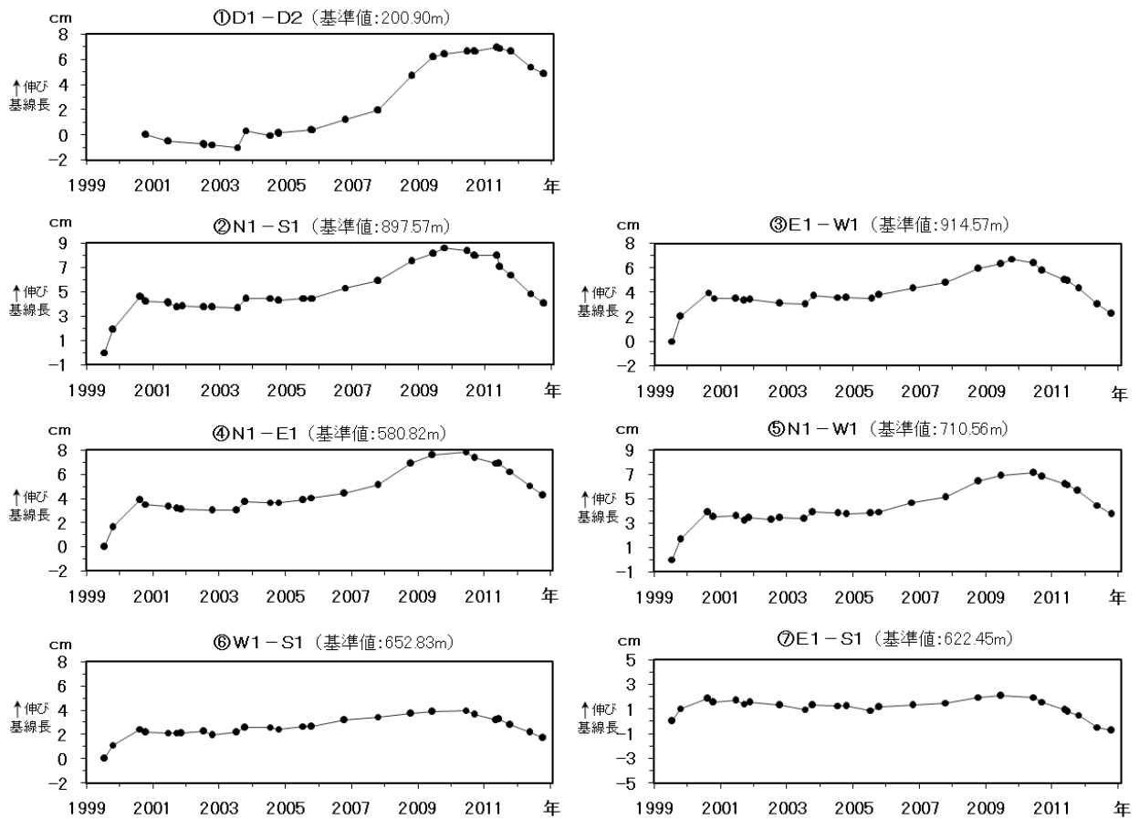
図7 樽前山 GPS 繰り返し観測による山頂溶岩ドーム付近の基線長変化 (1999 年～2012 年) GPS 基線①～⑦は図8の①～⑦に対応しています。
