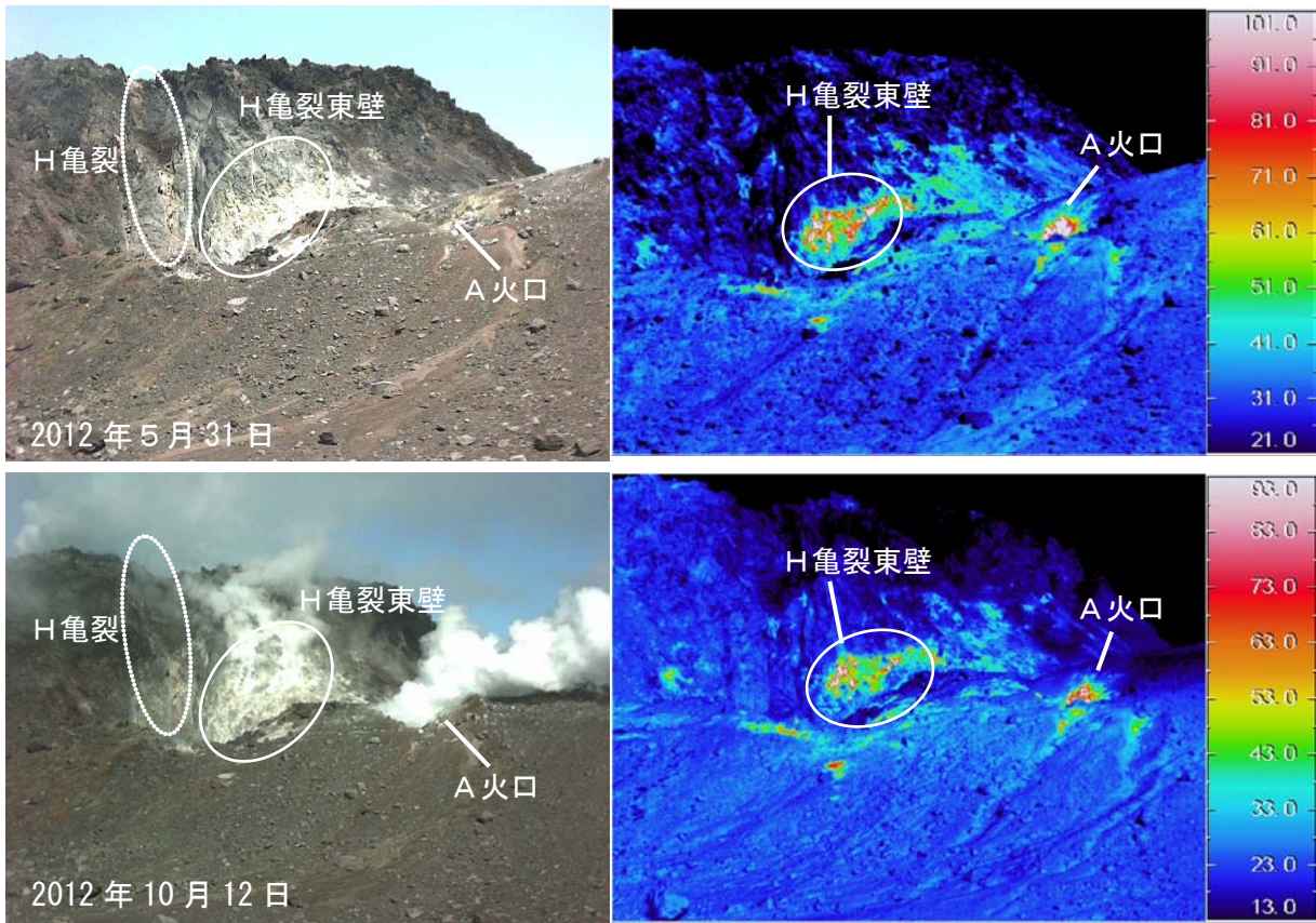
図 4 樽前山 赤外熱映像装置 1) によるA火口、H亀裂及びそれら周辺の地表面温度分布 (図3-①より撮影)
