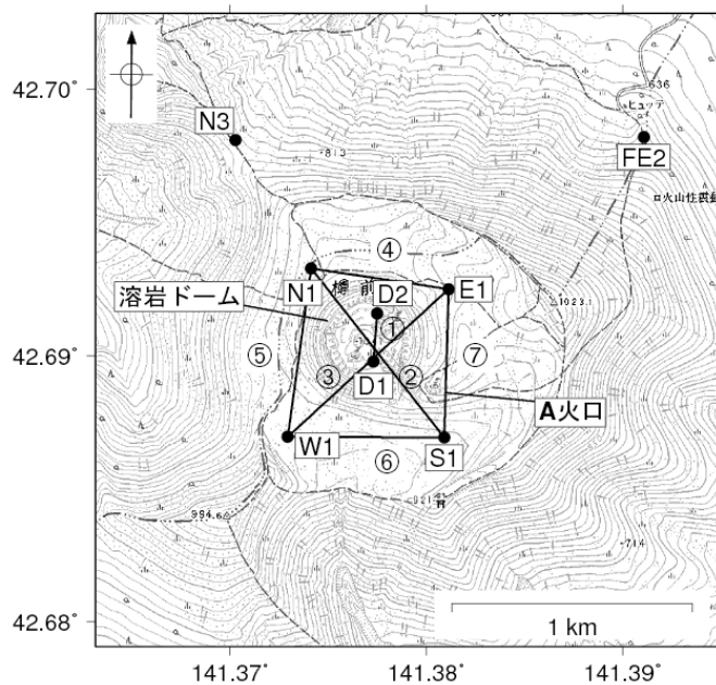
図8 樽前山 GPS 繰り返し観測点配置図
