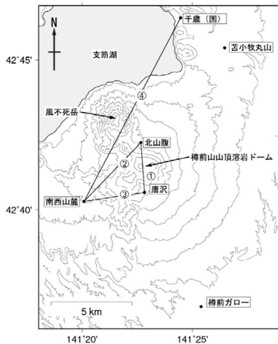
図10 樽前山 GPS連続観測点配置図 (国)：国土地理院
