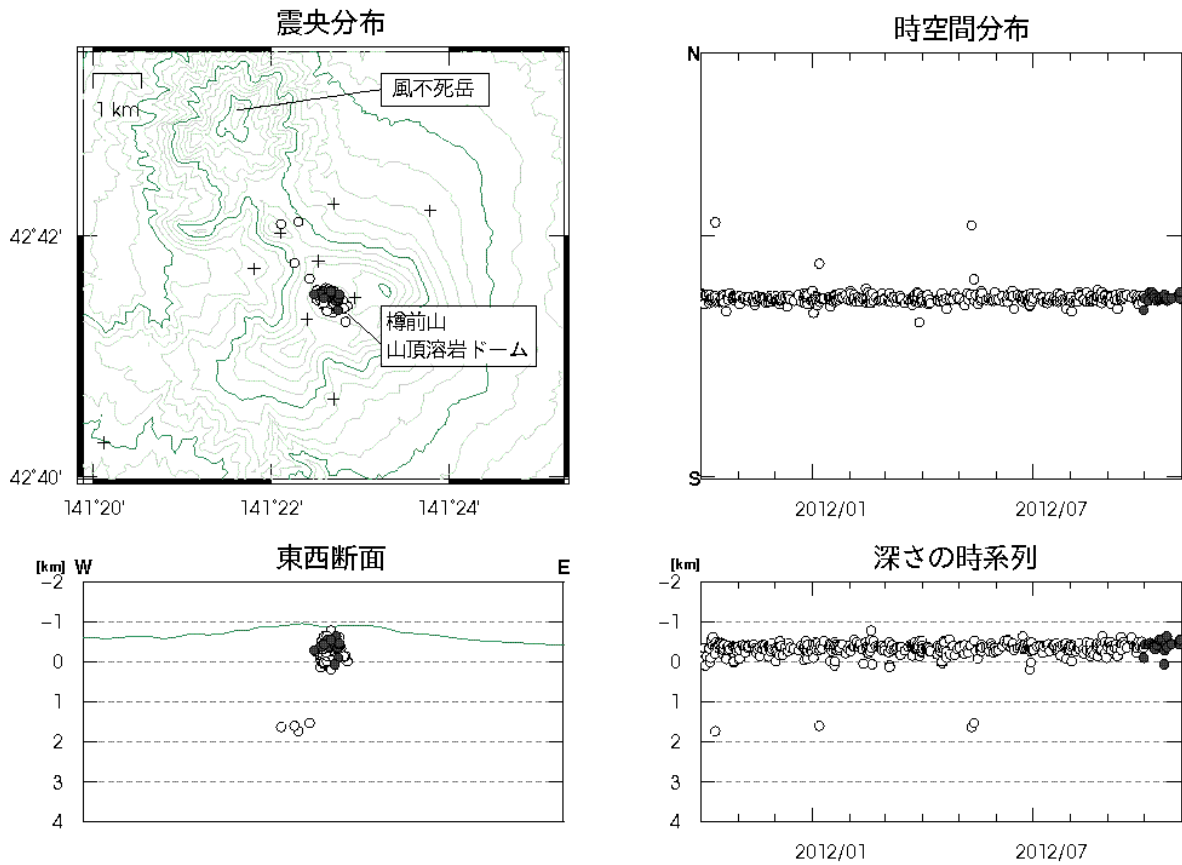
図 6※ 樽前山 火山性地震の震源分布 (2011年10月～2012年10月) ○印：2011年10月～2012年9月の震源 ●印：2012年10月の震源 +印：地震観測点
