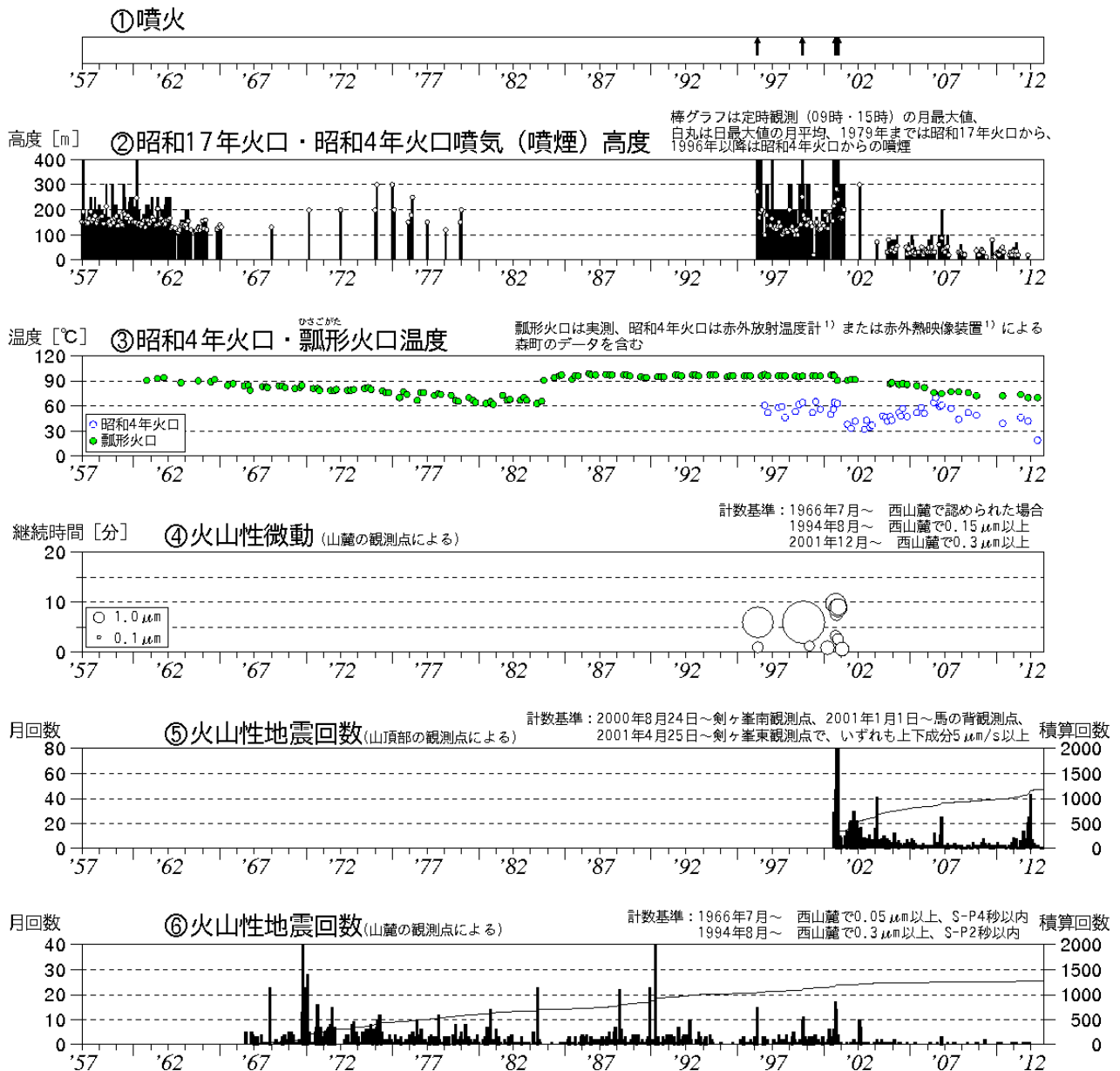
図 1※ 北海道駒ヶ岳 火山活動経過図（1957年 1 月～2012年 9 月）
