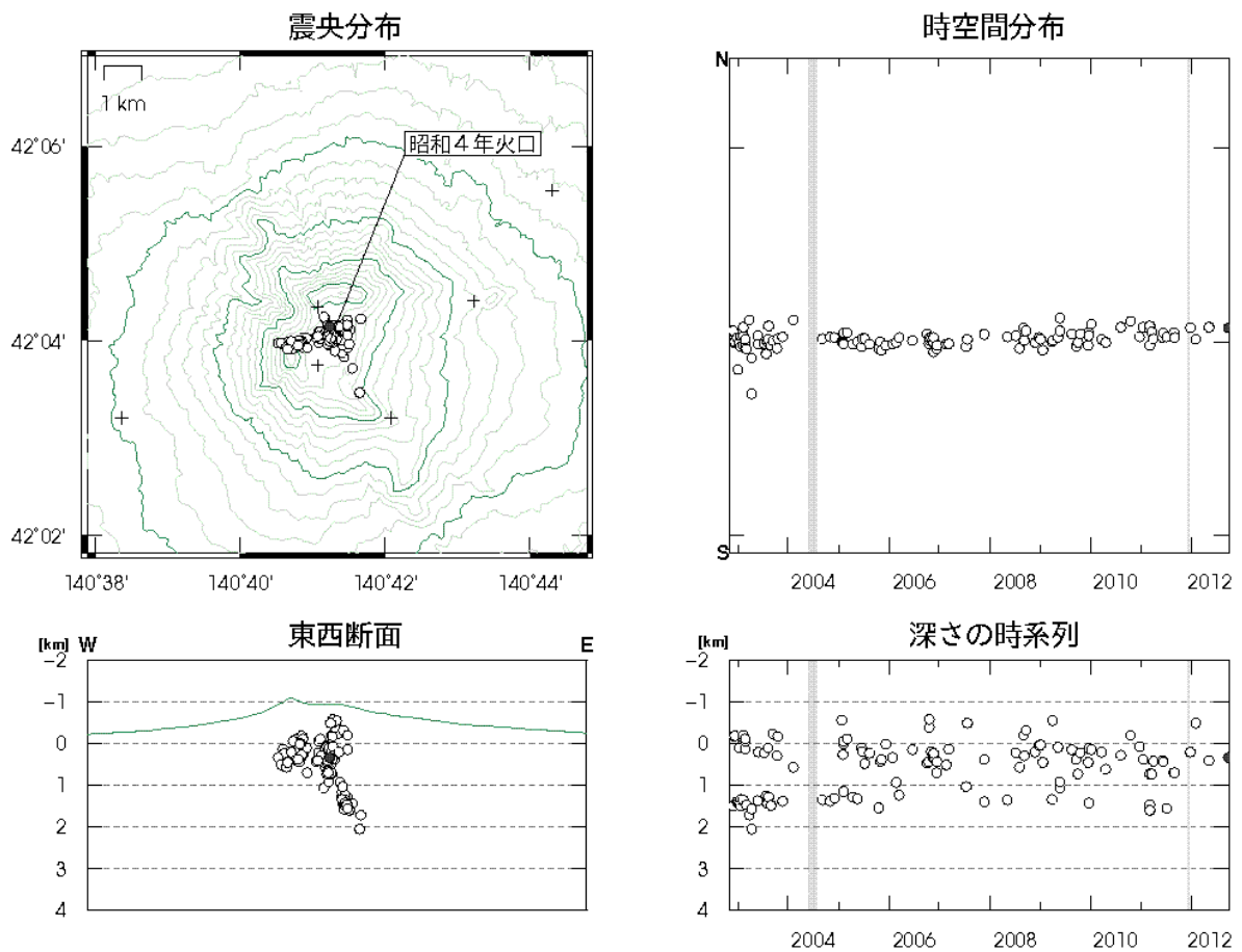
図3※ 北海道駒ヶ岳 火山性地震の震源分布（2002年12月～2012年9月） 灰色の期間は一部観測点欠測のため震源の決定数減少や精度低下が見られます ○印：2002年11月から2012年8月の震源 ●印：2012年9月の震源 +印：地震観測点
