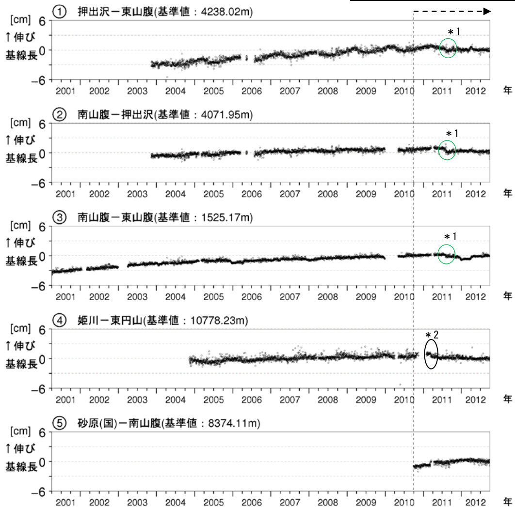
図 4 ※ 北海道駒ヶ岳 GPS連続観測による基線長変化 (2001年 4 月～2012年 9 月)
