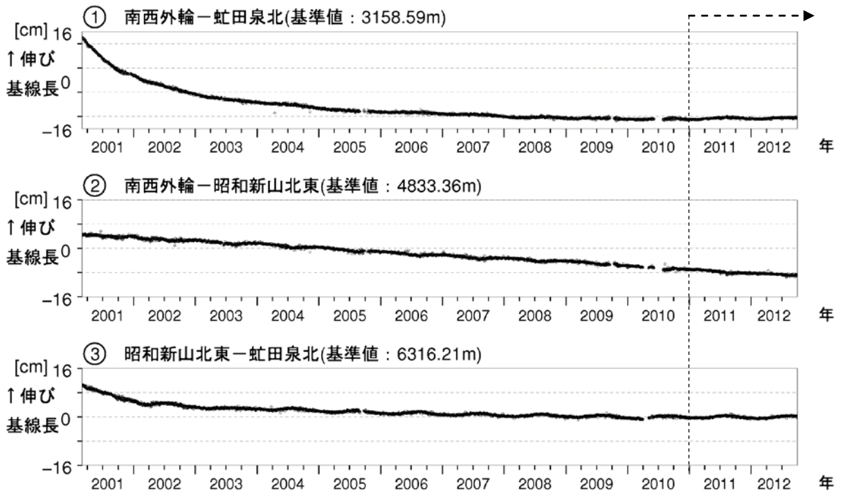
図 4 有珠山 GPS連続観測による基線長変化 (2001年3月~2012年9月)
