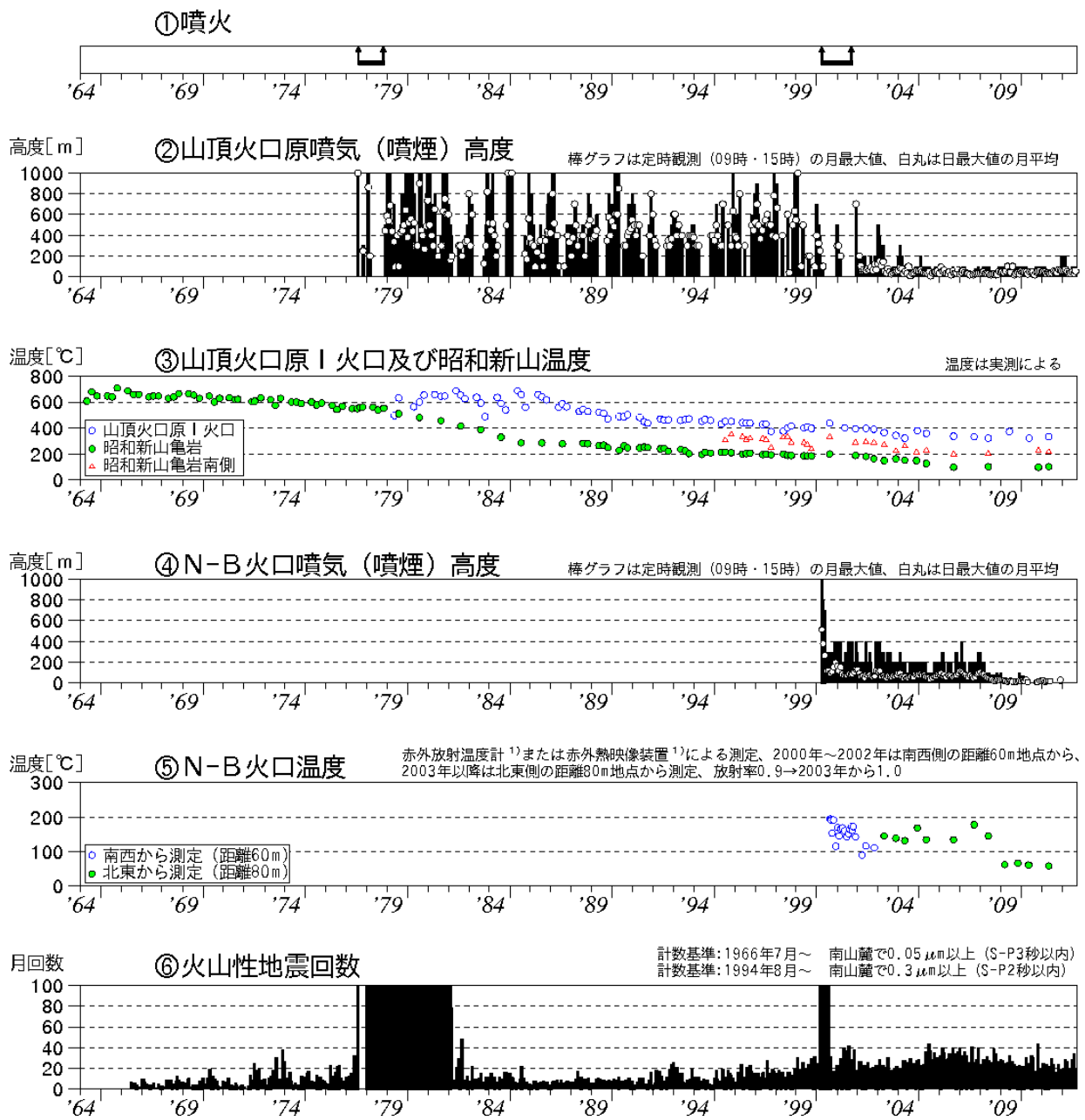
図 1※ 有珠山 火山活動経過図（1964年 1 月～2012年 9 月）
