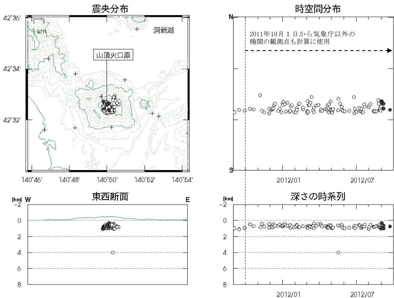
図 3※ 有珠山 火山性地震の震源分布（2011年9月～2012年9月）
