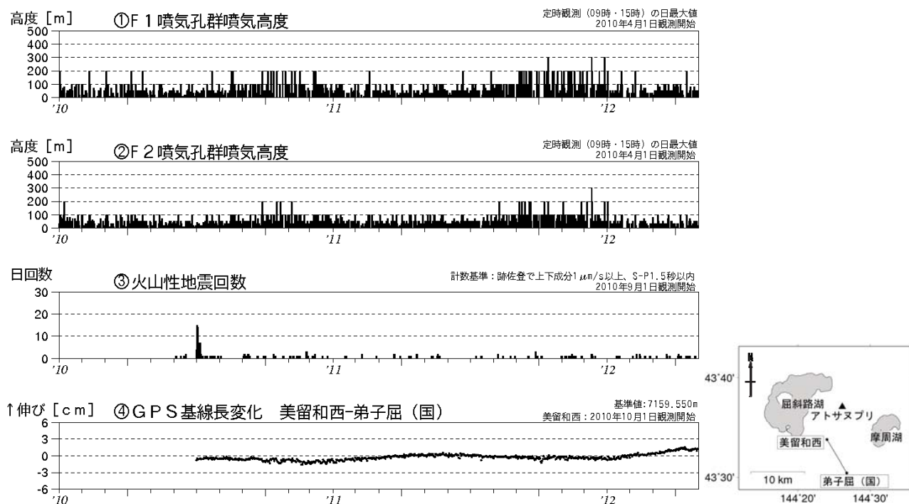
図 2※ アトサヌプリ 火山活動経過図 (2010年 4 月～2012年 7 月)、GPS連続観測点配置図 ・④のGPS基線は右図に対応しています ・(国)：国土地理院
