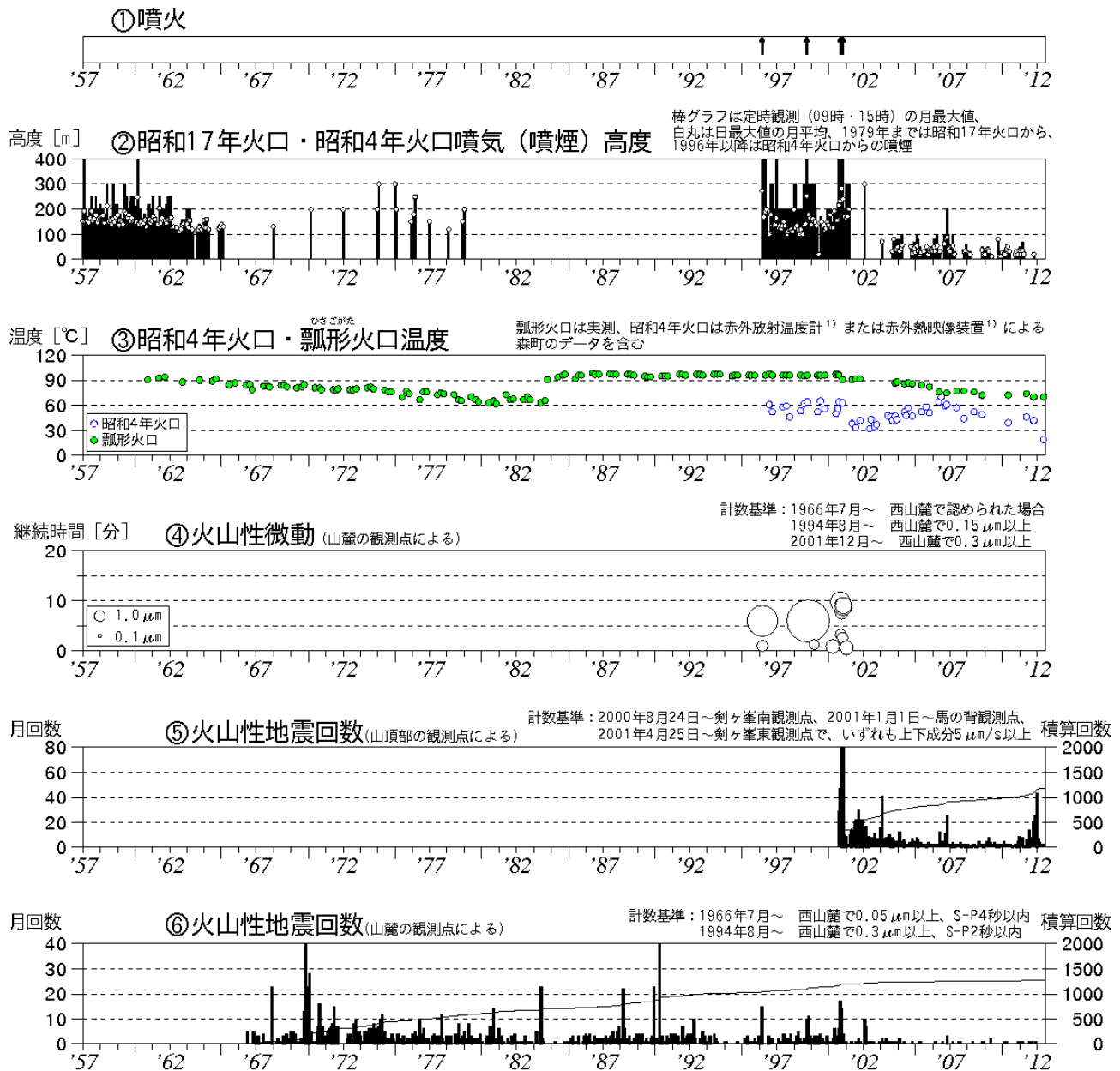
図 1※ 北海道駒ヶ岳 火山活動経過図（1957年 1 月～2012年 6 月）
