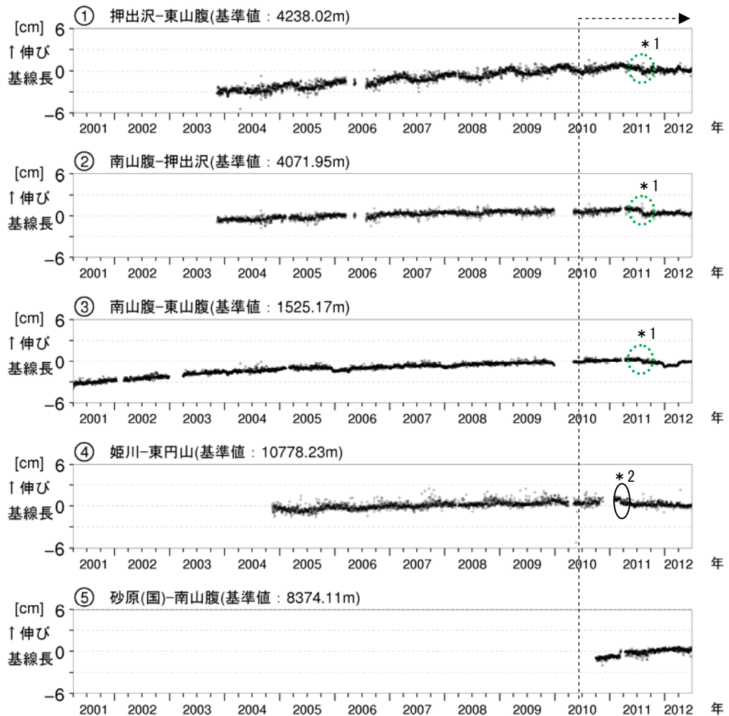
図 4 ※ 北海道駒ヶ岳 GPS連続観測による基線長変化（2001年 4 月～2012年 6 月）
