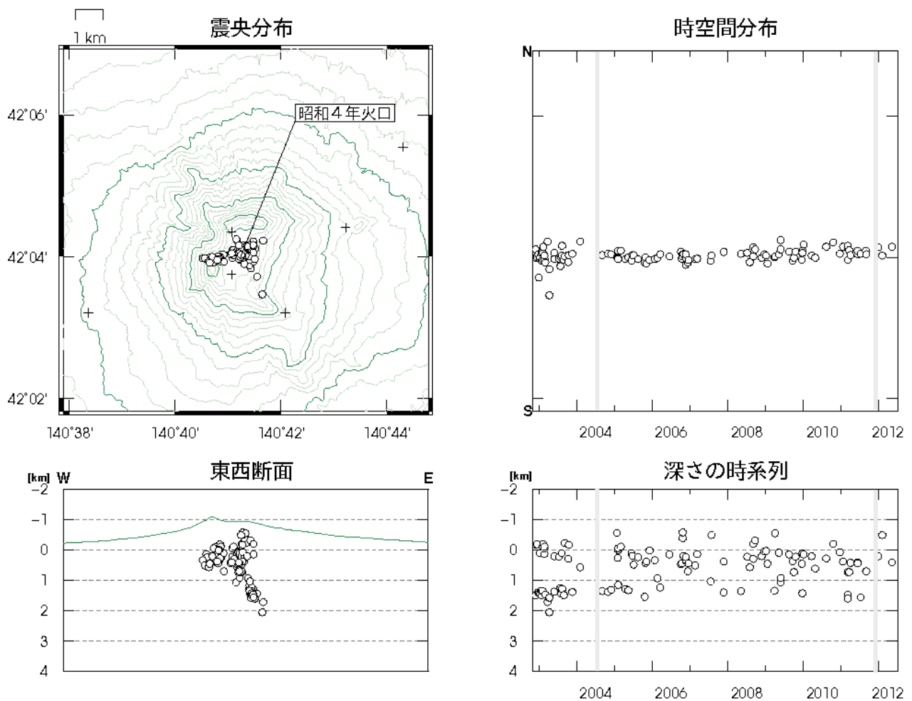
図3※ 北海道駒ヶ岳 火山性地震の震源分布（2002年12月～2012年6月） 灰色の期間は一部観測点欠測のため震源の決定数減少や精度低下が見られます ○印：2002年11月から2012年5月の震源 +印：地震観測点
