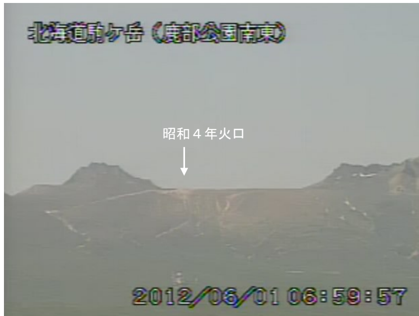
図2 北海道駒ヶ岳 山頂部の状況（6月1日、鹿部公園南東遠望カメラによる）
