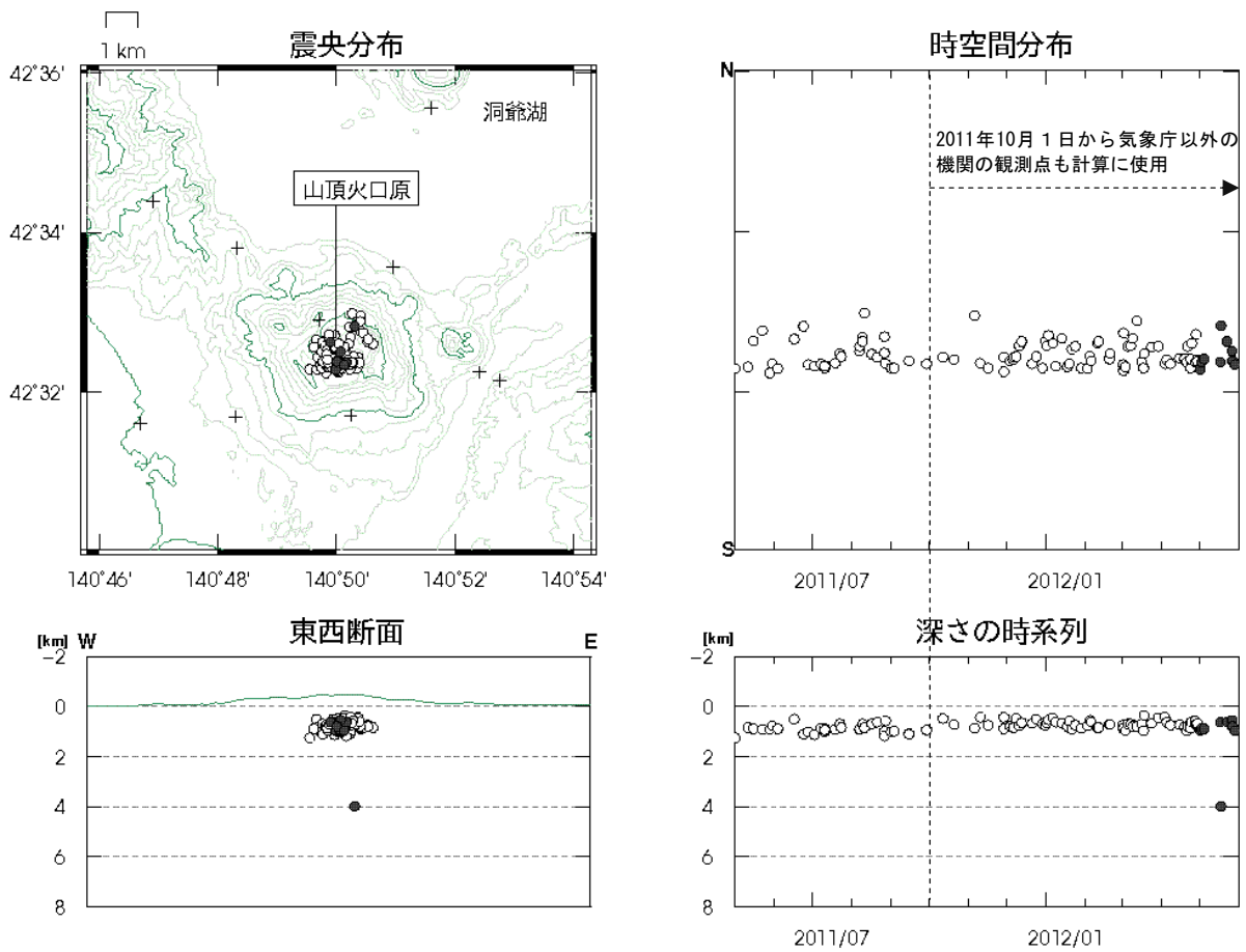
図3※ 有珠山 火山性地震の震源分布（2011年5月～2012年5月）
