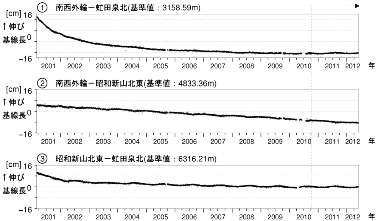
図 4 有珠山 GPS連続観測による基線長変化 (2001年3月~2012年5月) ・グラフの空白部分は欠測 GPS基線①~③は図5の①~③に対応 ・2010年10月以降のデータについては、電離層の影響を補正する等、解析方法を改良しています
