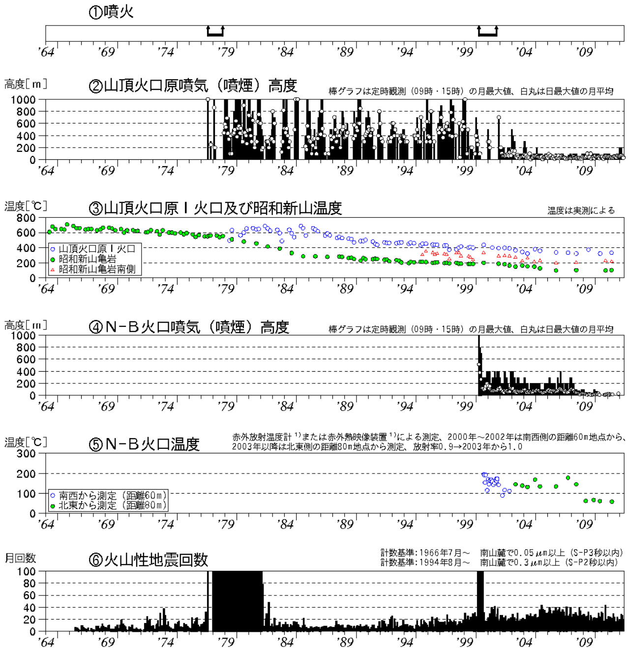
図 1※ 有珠山 火山活動経過図（1964年 1 月～2012年 5 月）
