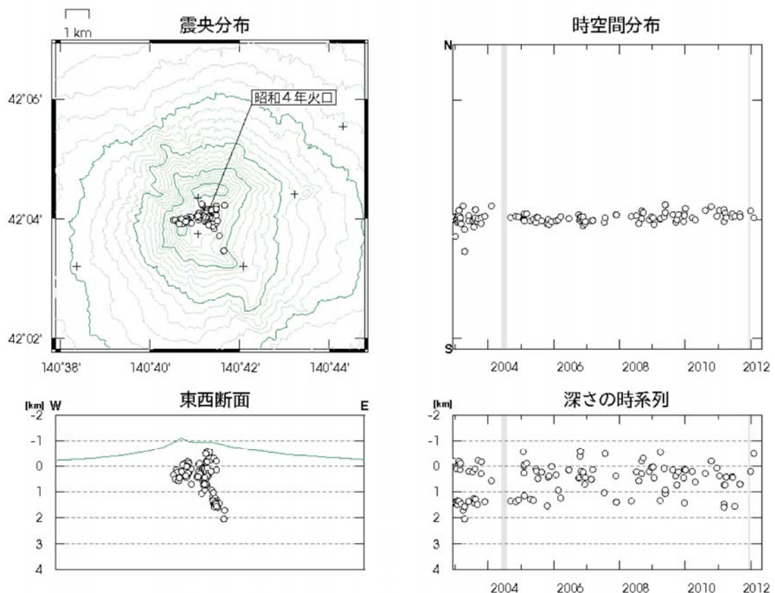
図 3※ 北海道駒ヶ岳 火山性地震の震源分布（2002年12月～2012年4月） 灰色の期間は一部観測点欠測のため震源の決定数減少や精度低下が見られます ○印：2002年11月から2012年3月の震源 +印：地震観測点
