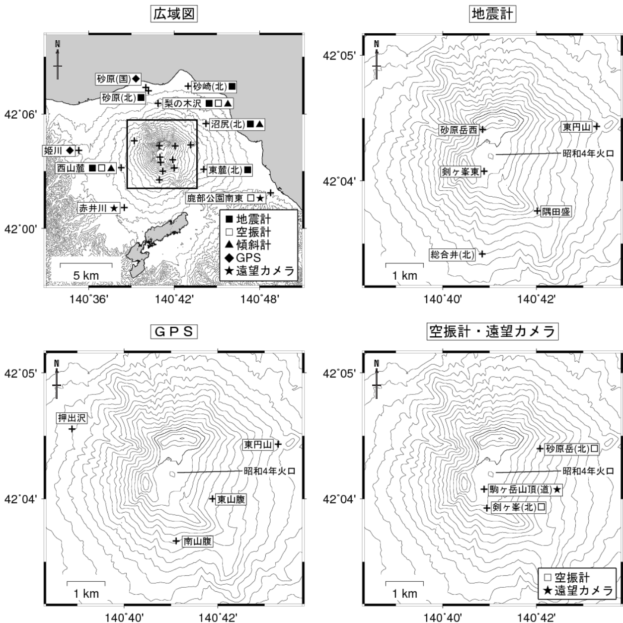
図 6 北海道駒ヶ岳 観測点配置図 広域図内の口は地震計、GPS・傾斜計、空振計・遠望カメラそれぞれの範囲を示します +は観測点の位置を示します 気象庁以外の機関の観測点には以下の記号を付しています (国)：国土地理院 (北)：北海道大学 (道)：北海道
