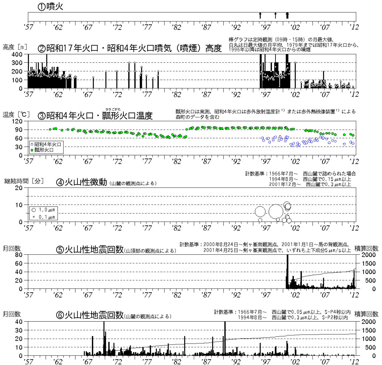
図 1 ※ 北海道駒ヶ岳 火山活動経過図（1957年 1 月～2012年 4 月）
