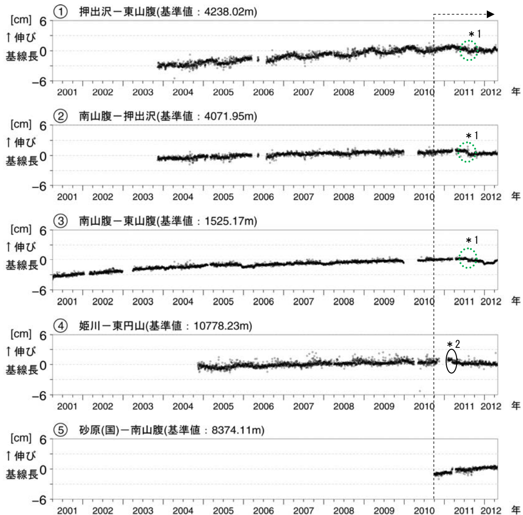
図 4 ※ 北海道駒ヶ岳 GPS連続観測による基線長変化（2001年 4 月～2012年 4 月）
