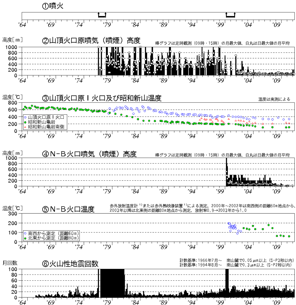
図 1 有珠山 火山活動経過図（1964年 1 月～2012年 4 月）
