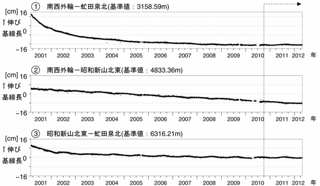
図4 有珠山 GPS連続観測による基線長変化(2001年3月~2012年4月) ・グラフの空白部分は欠測 GPS基線 ~ は図5の ~ に対応 ・2010年10月以降のデータについては、電離層の影響を補正する等、解析方法を改良しています
