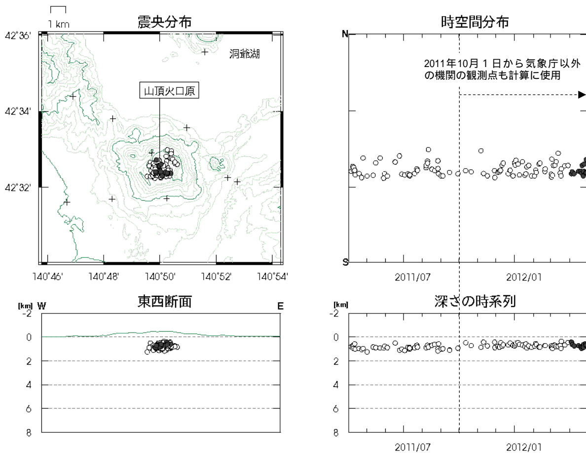
図 3 有珠山 火山性地震の震源分布（2011年4月～2012年4月）
