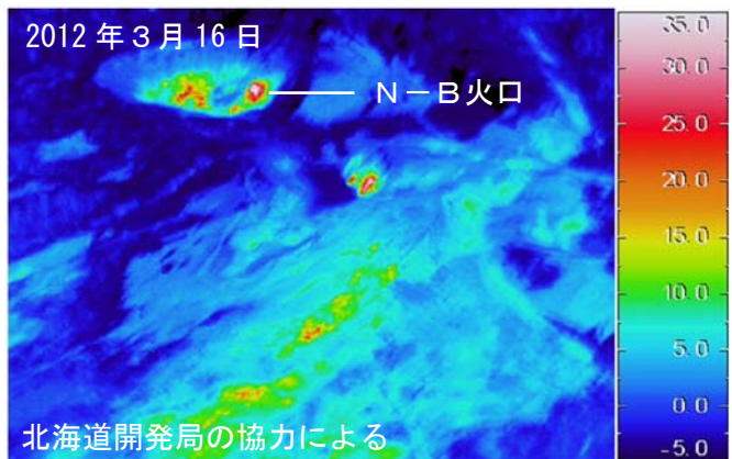
図5 有珠山 赤外熱映像装置 1) によるN-B火口の地表面温度分布 北側上空 (図2の③矢印方向) から撮影
