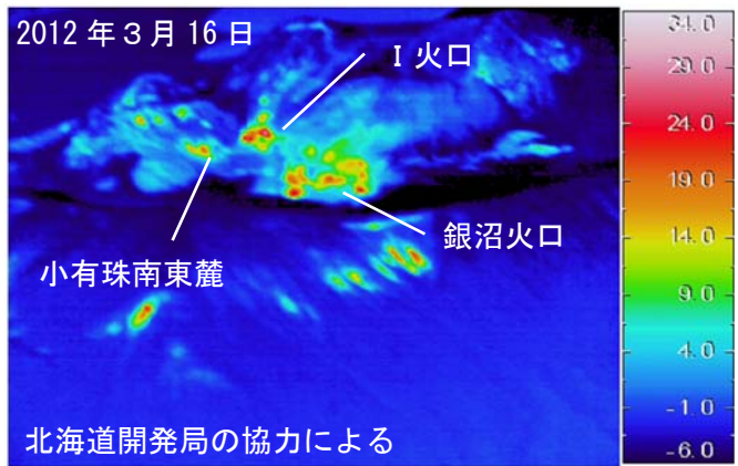
図4 有珠山 赤外熱映像装置 1) による山頂火口原の地表面温度分布 南側上空 (図2の②矢印方向) から撮影
