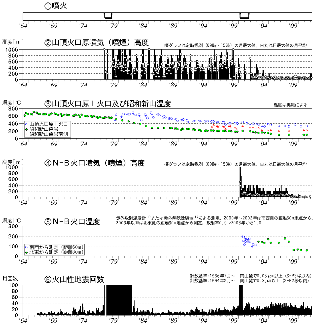
図 1※ 有珠山 火山活動経過図（1964年 1 月～2012年 3 月）
