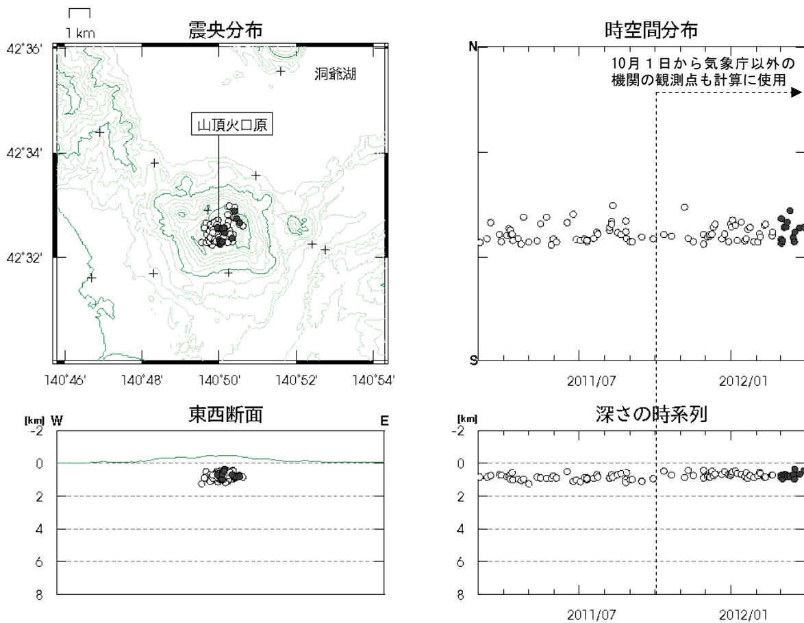
図 7※ 有珠山 火山性地震の震源分布（2011年3月～2012年3月）
