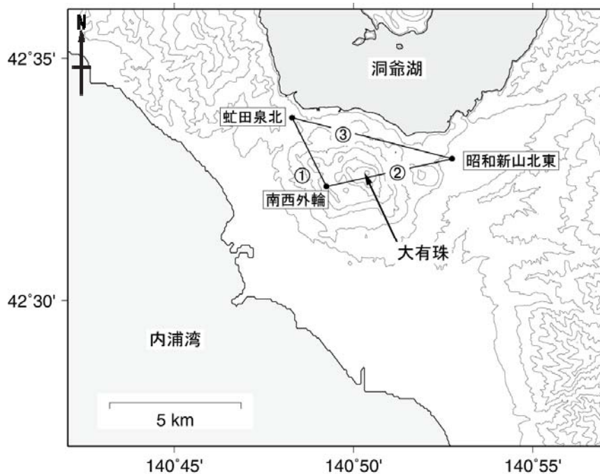
図 9 有珠山 GPS連続観測点配置図
