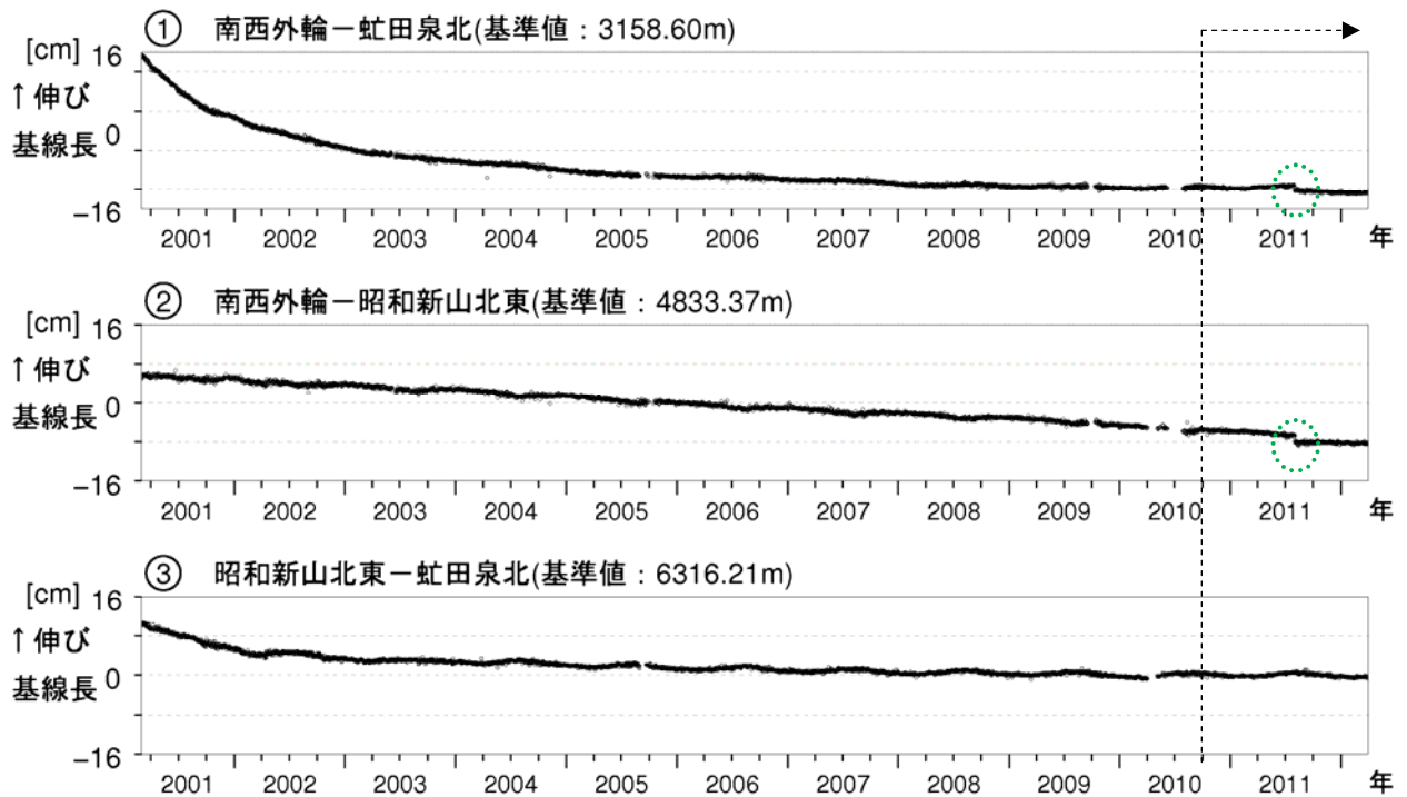
図 8 有珠山 GPS連続観測による基線長変化 (2001年3月～2012年3月)
