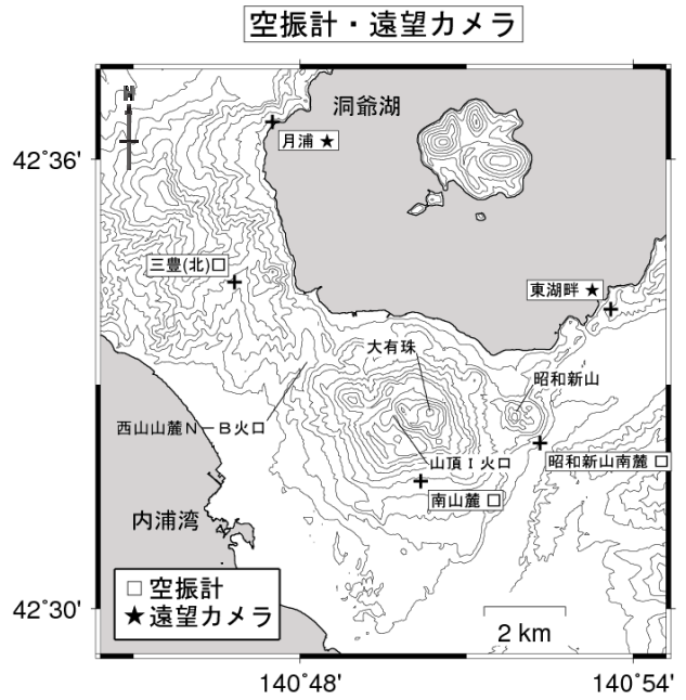
図10 有珠山 観測点配置図 +は観測点の位置を示します 気象庁以外の機関の観測点には以下の記号を付しています (北) : 北海道大学 (防) : 防災科学技術研究所
