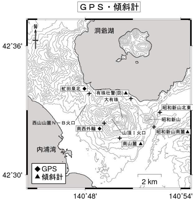
図10 有珠山 観測点配置図 +は観測点の位置を示します 気象庁以外の機関の観測点には以下の記号を付しています (北) : 北海道大学 (防) : 防災科学技術研究所
