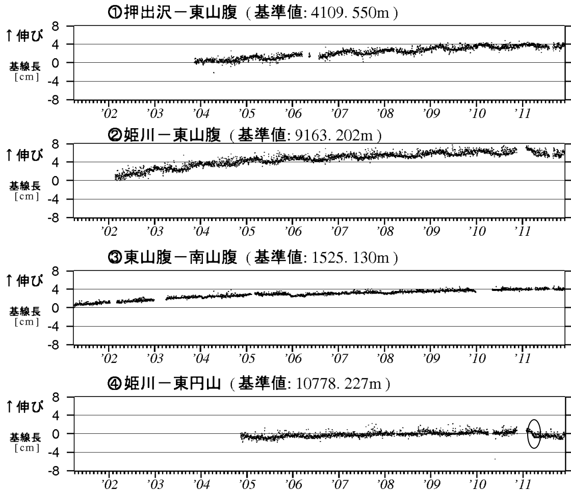
図4 北海道駒ヶ岳 GPS 連続観測による基線長変化（2001 年 4 月～2011 年 11 月） ・グラフの空白部分は欠測 ・楕円内の変動は、2011 年 3 月 11 日に発生した東北地方太平洋沖地震の影響による。 ・GPS 基線①～④は図5 ①～④に対応
