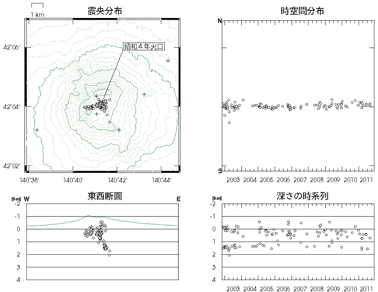
図 3※ 北海道駒ヶ岳 火山性地震の震源分布（2002 年 11 月～2011 年 11 月）
