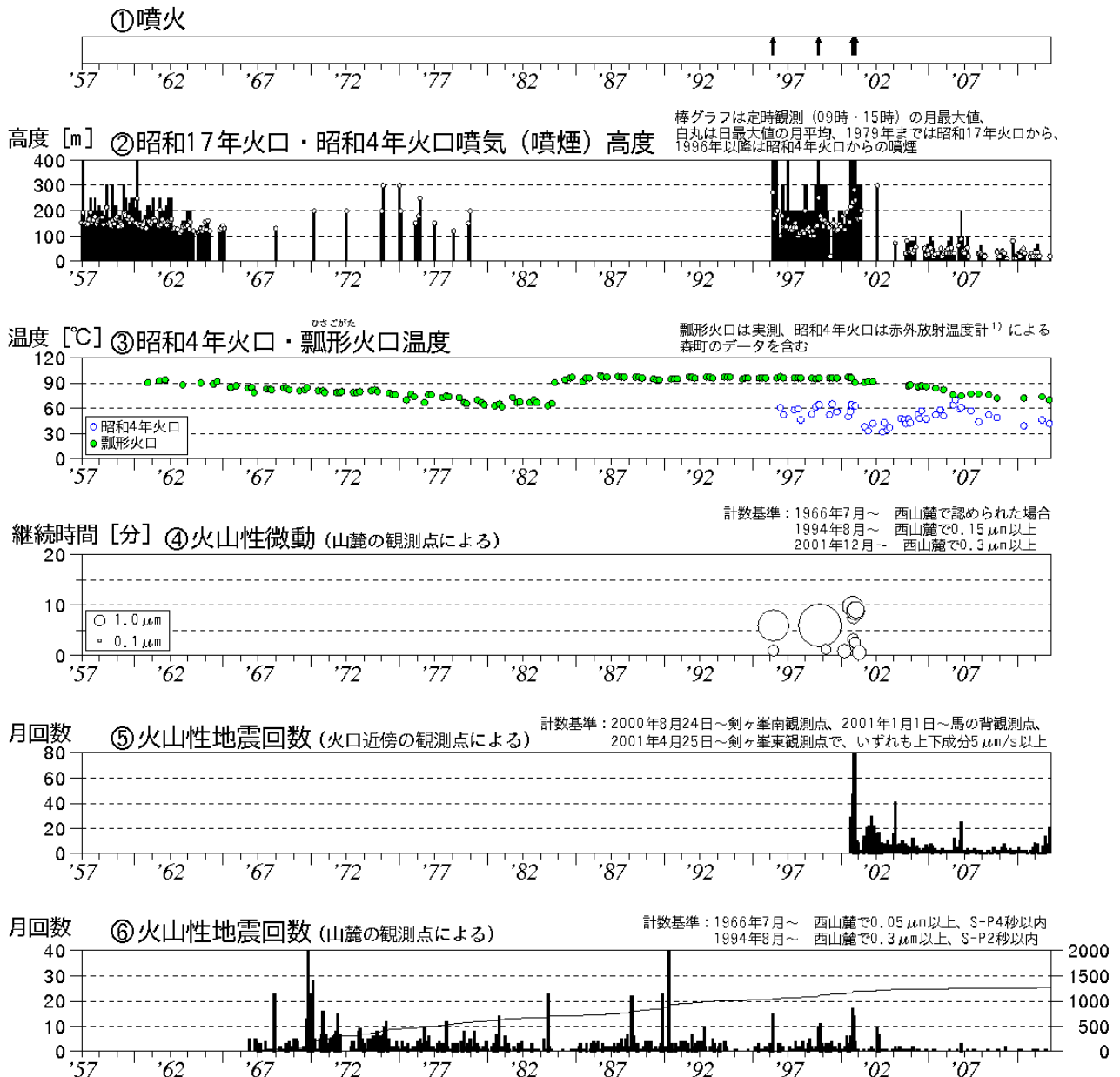
図 1 ※ 北海道駒ヶ岳 火山活動経過図（1957 年 1 月～2011 年 11 月）
