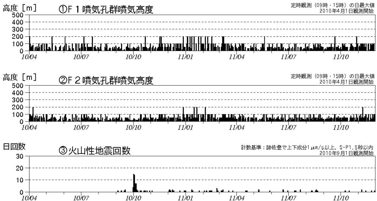
図 1 アトサヌプリ 火山活動経過図（2010年4月～2011年11月）
