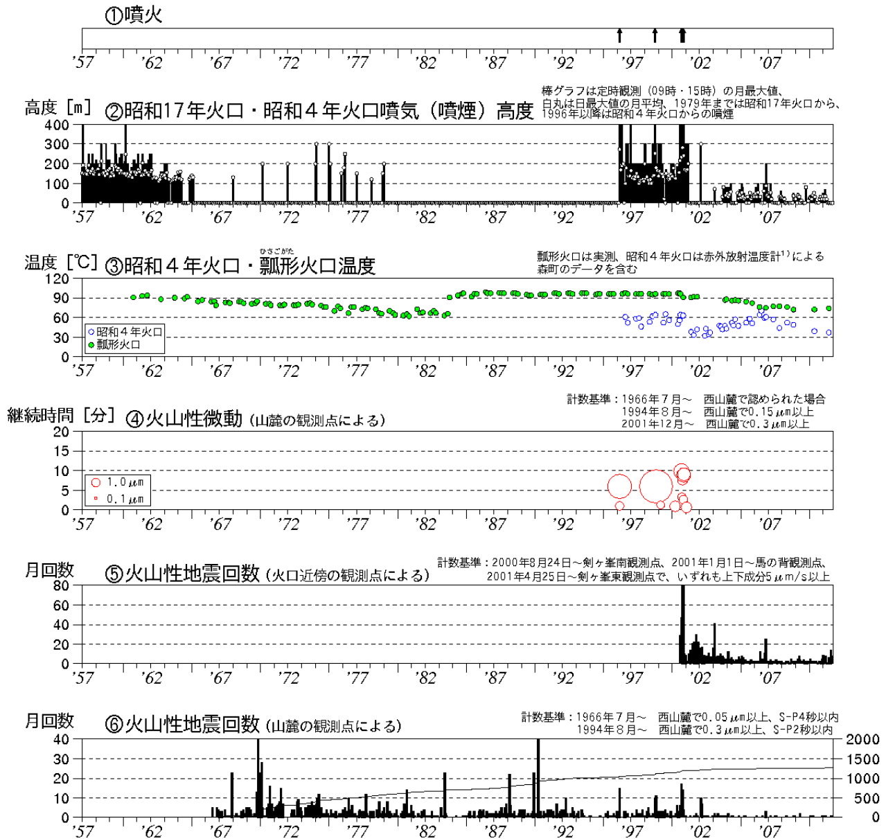
図 1 ※ 北海道駒ヶ岳 火山活動経過図（1957 年 1 月～2011 年 9 月）
