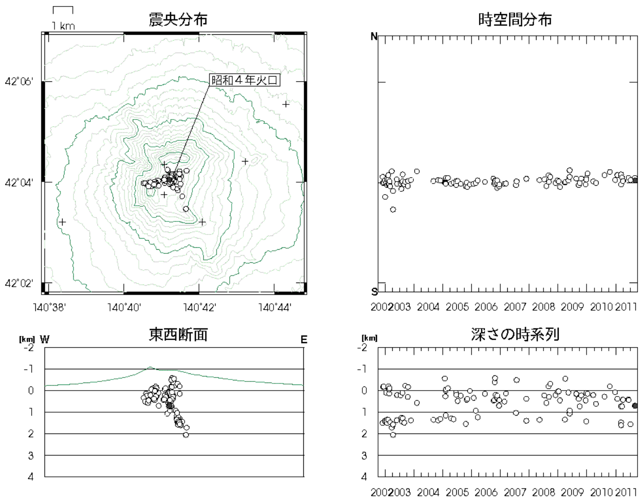
図 3※ 北海道駒ヶ岳 火山性地震の震源分布(2002 年 11 月～2011 年 9 月)
