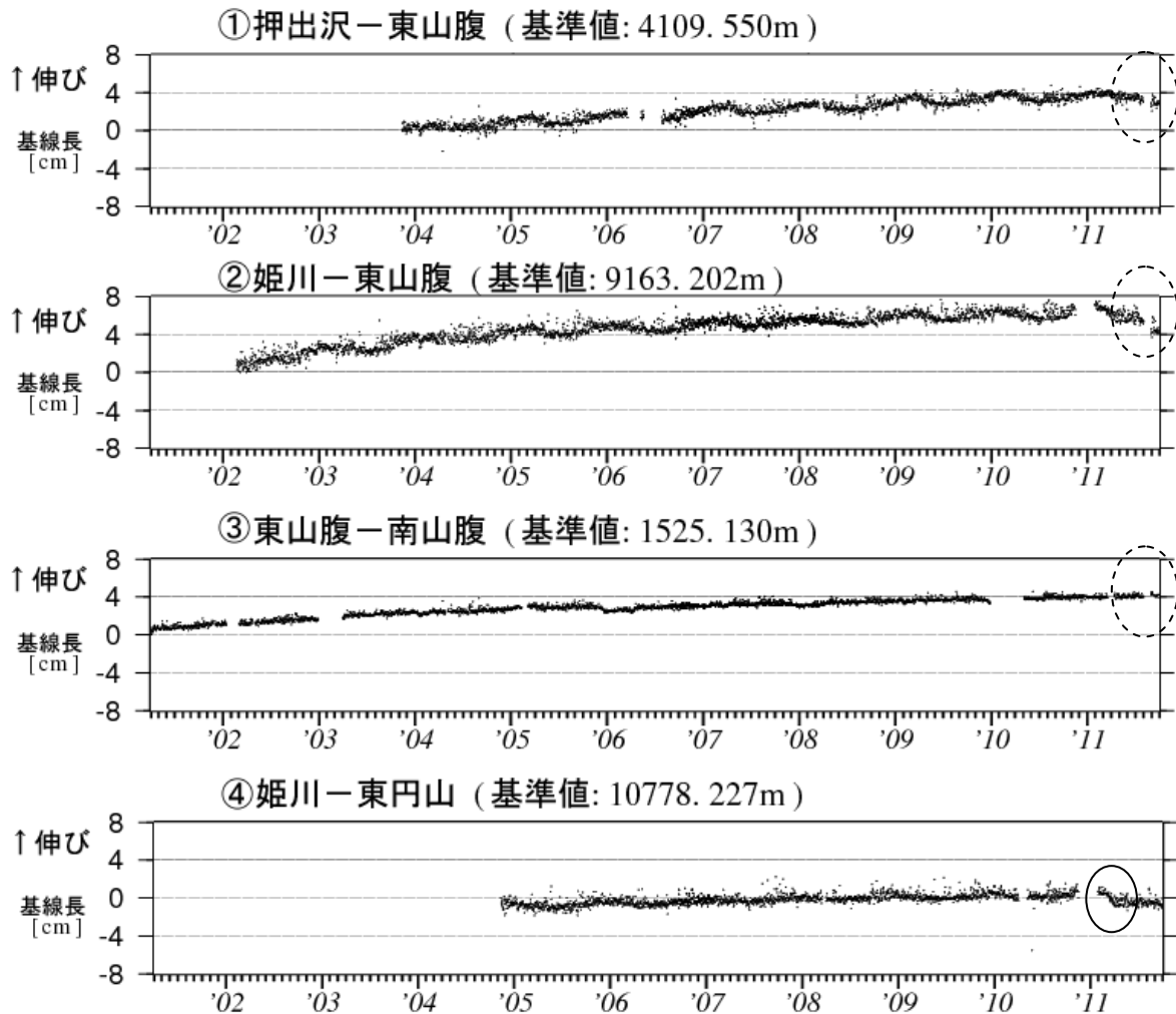
図4 北海道駒ヶ岳 GPS 連続観測による基線長変化（2001 年 4 月～2011 年 9 月） グラフの空白部分は欠測 破線楕円内の変動及び欠測は観測機器更新（2011 年 8 月 1～30 日）による。 実線楕円内の変動は東北地方太平洋沖地震（2011 年 3 月 11 日）による。 GPS 基線①～④は図 5 ①～④に対応
