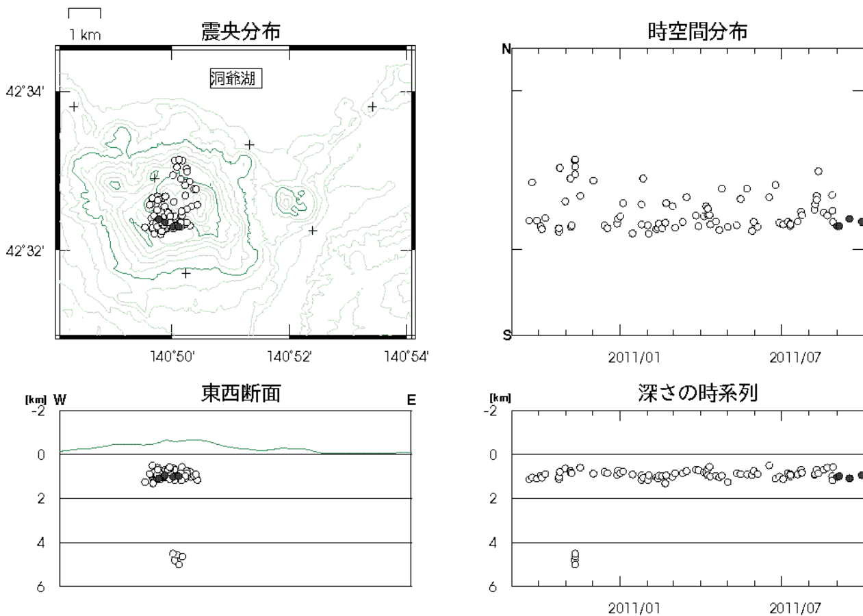
図 3 有珠山 火山性地震の震源分布（2010年8月～2011年9月）
