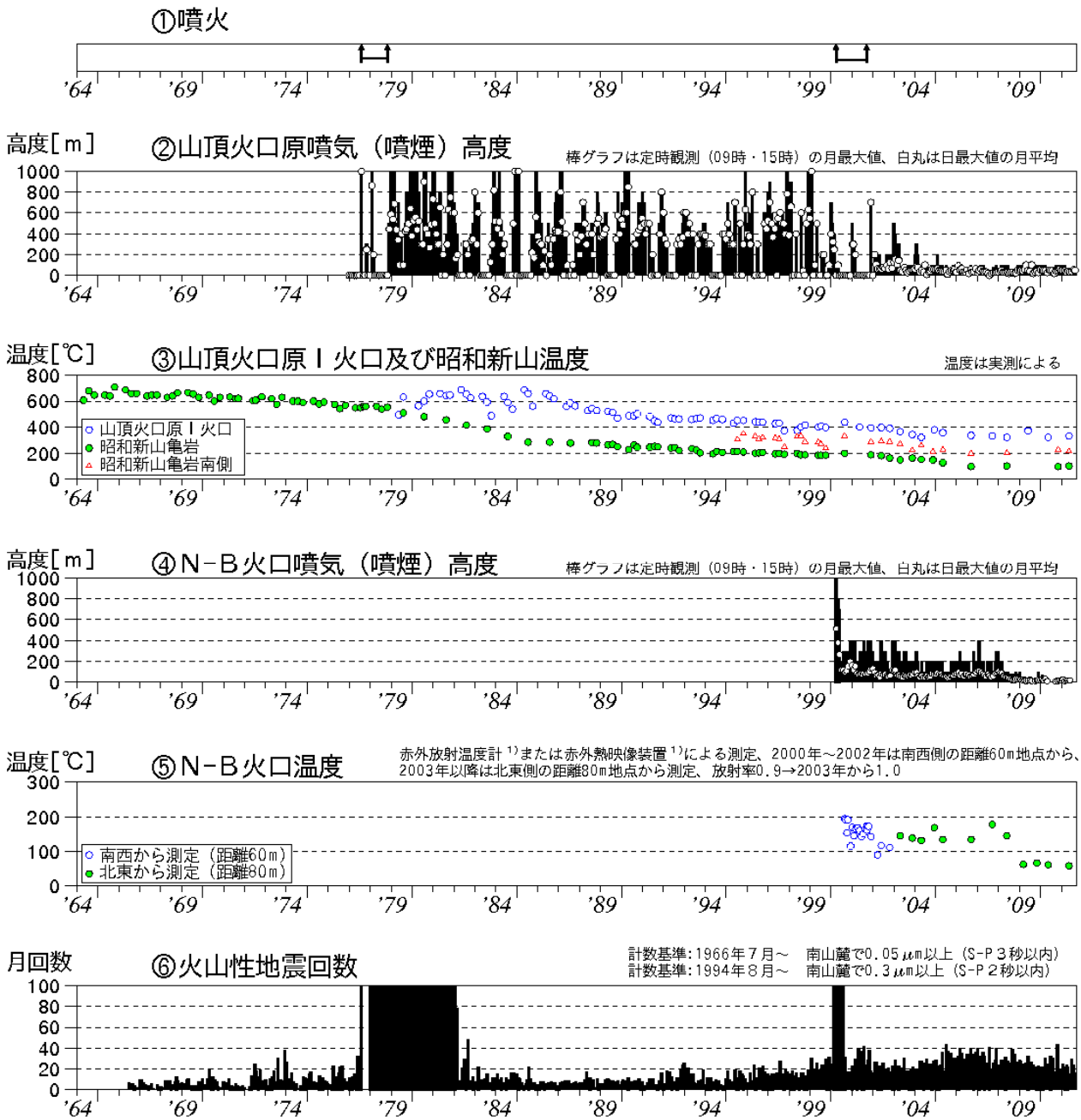
図1 有珠山 火山活動経過図（1964年1月～2011年9月）
