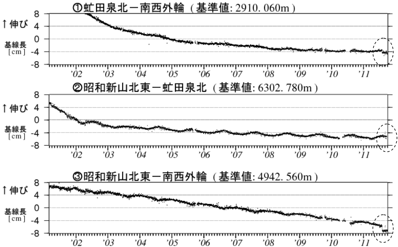
図 4 有珠山 GPS 連続観測による基線長変化（2001 年 3 月～2011 年 9 月） グラフの空白部分は欠測 破線楕円内の変動は観測機器更新（2011 年 8 月 1 日）による。 GPS 基線①～③は図 5 ①～③に対応
