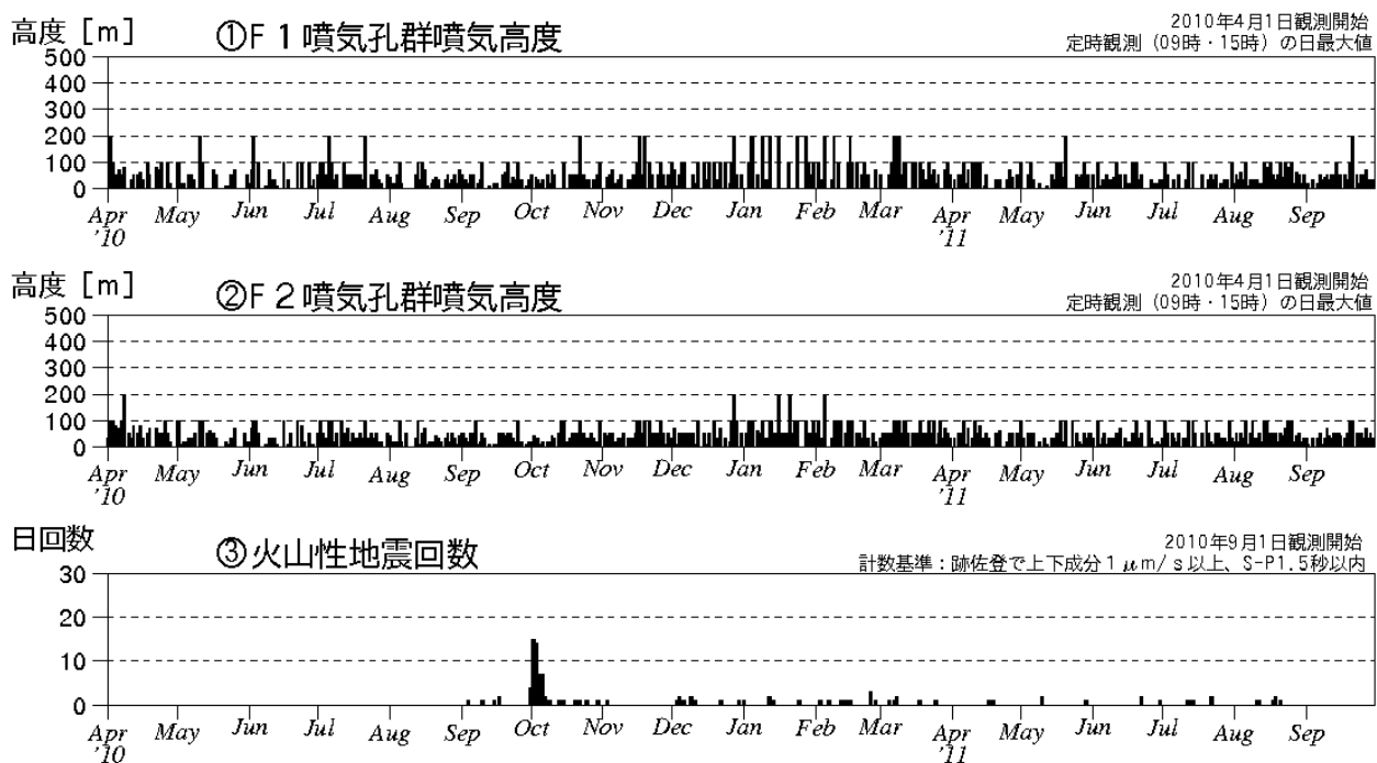
図 1 アトサヌプリ 火山活動経過図（2010 年 4 月～2011 年 9 月）
