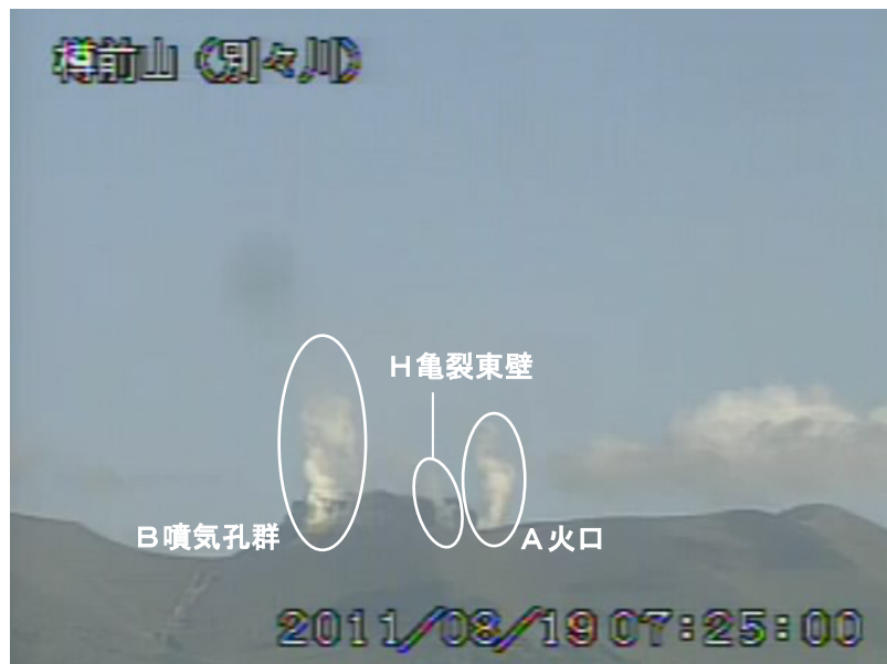
図5 樽前山 山頂溶岩ドーム付近の状況 (8月19日、別々川遠望カメラによる) 白丸内はA火口、B噴気孔群、H亀裂東壁の噴気
