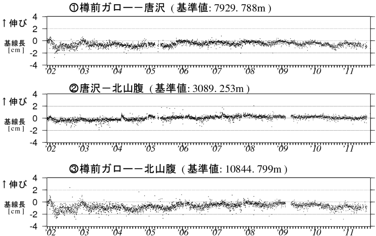
図7 樽前山 GPS 連続観測による基線長変化 (2001 年 12 月~2011 年 8 月) グラフの空白部分は欠測 GPS 基線①~③は、図8の①~③に対応しています。
