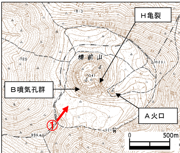
図2 樽前山 火口周辺図 (①は赤外熱映像の撮影位置)
