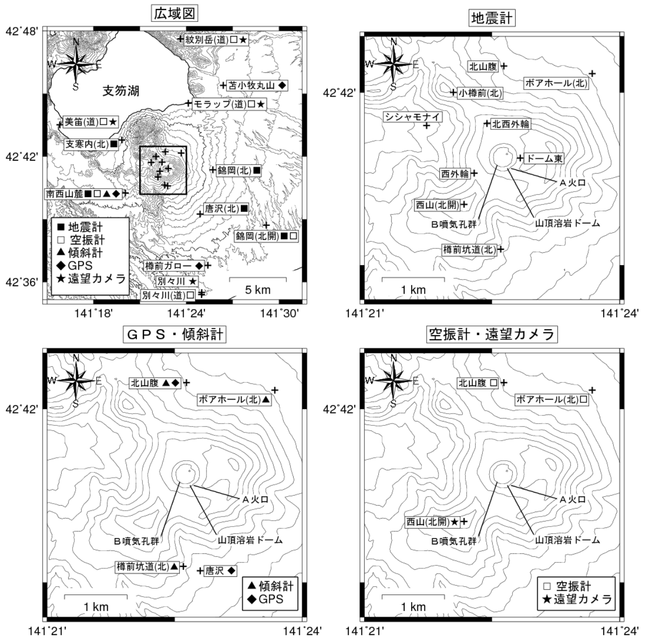
図9 樽前山 観測点配置図 +は観測点の位置を示す 他機関の観測点には以下の記号を付している (北) : 北海道大学 (北開) : 北海道開発局 (道) : 北海道
