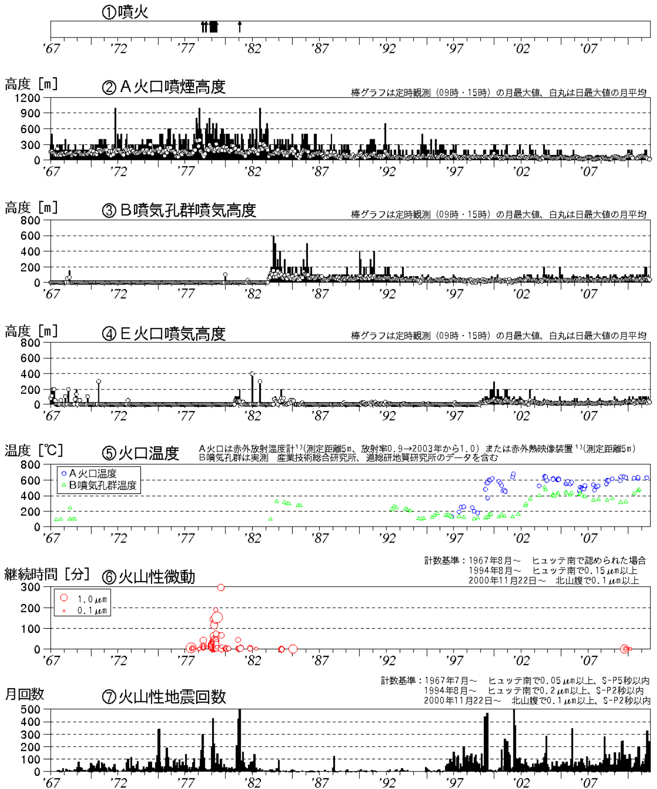
図 1 ※ 樽前山 火山活動経過図 (1967 年 1 月～2011 年 8 月)
