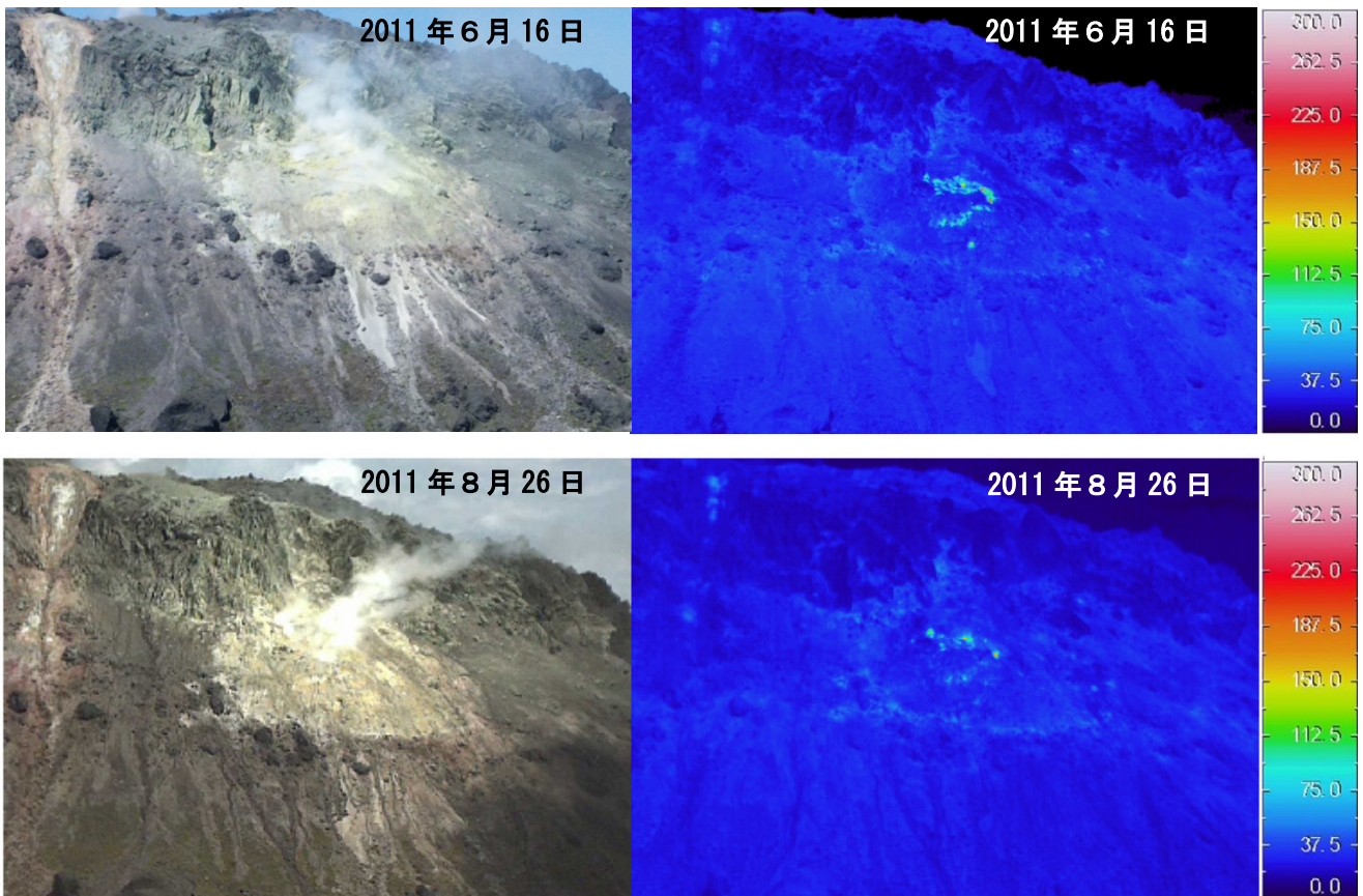
図4 樽前山 赤外熱映像装置 1) によるB噴気孔群の地表面温度分布 (図2の①より撮影)
