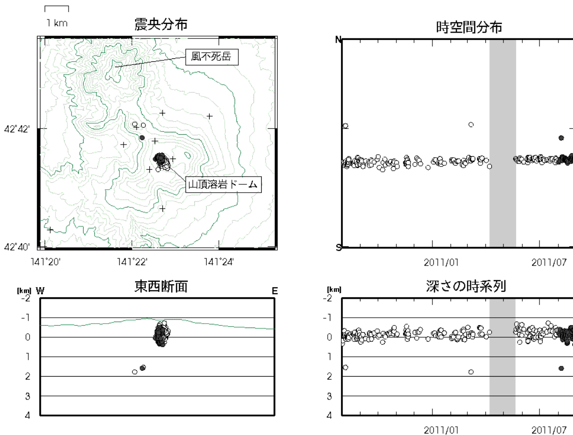
図6※ 樽前山 火山性地震の震源分布 (2010年8月~2011年8月) 表示期間中、灰色の期間は一部観測点欠測のため震源の決定数減少や精度低下が見られます ○印：2010年8月~2011年7月の震源 ●印：2011年8月の震源 +印：地震観測点
