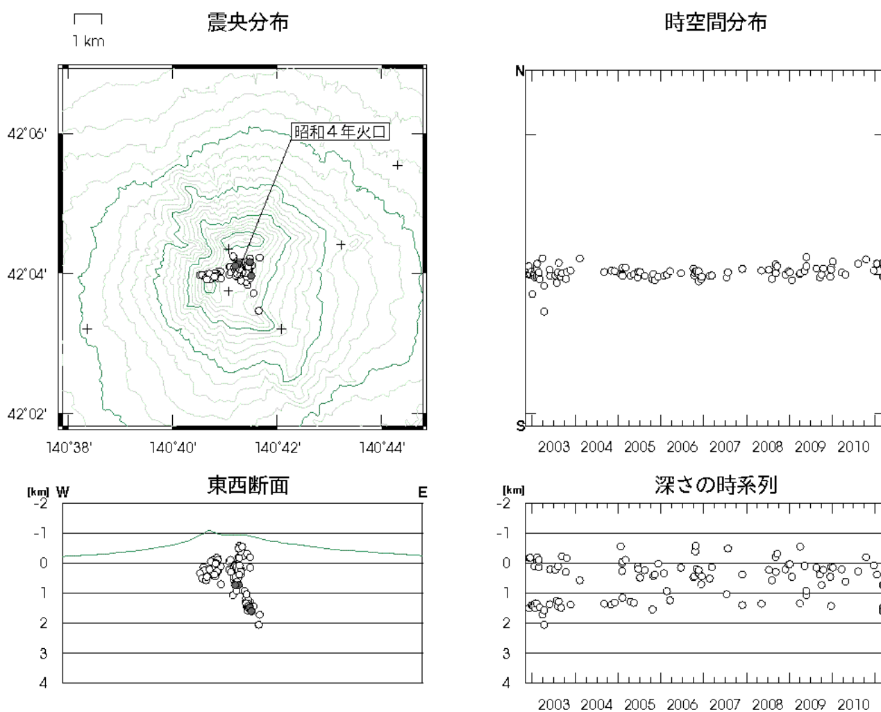
図 3※ 北海道駒ヶ岳 震源分布図（2002 年 11 月～2011 年 3 月、+は地震観測点）
