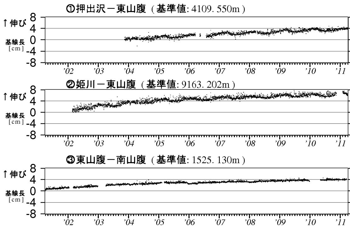
図 4 北海道駒ヶ岳 GPS 連続観測による基線長変化（2001 年 4 月～2011 年 3 月） グラフの空白部分は欠測 図 4 の①～③は、図 5 の GPS 基線①～③に対応しています。 姫川観測点は 2010 年 10 月 29 日に機器の更新を行いました。
