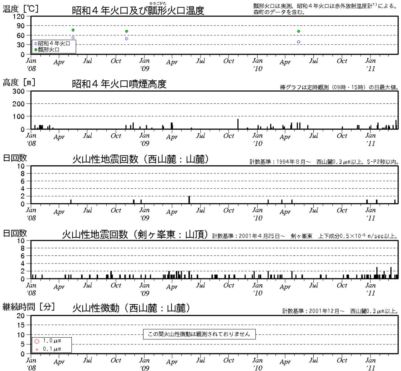
図2※ 北海道駒ヶ岳 最近の火山活動経過図（2008年1月～2011年3月）
