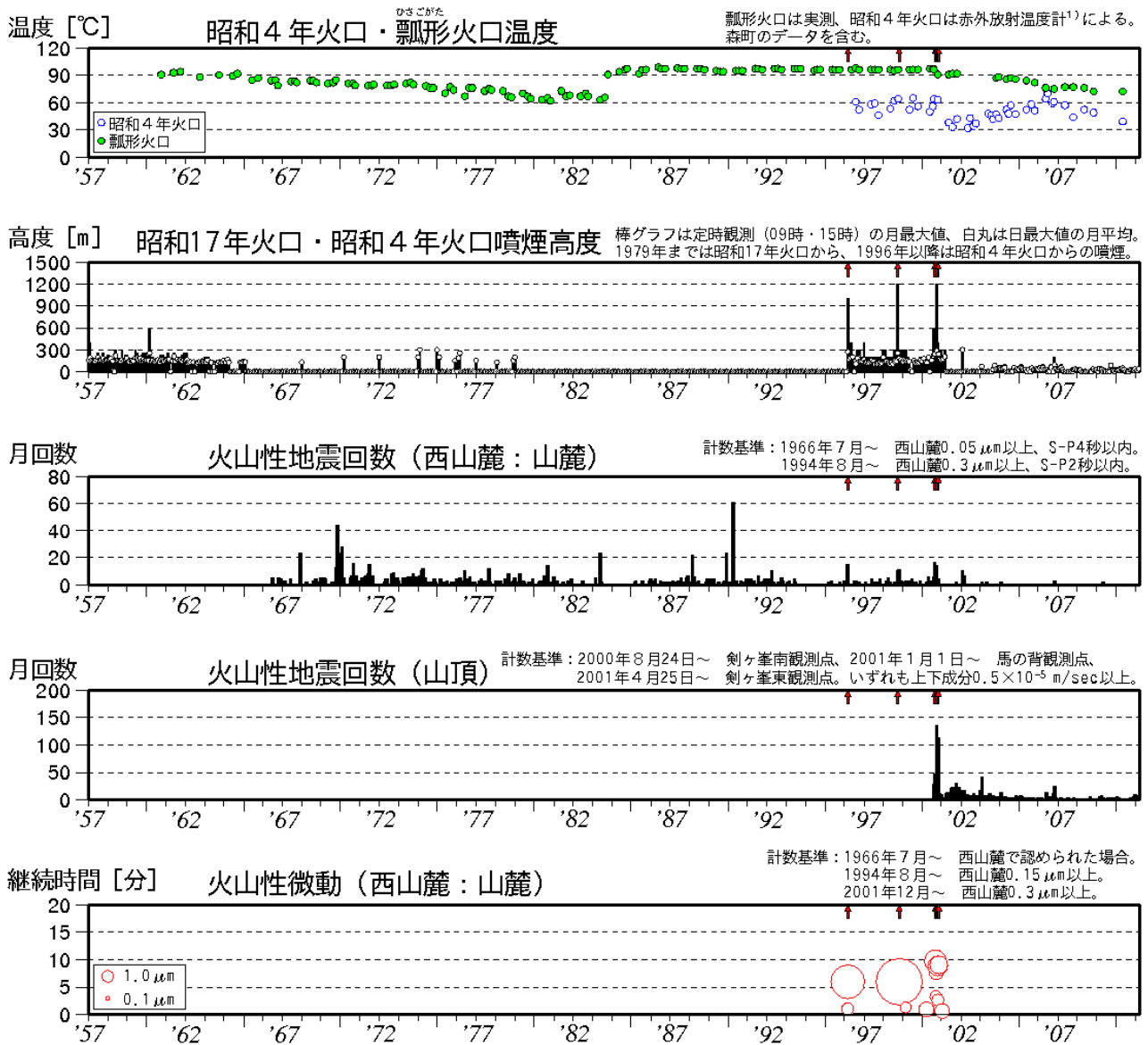
図1※ 北海道駒ヶ岳 長期の火山活動経過図（1957年1月～2011年3月） ↑印は噴火
