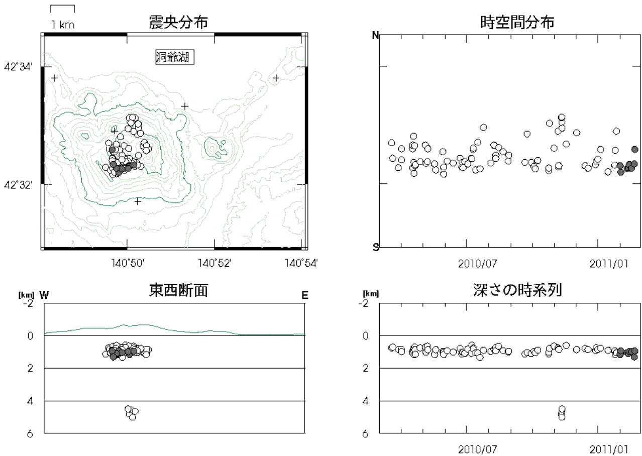
図 3 有珠山 震源分布図（2010 年 3 月～2011 年 2 月、+は地震観測点）
