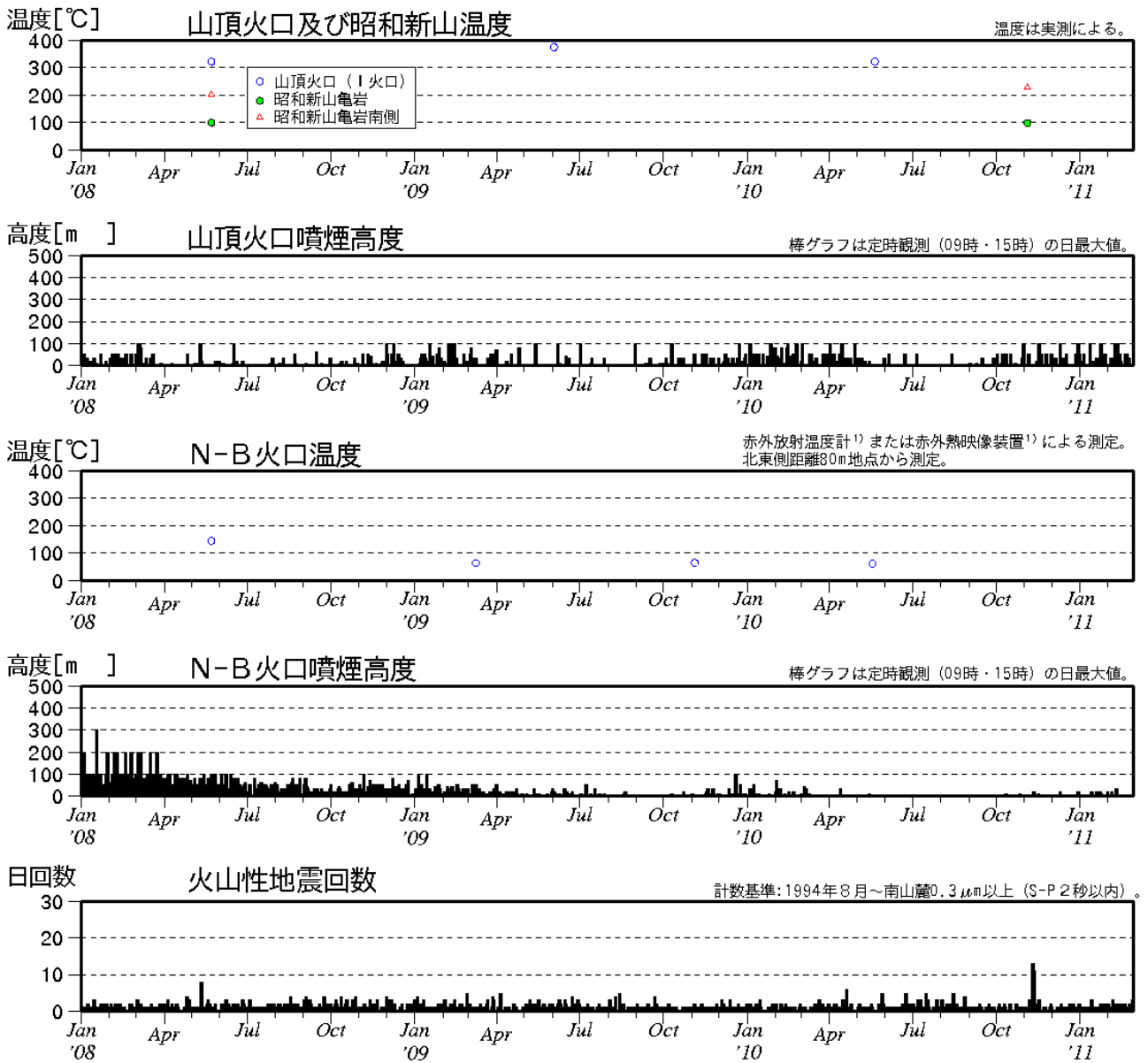
図2 有珠山 最近の火山活動経過図（2008年1月～2011年2月）
