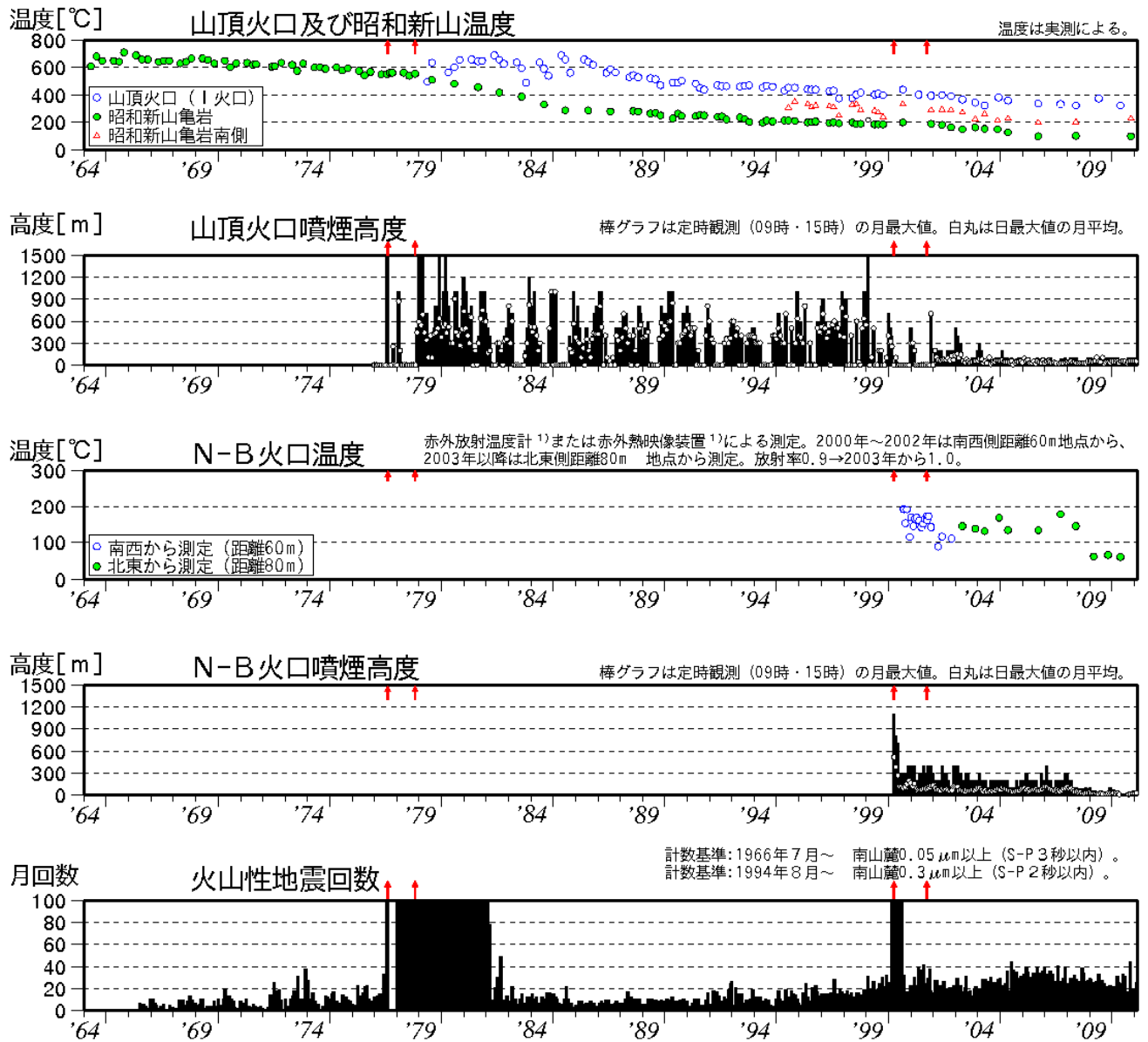
図 1 有珠山 長期の火山活動経過図（1964 年 1 月～2011 年 2 月）
