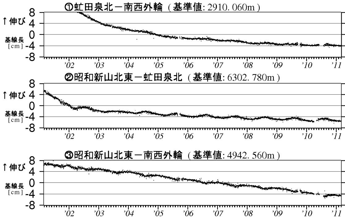
図 4 有珠山 GPS 連続観測による基線長変化（2001 年 3 月～2011 年 2 月） グラフの空白部分は欠測
