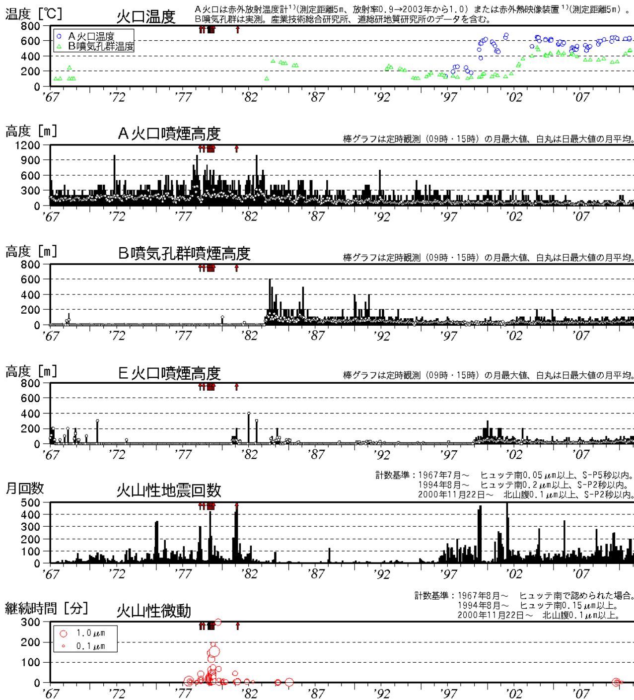
図 1※ 樽前山 長期の火山活動経過図 (1967年 1 月～2011年 2 月) ↑印は噴火
