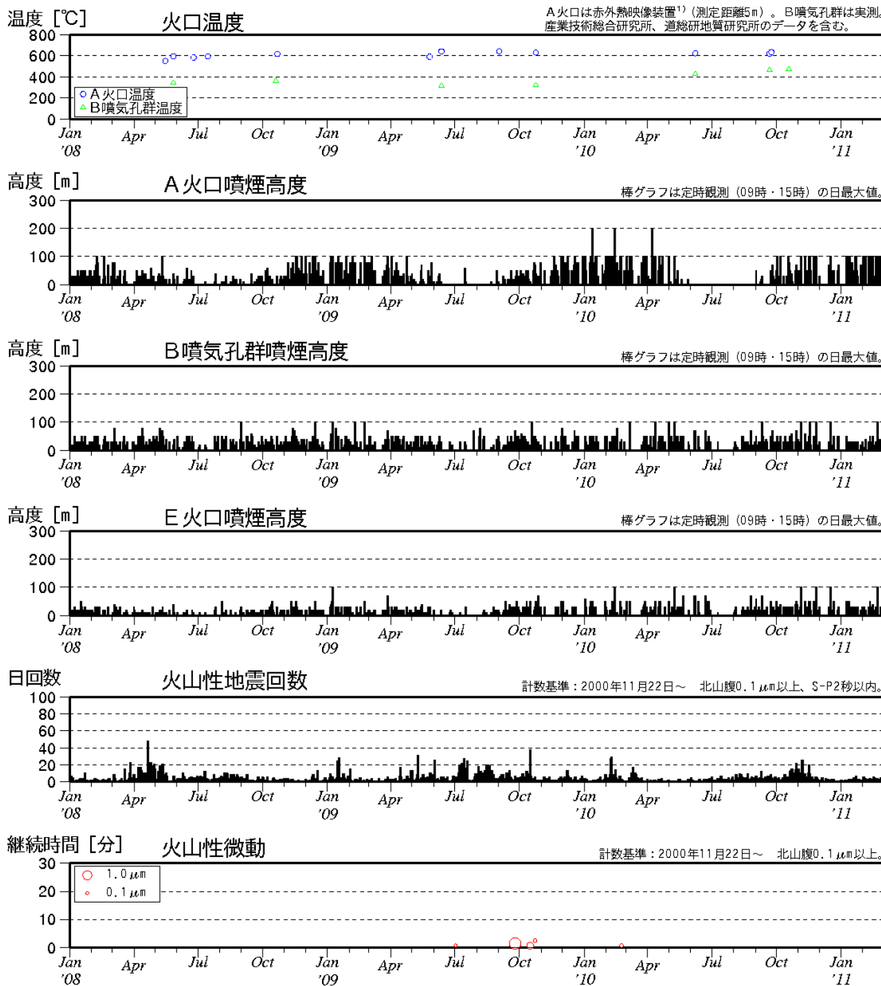
図 2※ 樽前山 最近の火山活動経過図（2008 年 1 月～2011 年 2 月）
