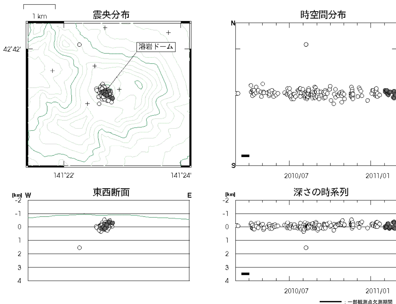
図 5 樽前山 震源分布図 (2010 年 3 月~2011 年 2 月、+は地震観測点)
