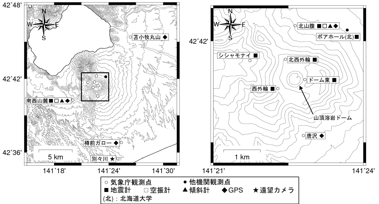
図 8 樽前山 観測点配置図
