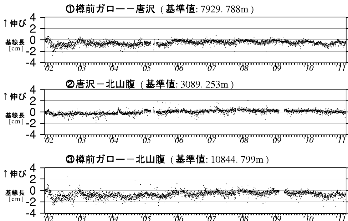
図 6 樽前山 GPS 連続観測による基線長変化 (2001 年 12 月～2011 年 2 月)
