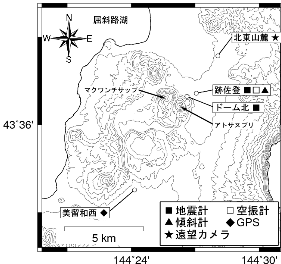
図3 アトサヌプリ 観測点配置図
