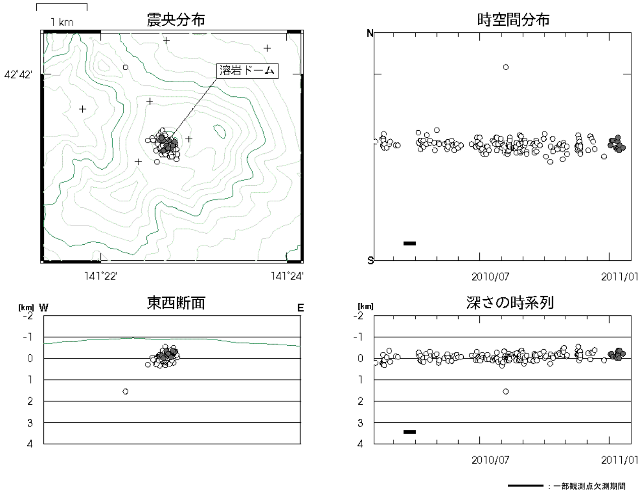
図 5※ 樽前山 震源分布図 (2010 年 2 月～2011 年 1 月、+は地震観測点)
