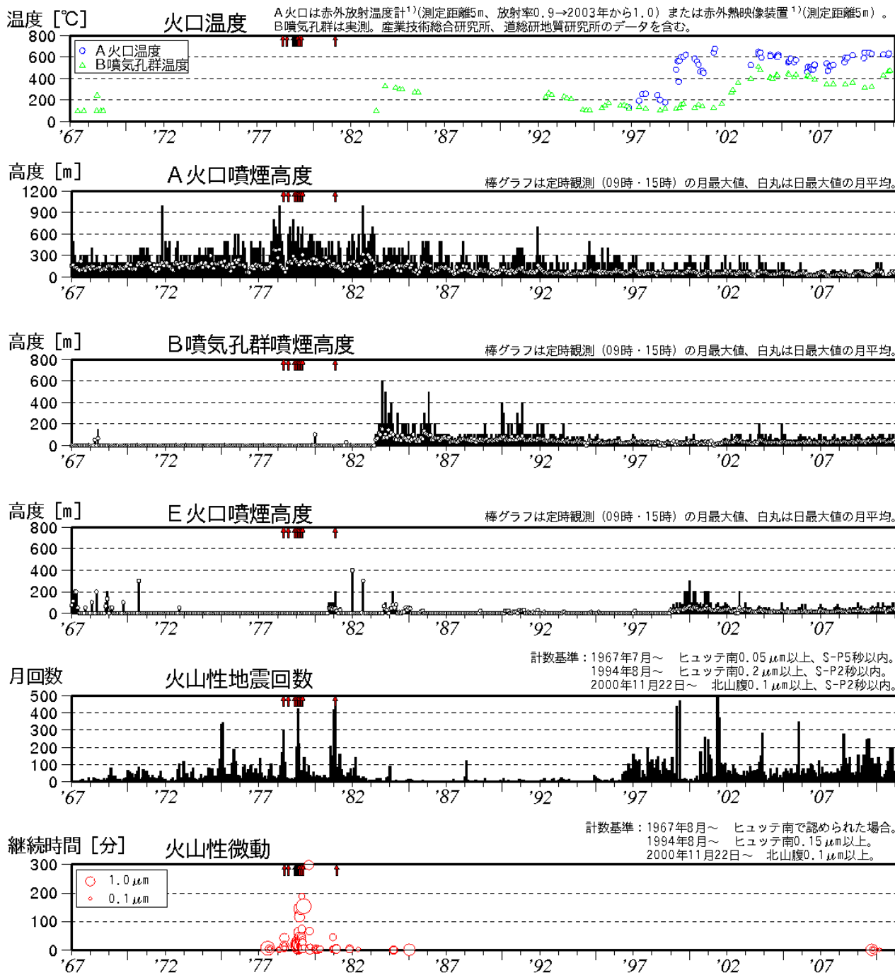
図 1※ 樽前山 長期の火山活動経過図（1967年 1 月～2011年 1 月） ↑印は噴火
