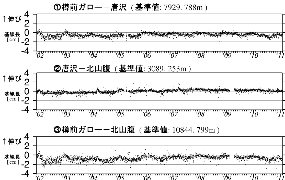
図 6 樽前山 GPS 連続観測による基線長変化 (2001 年 12 月～2011 年 1 月)
