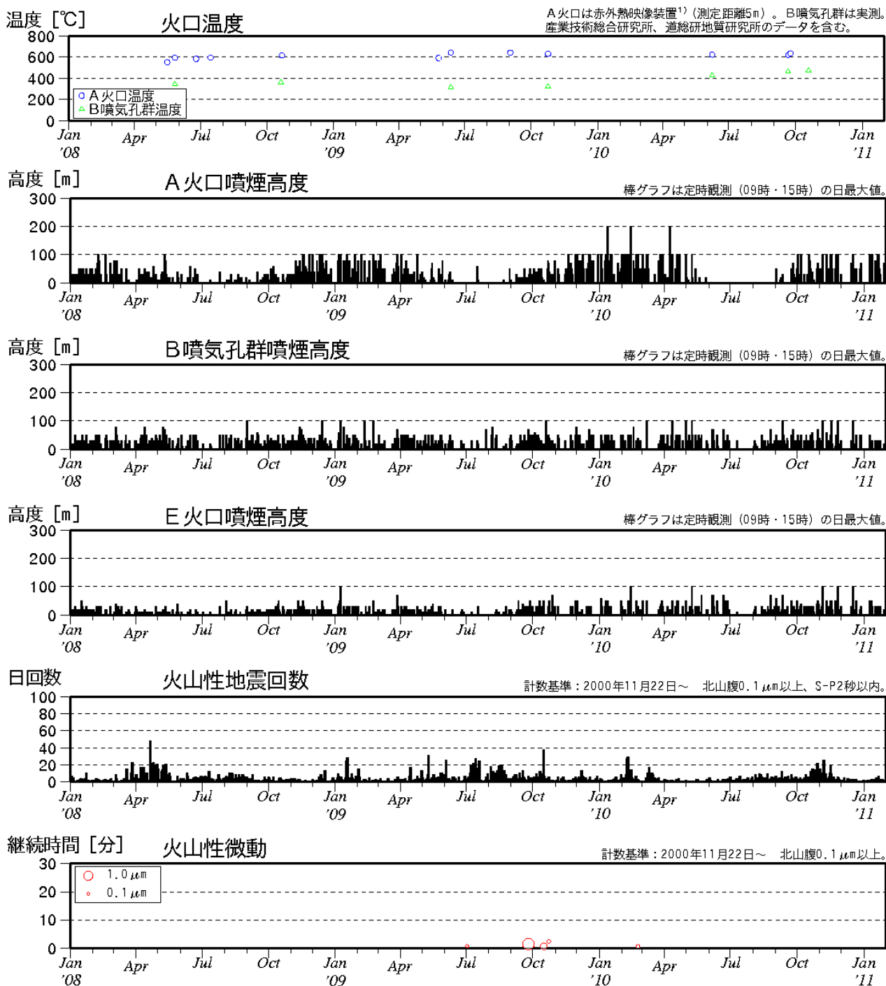
図 2※ 樽前山 最近の火山活動経過図 (2008 年 1 月～2011 年 1 月)
