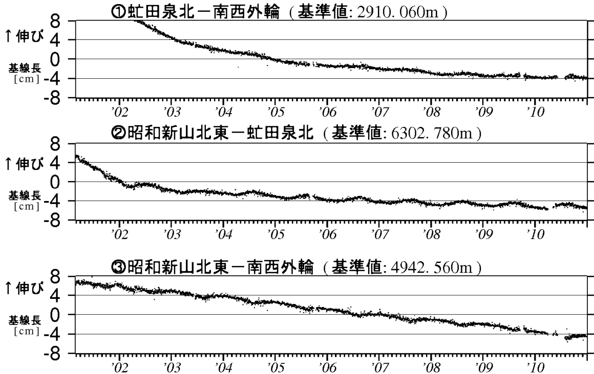
図 4 有珠山 GPS 連続観測による基線長変化 (2001 年 3 月～2010 年 12 月)
