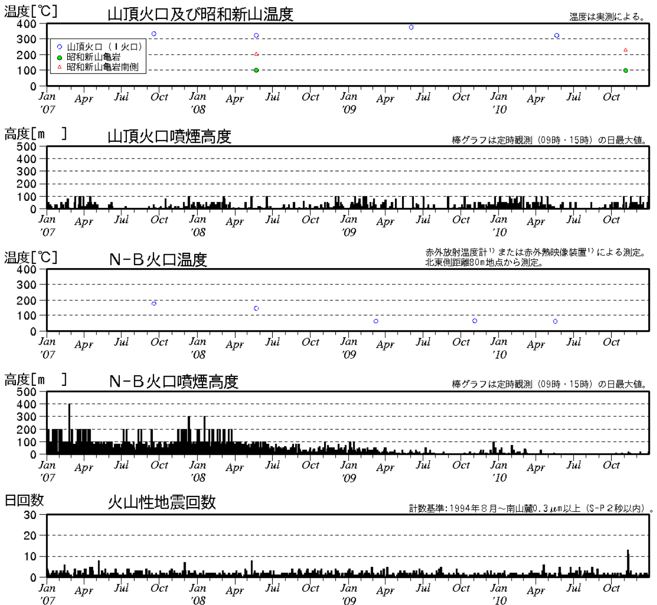
図 2 有珠山 最近の火山活動経過図（2007 年 1 月～2010 年 12 月）
