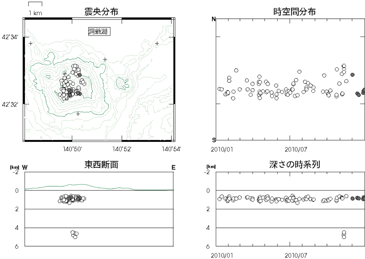
図 3 有珠山 震源分布図（2010 年 1 月～2010 年 12 月、+は地震観測点）
