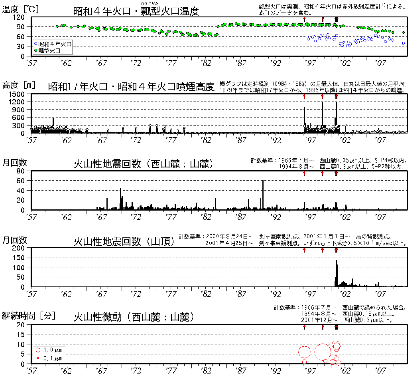
図 1※ 北海道駒ヶ岳 長期の火山活動経過図（1957 年 1 月～2010 年 11 月）↑印は噴火
