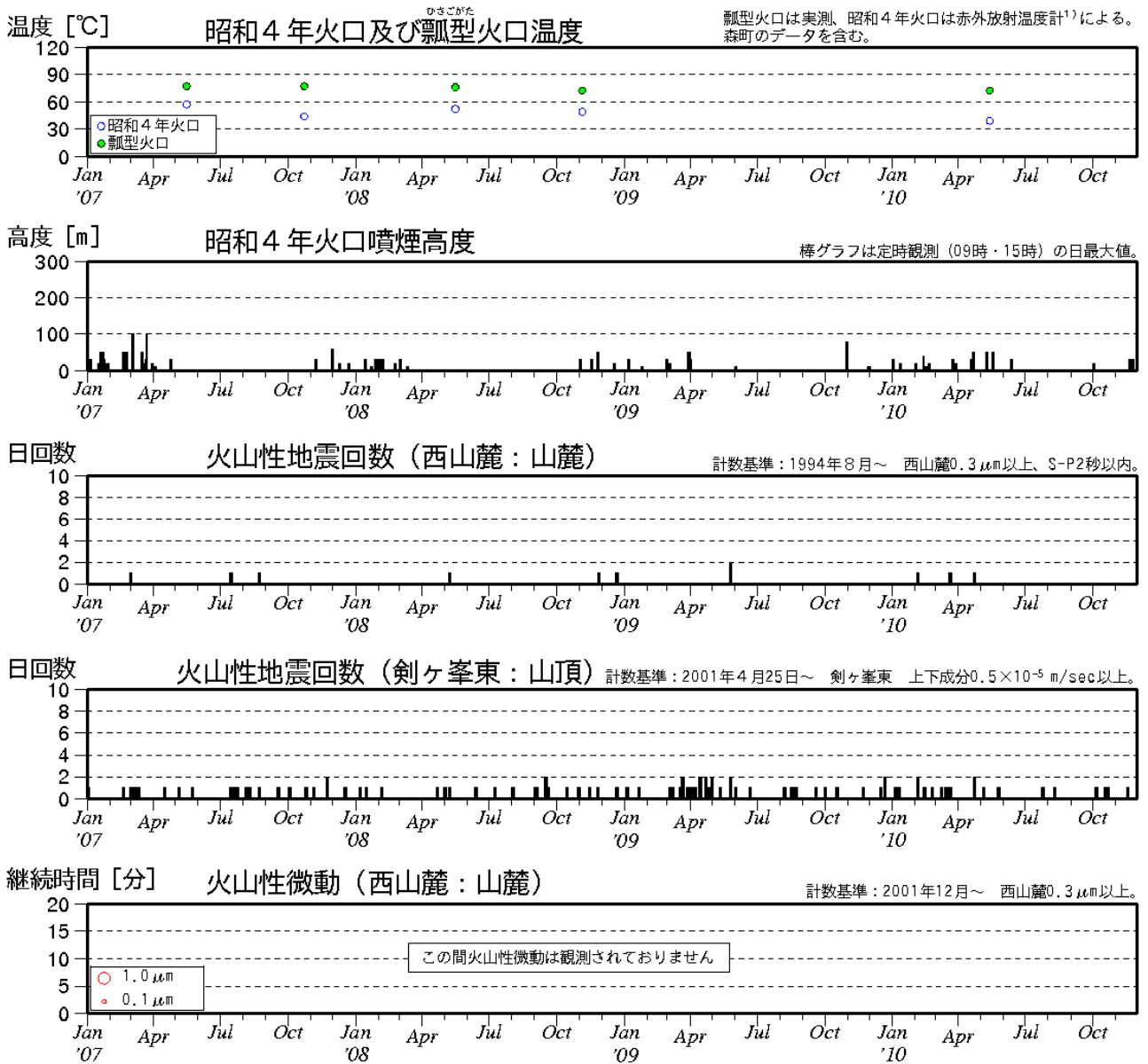
図2※ 北海道駒ヶ岳 最近の火山活動経過図（2007年1月～2010年11月）
