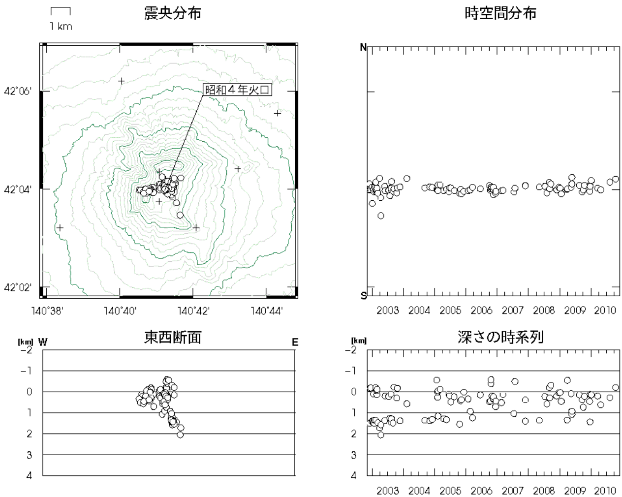
図 3※ 北海道駒ヶ岳 震源分布図（2002 年 11 月～2010 年 11 月、+は地震観測点）
