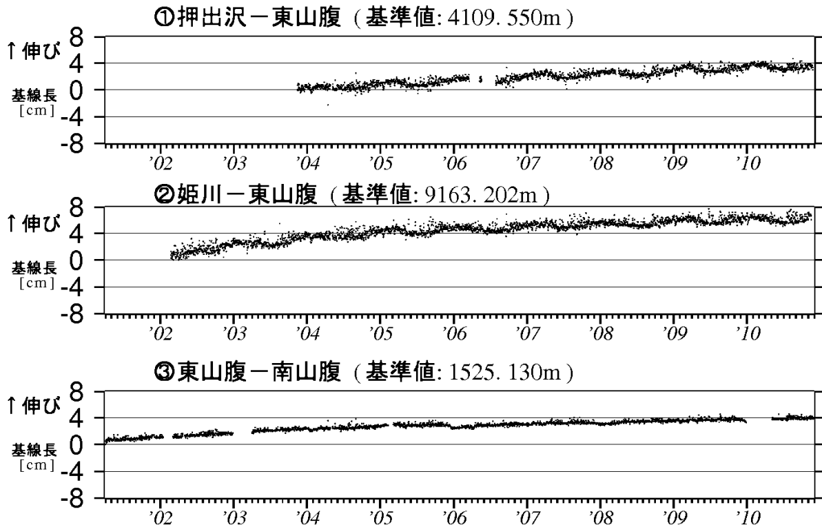
図 4 北海道駒ヶ岳 GPS 連続観測による基線長変化（2001 年 4 月～2010 年 11 月） グラフの空白部分は欠測 図 4 の①～③は、図 5 の GPS 基線①～③に対応しています。 姫川観測点は 2010 年 10 月 29 日に機器の更新を行いました。
