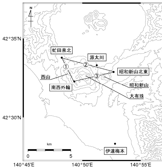
図 5 有珠山 GPS 連続観測点配置図
