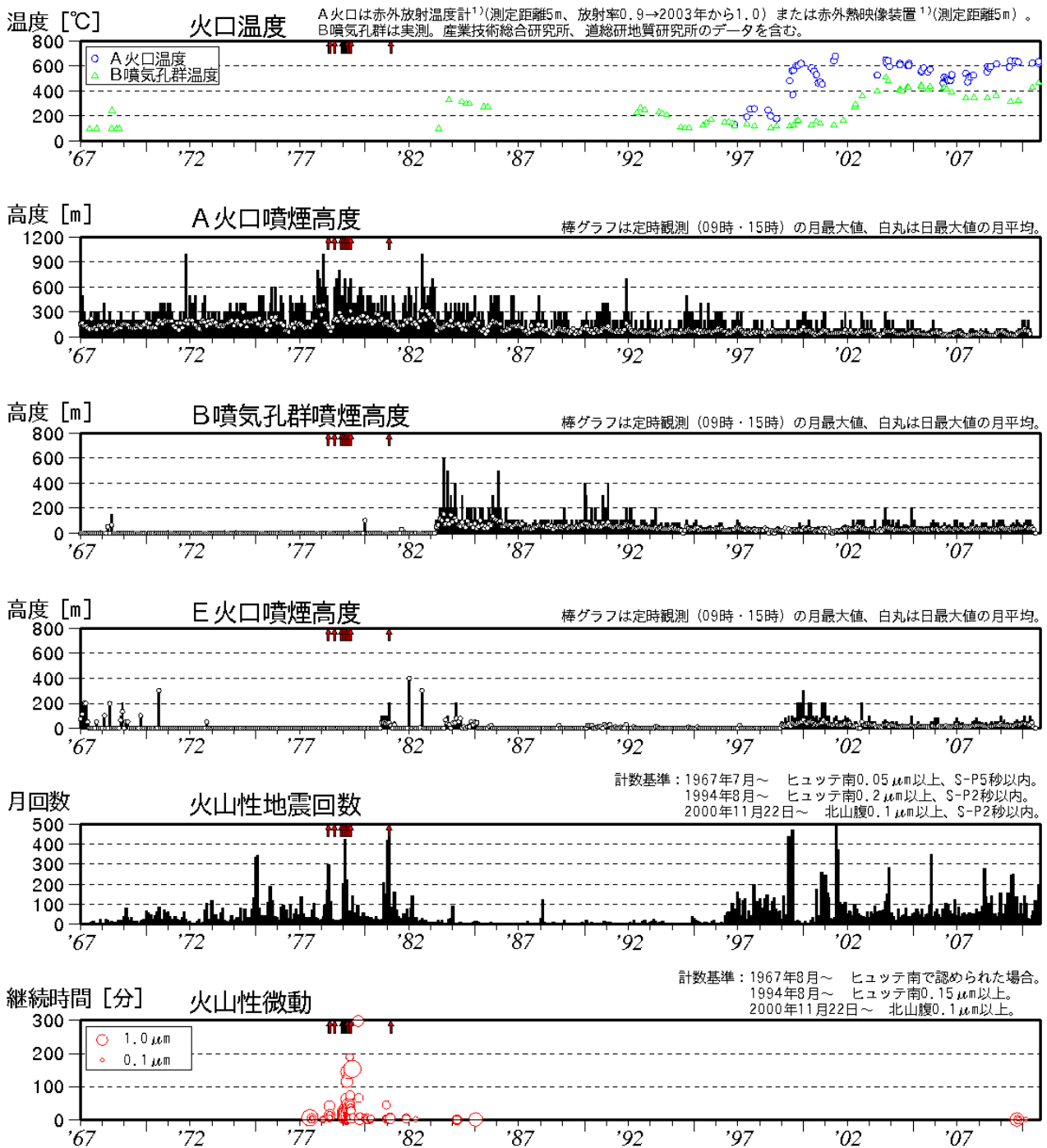
図 1※ 樽前山 長期の火山活動経過図 (1967年 1 月～2010年10月) ↑印は噴火
