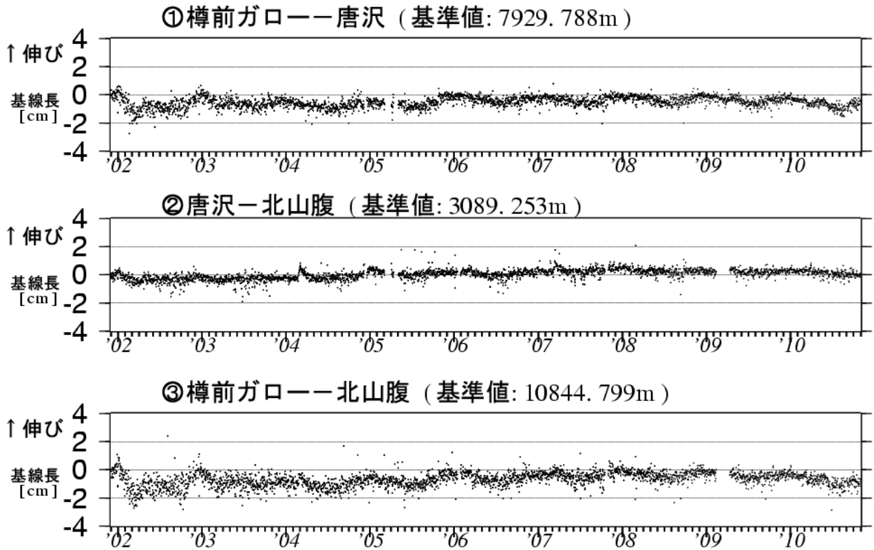
図 4 樽前山 GPS 連続観測による基線長変化 (2001 年 12 月～2010 年 10 月)
