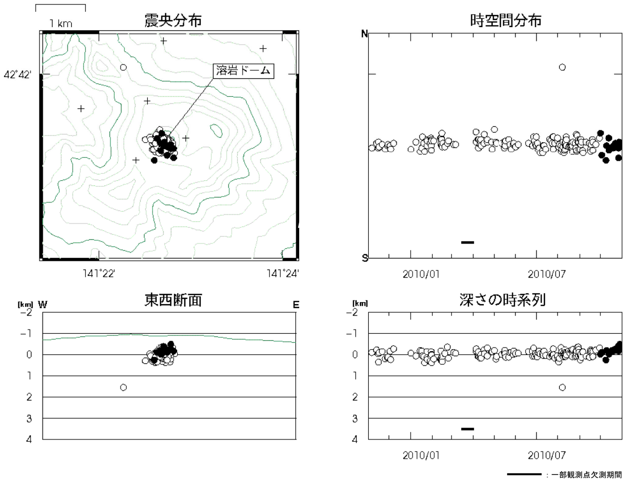
図 3※ 樽前山 震源分布図 (2009 年 11 月~2010 年 10 月、+は地震観測点)
