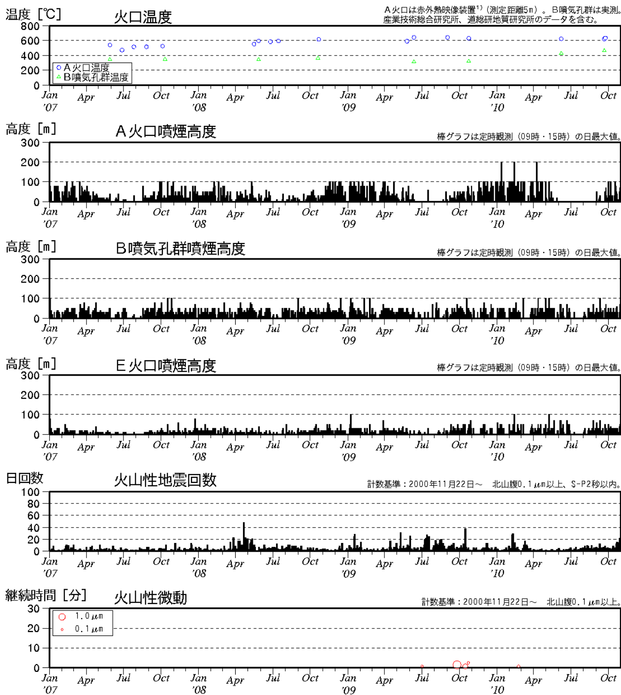
図 2 ※ 樽前山 最近の火山活動経過図 (2007 年 1 月～2010 年 10 月)
