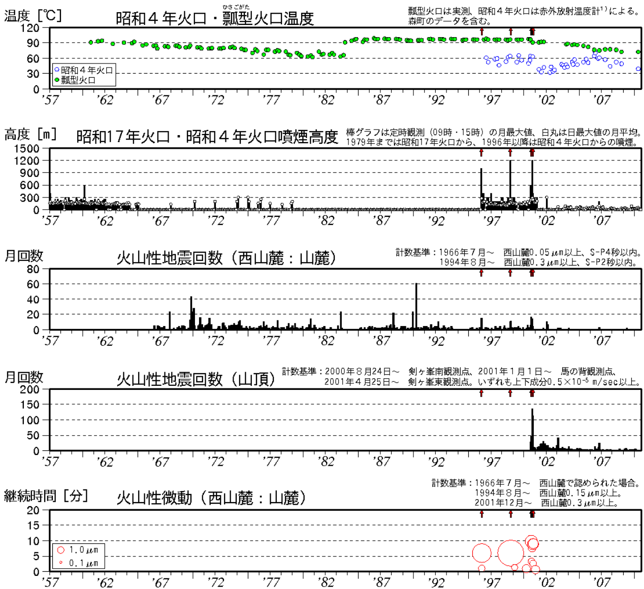
図 1※ 北海道駒ヶ岳 長期の火山活動経過図（1957 年 1 月～2010 年 9 月） ↑印は噴火
