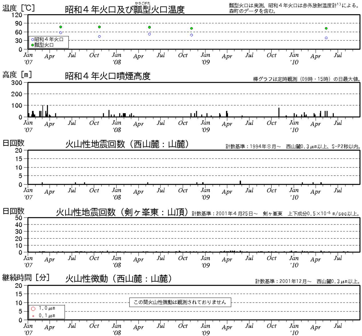
図 2* 北海道駒ヶ岳 最近の火山活動経過図（2007年1月～2010年9月）
