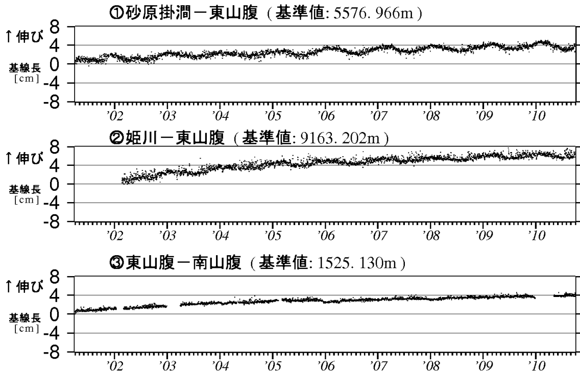
図 4 北海道駒ヶ岳 GPS 連続観測による基線長変化（2001 年 4 月～2010 年 9 月）
