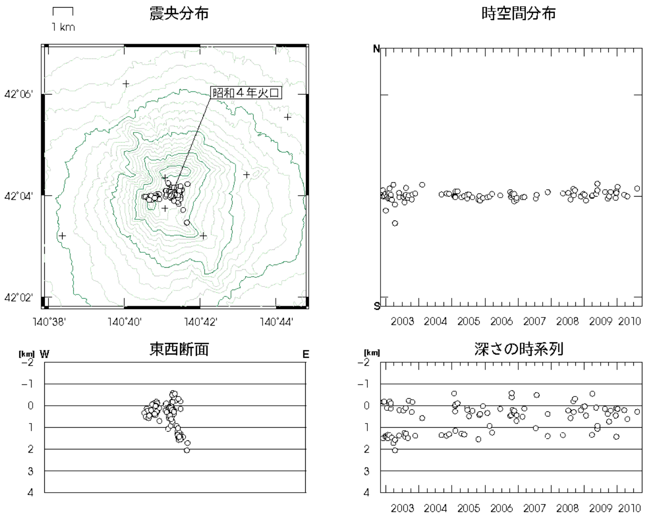
図 3 ※ 北海道駒ヶ岳 震源分布図（2002 年 11 月～2010 年 9 月、+は地震観測点）
