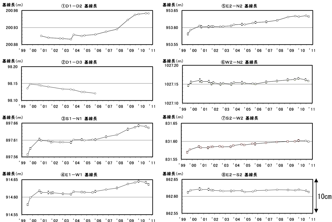
図 8 樽前山 GPS 繰り返し観測による溶岩ドーム付近の基線長変化 (1999 年 7 月～2010 年 9 月) 図 8 の①～⑧は図 9 の①～⑧に対応しています。
