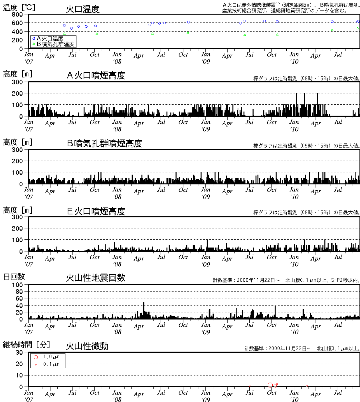
図 2 ※ 樽前山 最近の火山活動経過図 (2007 年 1 月～2010 年 9 月)
