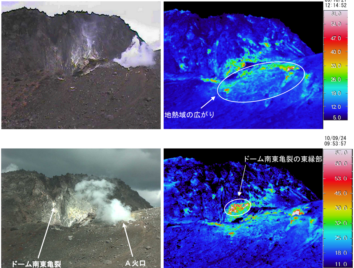
図3 樽前山 赤外熱映像装置 1) によるA火口、ドーム南東亀裂の地表面温度分布 (上段：2009年10月21日 下段：2010年9月24日 図4 ①より撮影)
