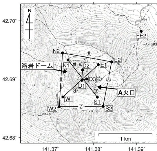
図 9 樽前山 GPS 繰り返し観測点配置図
