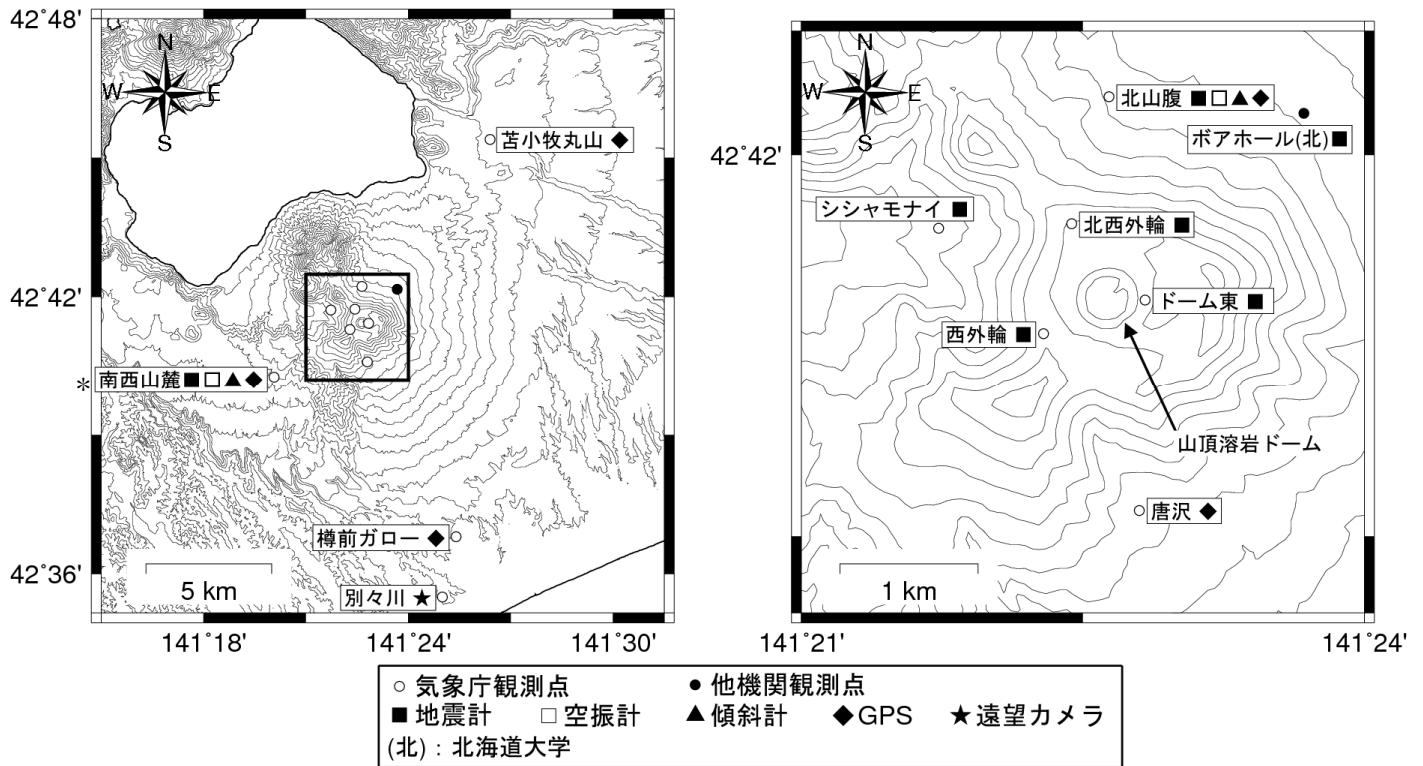
図 10 樽前山 観測点配置図
