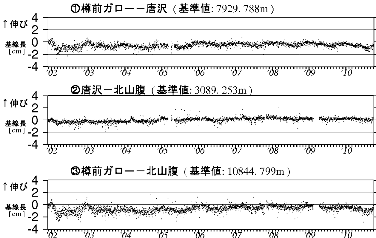
図 6 樽前山 GPS 連続観測による基線長変化 (2001 年 12 月～2010 年 9 月)
