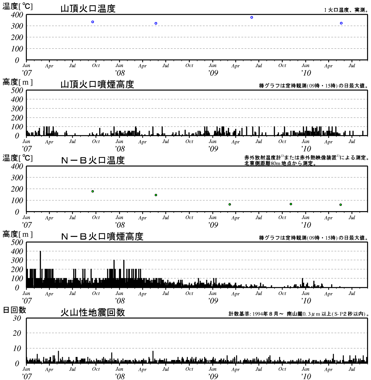
図2 有珠山 最近の火山活動経過図（2007年1月～2010年8月）
