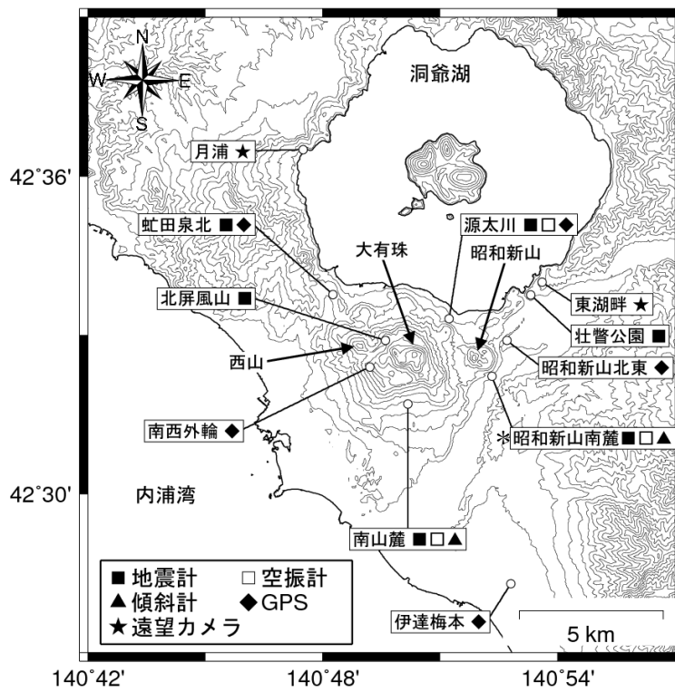
図 6 有珠山 観測点配置図
