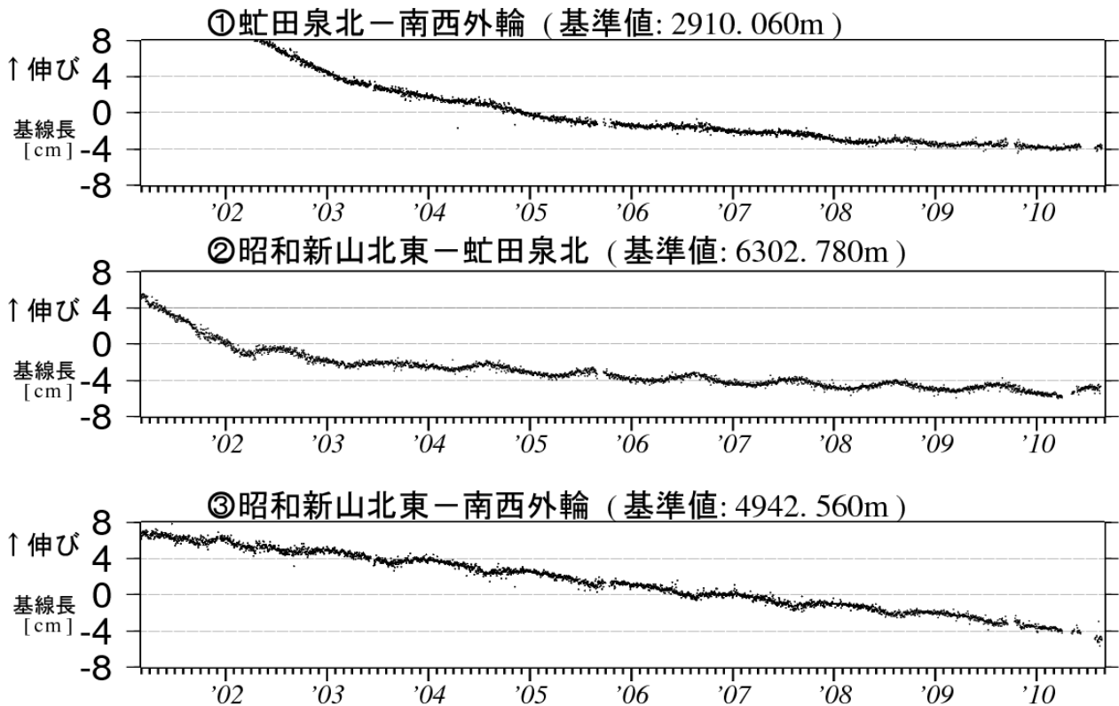
図 4 有珠山 GPS 連続観測による基線長変化（2001 年 3 月～2010 年 8 月）
