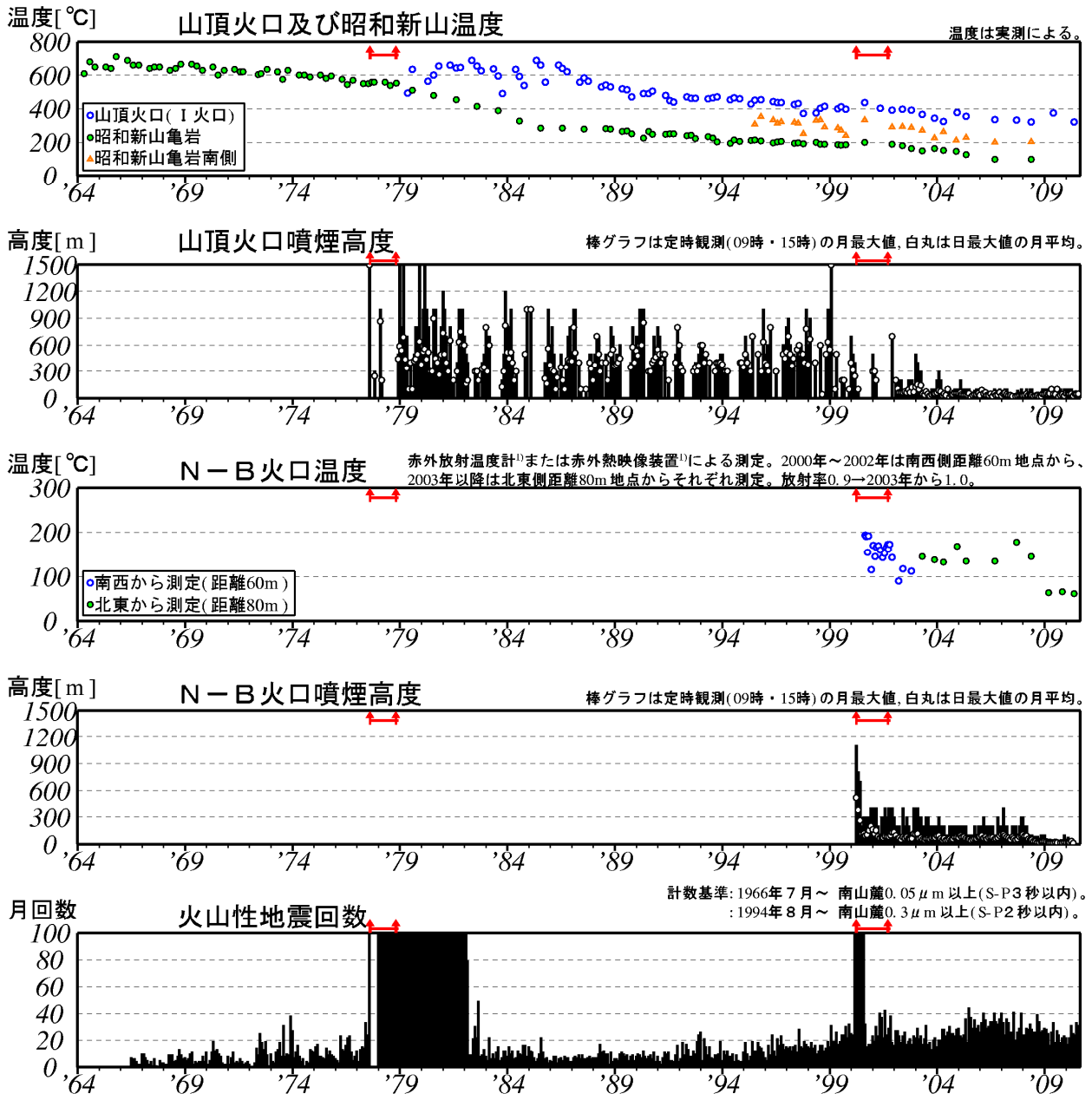
図 1 有珠山 長期の火山活動経過図（1964 年 1 月～2010 年 8 月）
