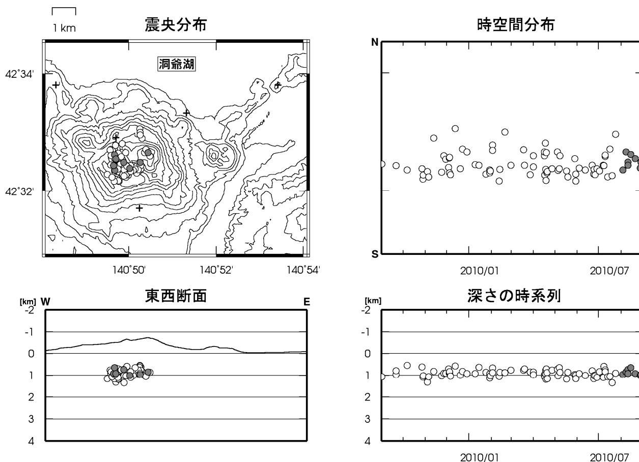
図 3 有珠山 震源分布図（2009 年 9 月～2010 年 8 月、+は地震観測点）
