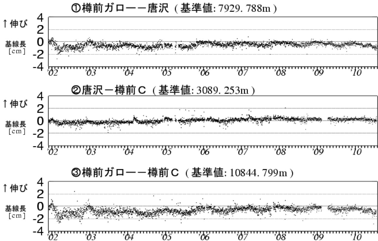
図 4 樽前山 GPS 連続観測による基線長変化 (2001 年 12 月～2010 年 7 月)
