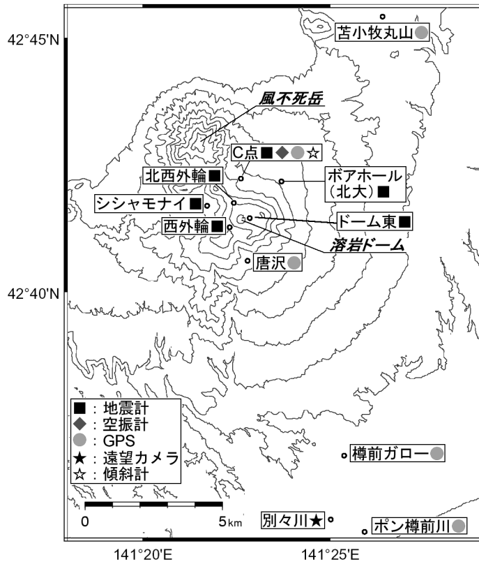
図 6 樽前山 従来の観測点配置図
