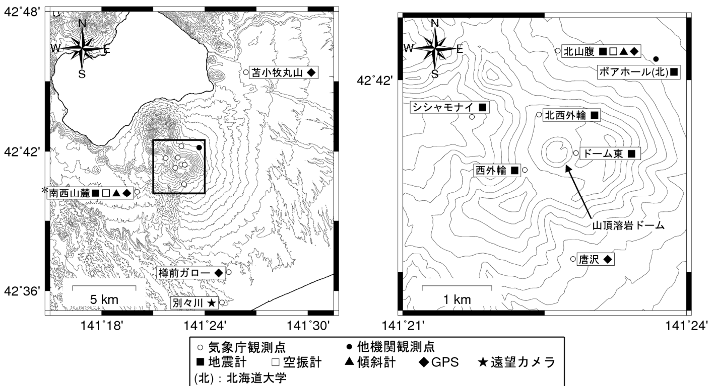
図 7 樽前山 新しい観測点名称を使用した観測点配置図
