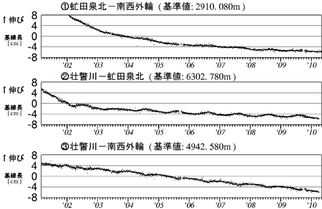
図5 有珠山 GPS 連続観測による基線長変化（2001 年 3 月～2010 年 4 月）
