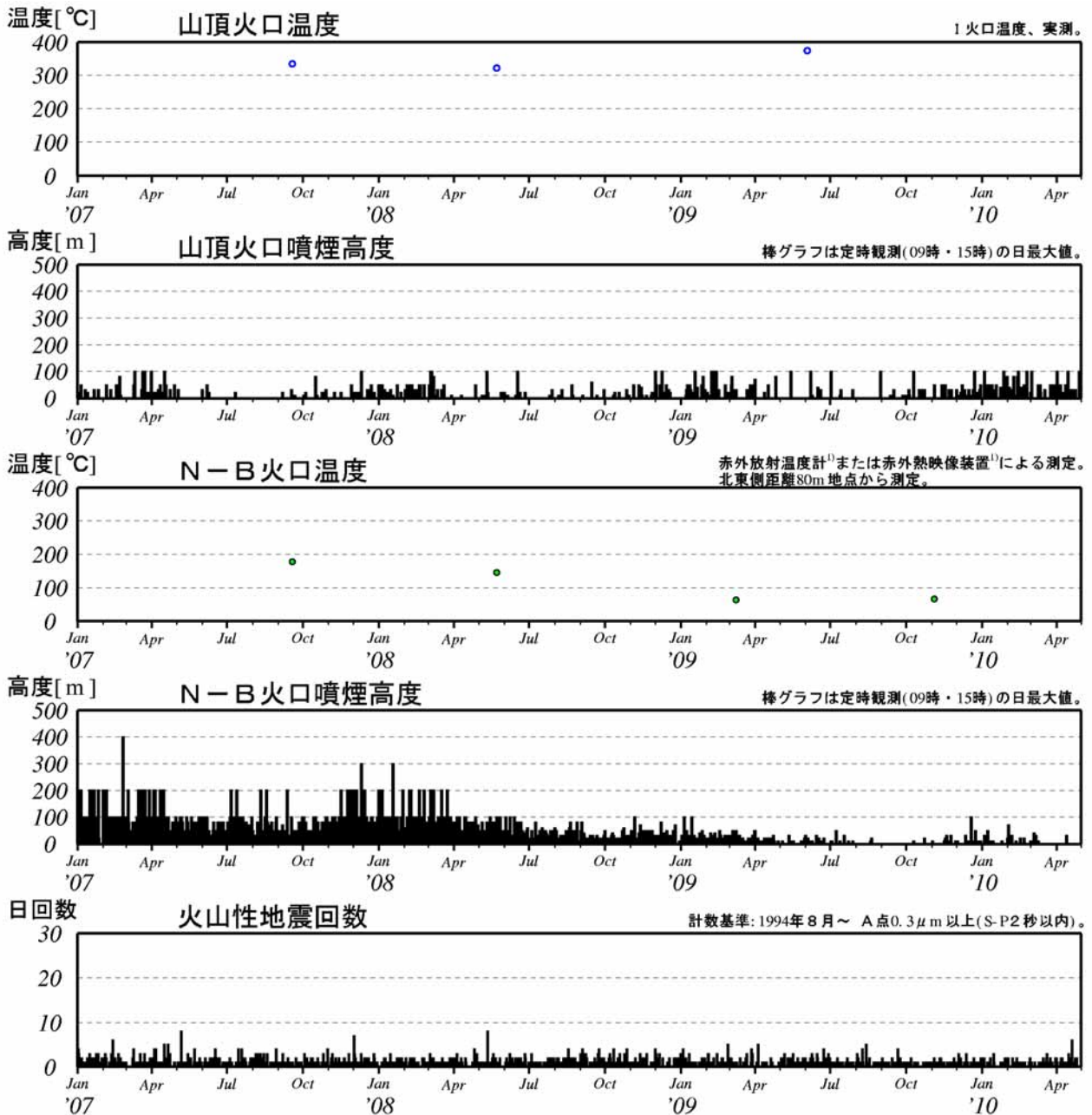
図3 有珠山 最近の火山活動経過図（2007年1月～2010年4月）
