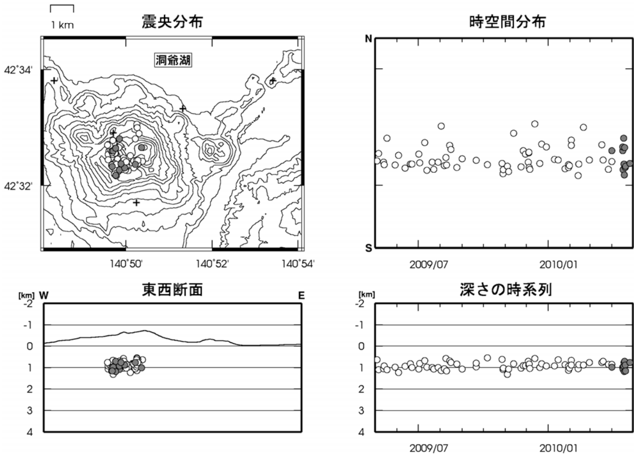
図4 有珠山 震源分布図(2009年5月~2010年4月、+は地震観測点)
