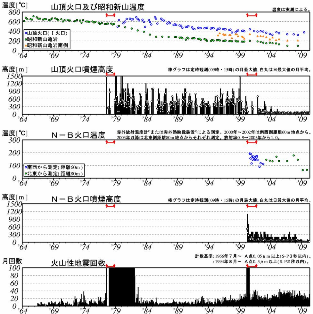
図 2 有珠山 長期の火山活動経過図（1964 年 1 月～2010 年 4 月）
