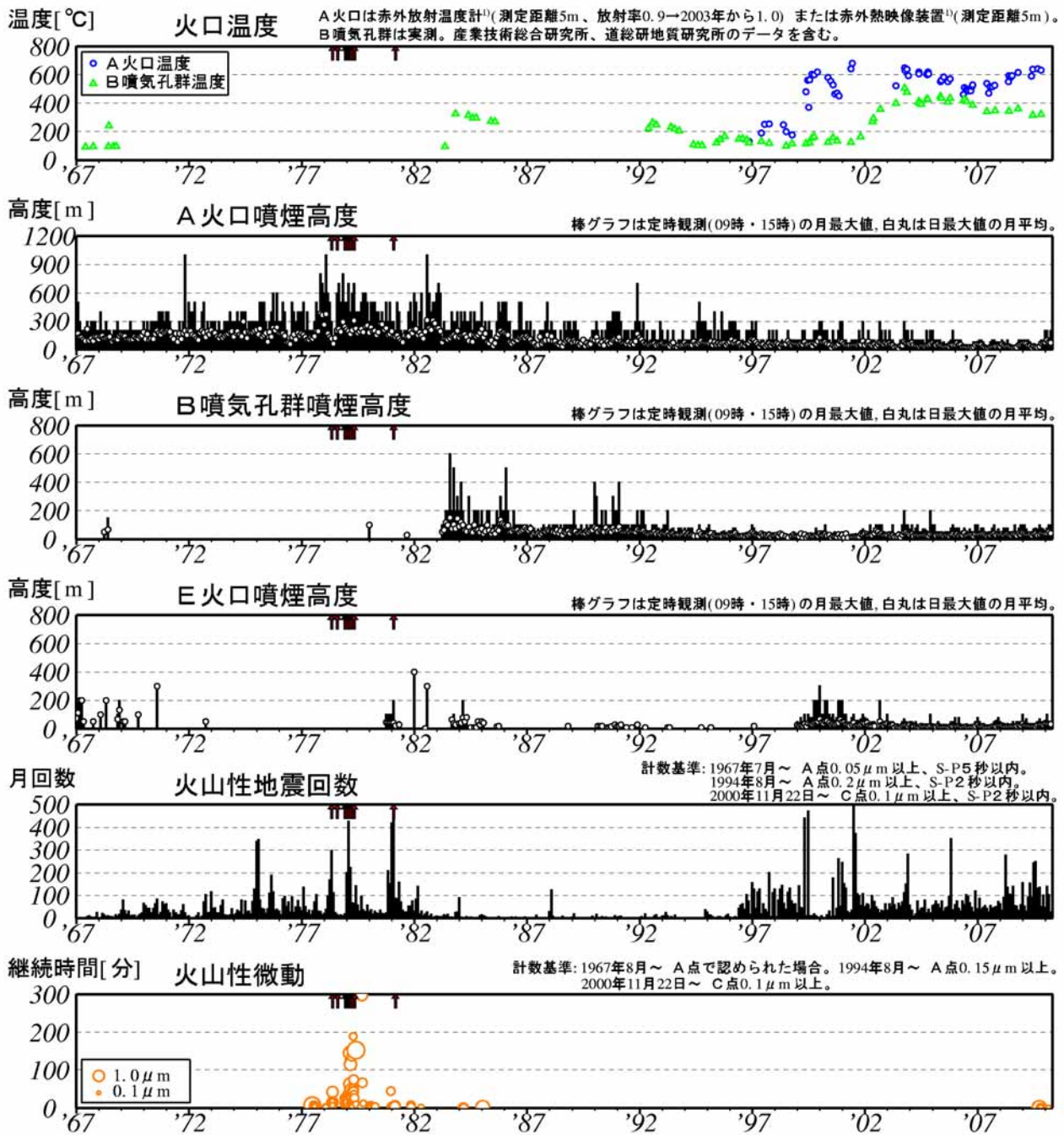
図2 樽前山 長期の火山活動経過図（1967年1月～2010年4月） 印は噴火
