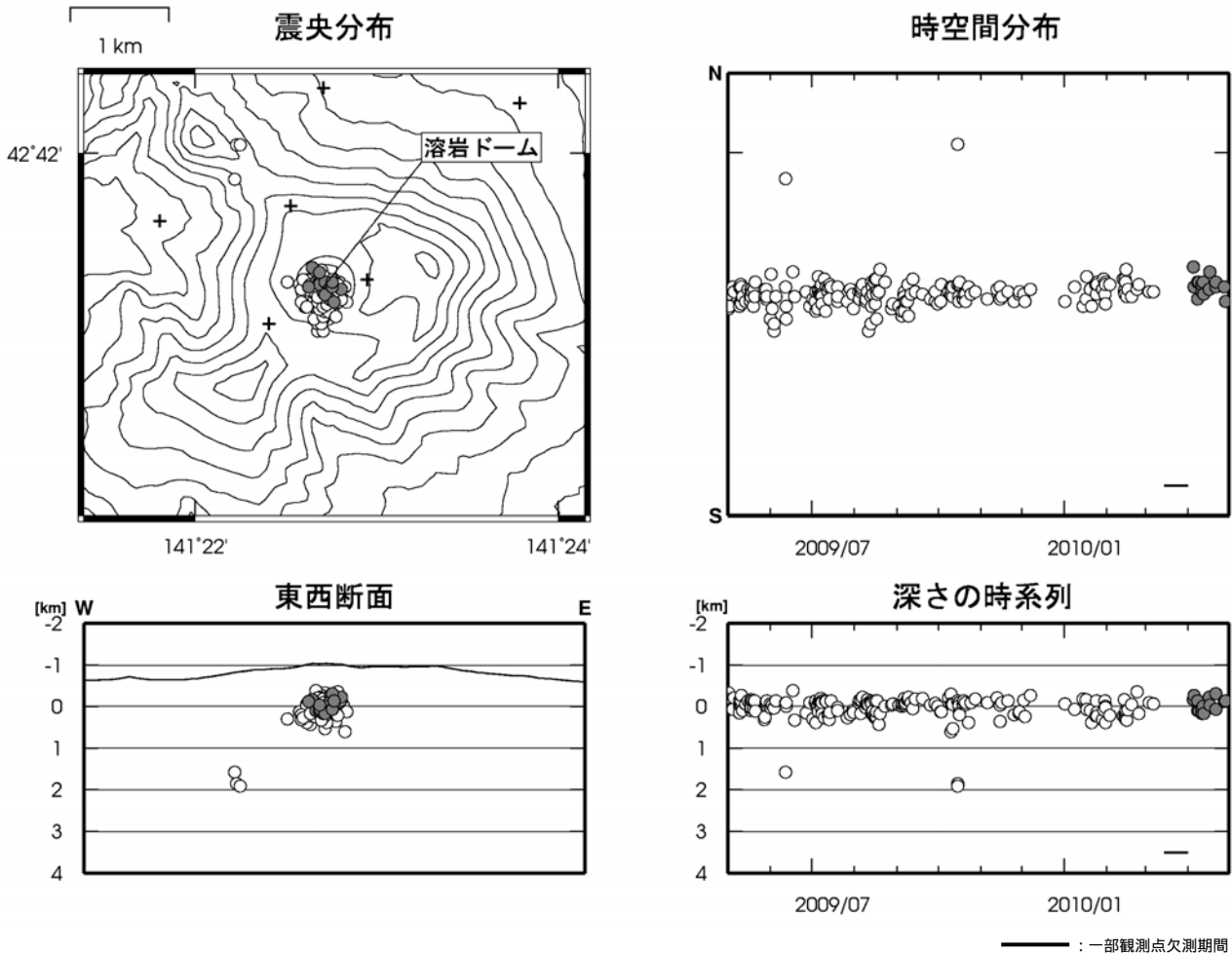
図4 樽前山 震源分布図(2009年5月~2010年4月、+は地震観測点)
