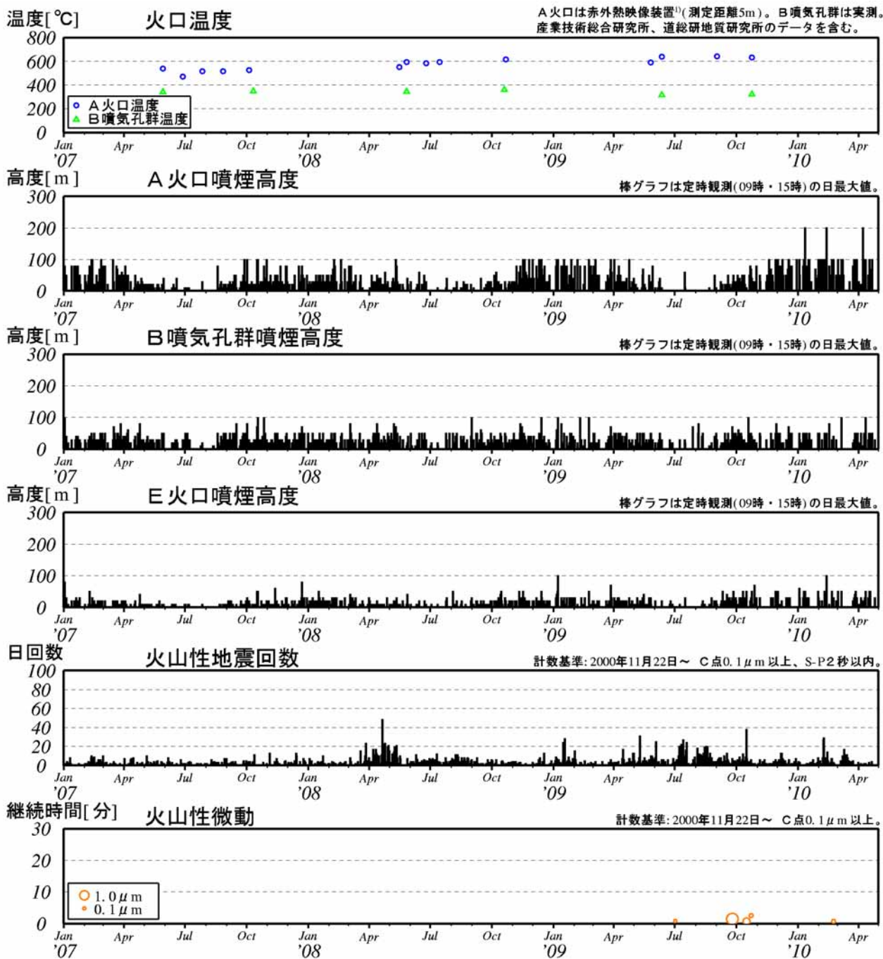
図3 樽前山 最近の火山活動経過図（2007年1月～2010年4月）
