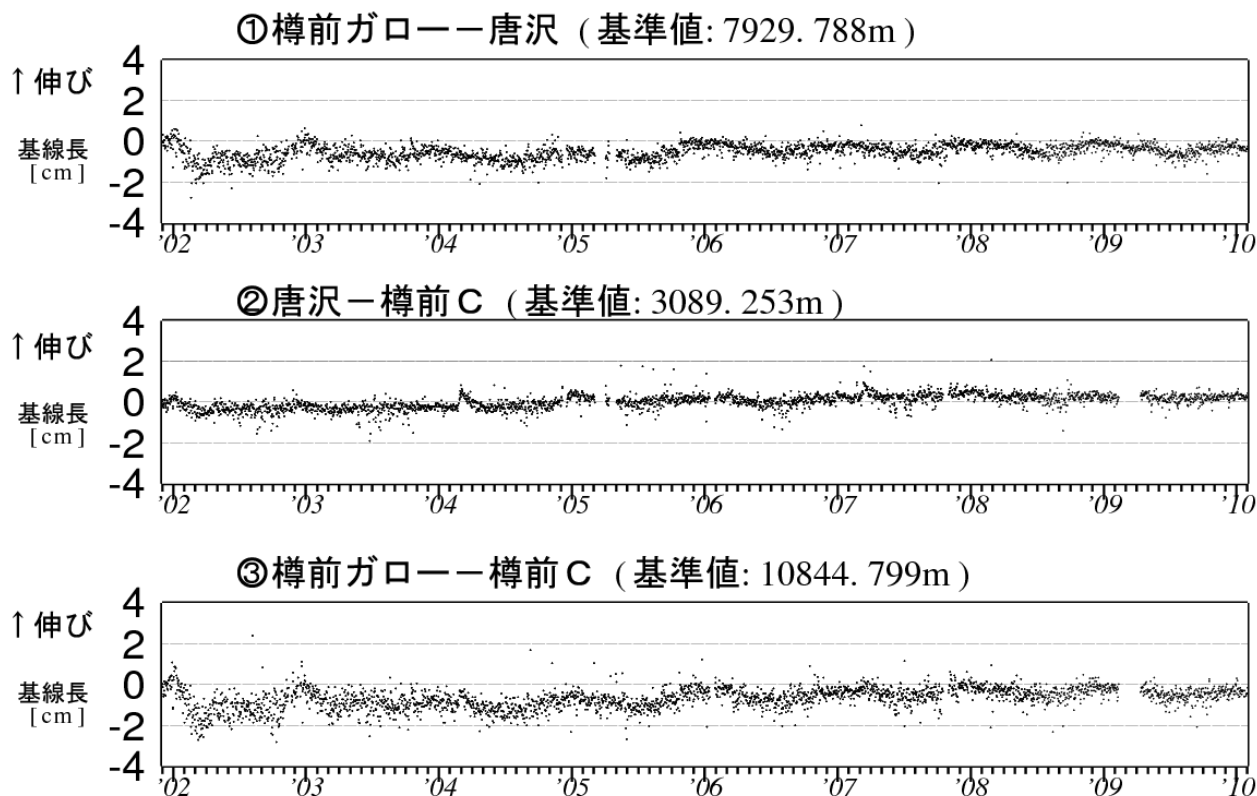
図5 樽前山 GPS 連続観測による基線長変化 (2001 年 12 月～2010 年 1 月)
