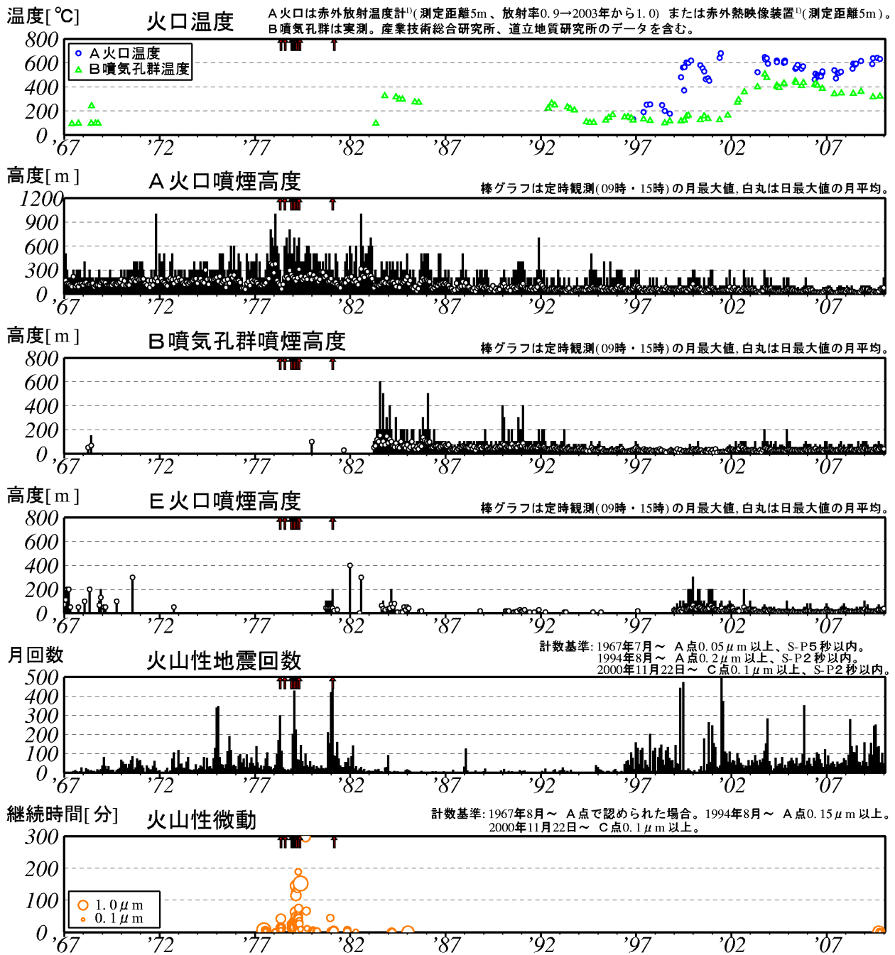
図 2* 樽前山 長期の火山活動経過図 (1967年 1 月～2010年 1 月) ↑印は噴火
