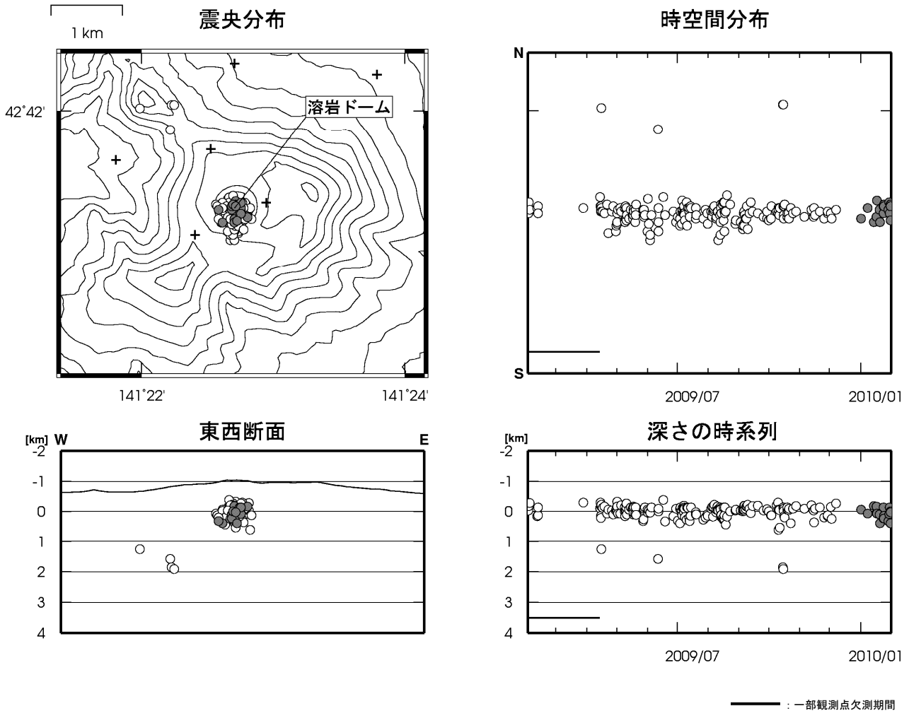
図 4※ 樽前山 震源分布図 (2009 年 2 月~2010 年 1 月、+は地震観測点)
