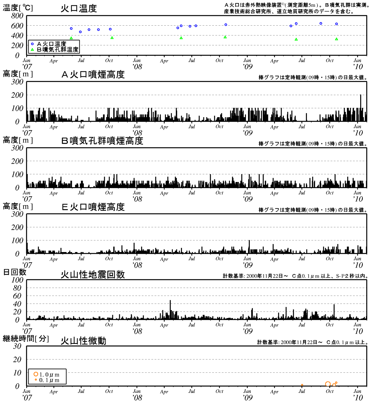
図 3※ 樽前山 最近の火山活動経過図 (2007 年 1 月～2010 年 1 月)
