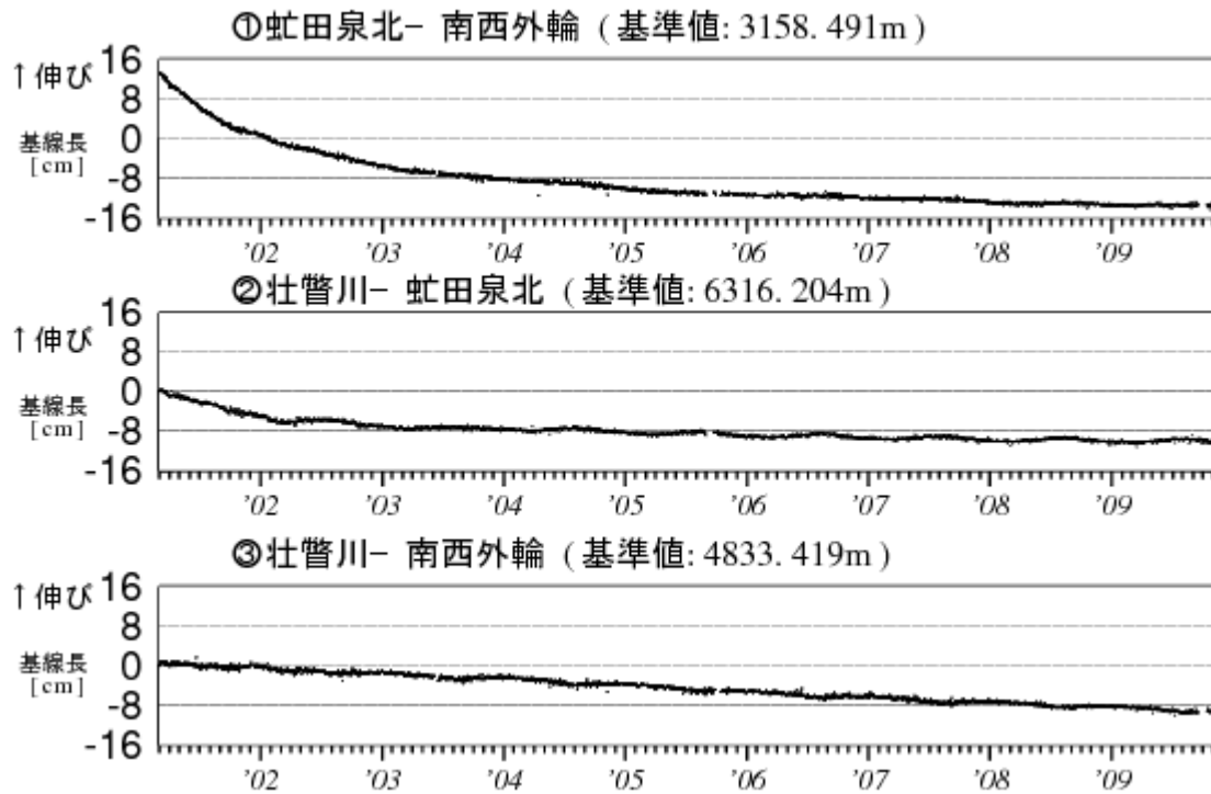
図5 有珠山 GPS 連続観測による基線長変化（2001年3月～2009年10月） グラフの空白部分は欠測 図5の①～③は、図6のGPS基線①～③に対応しています。
