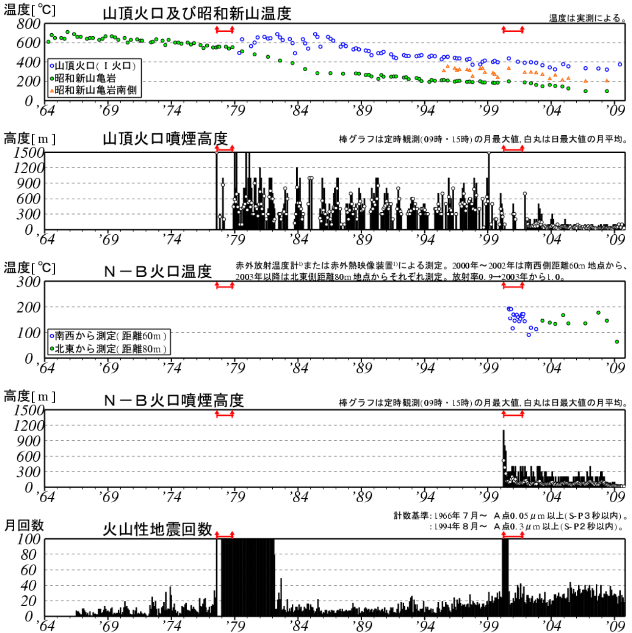
図2 有珠山 長期の火山活動経過図（1964年1月～2009年10月）
