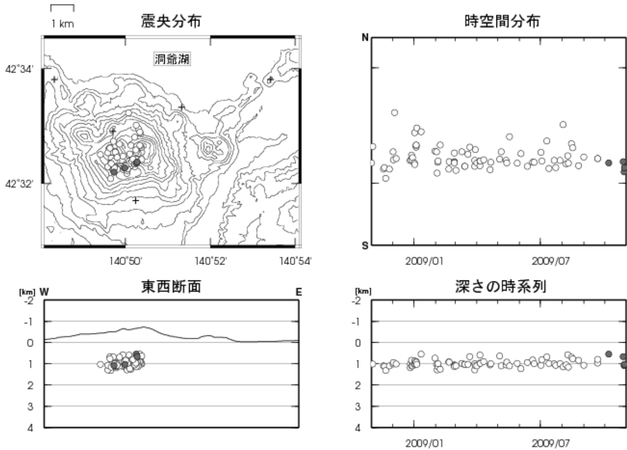
図 4 有珠山 震源分布図（2008 年 11 月～2009 年 10 月、+は地震観測点）
