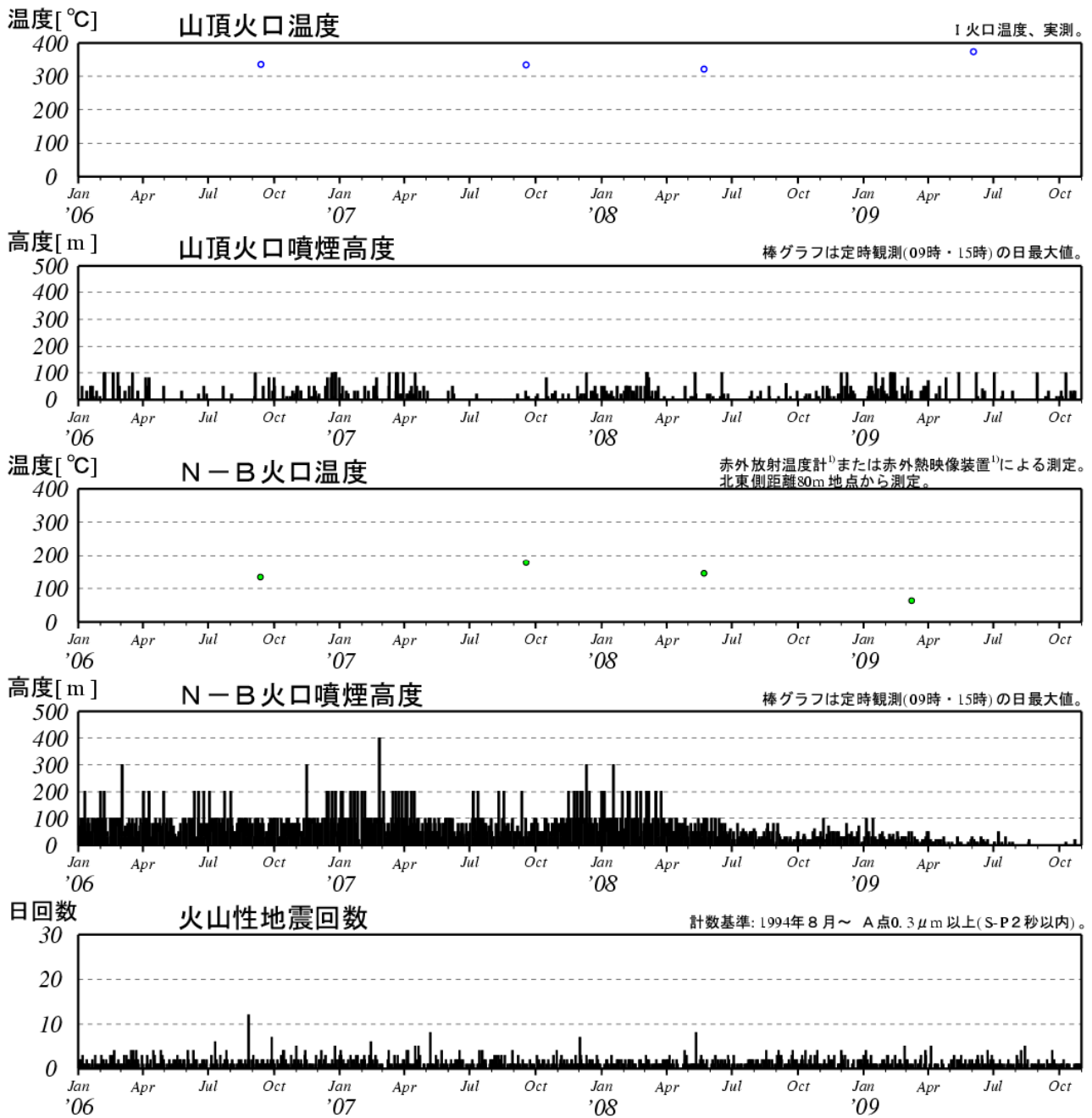
図3 有珠山 最近の火山活動経過図（2006年1月～2009年10月）
