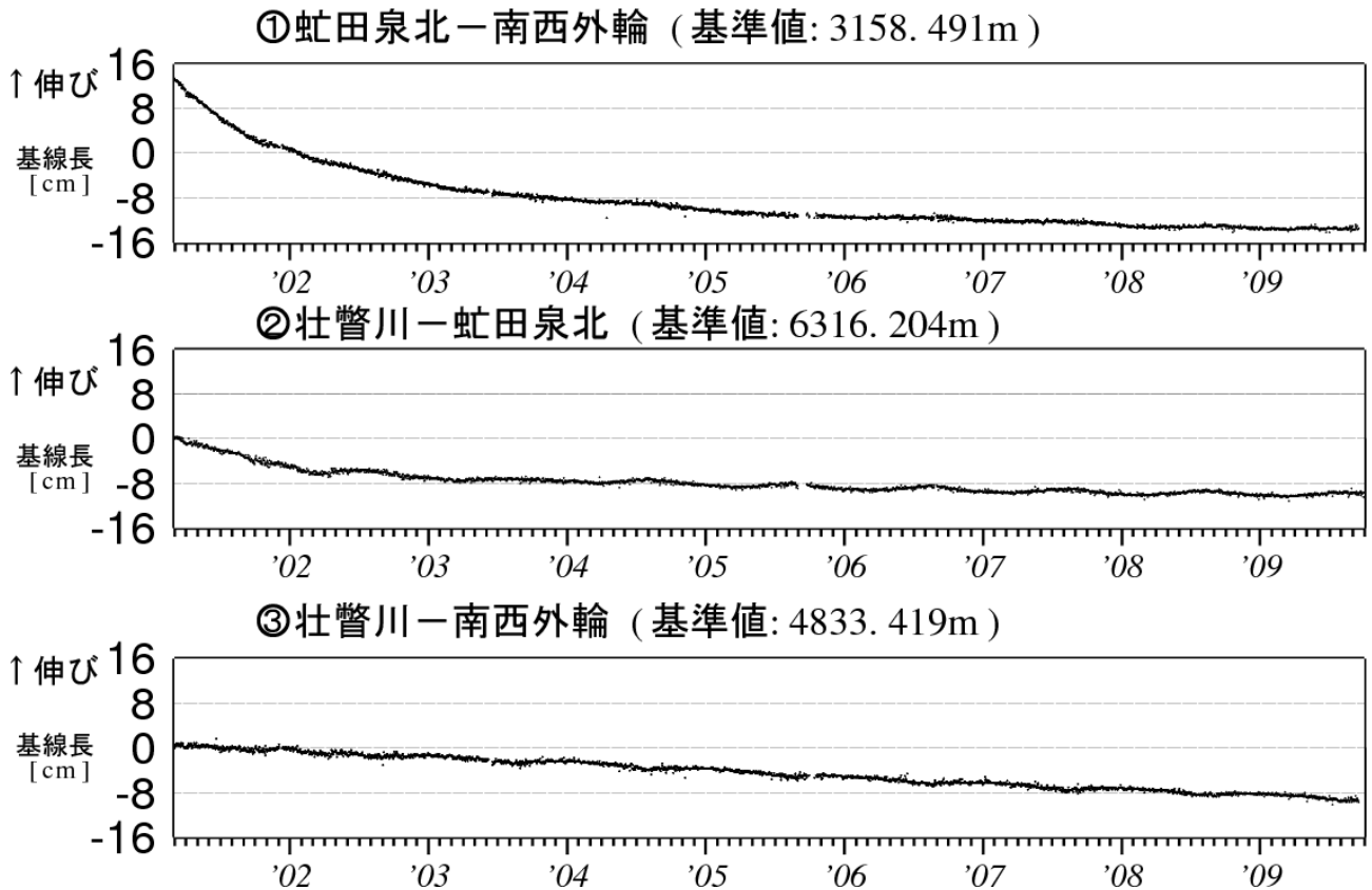
図5 有珠山 GPS 連続観測による基線長変化（2001年3月～2009年9月） グラフの空白部分は欠測 図5の①～③は、図6のGPS基線①～③に対応しています。
