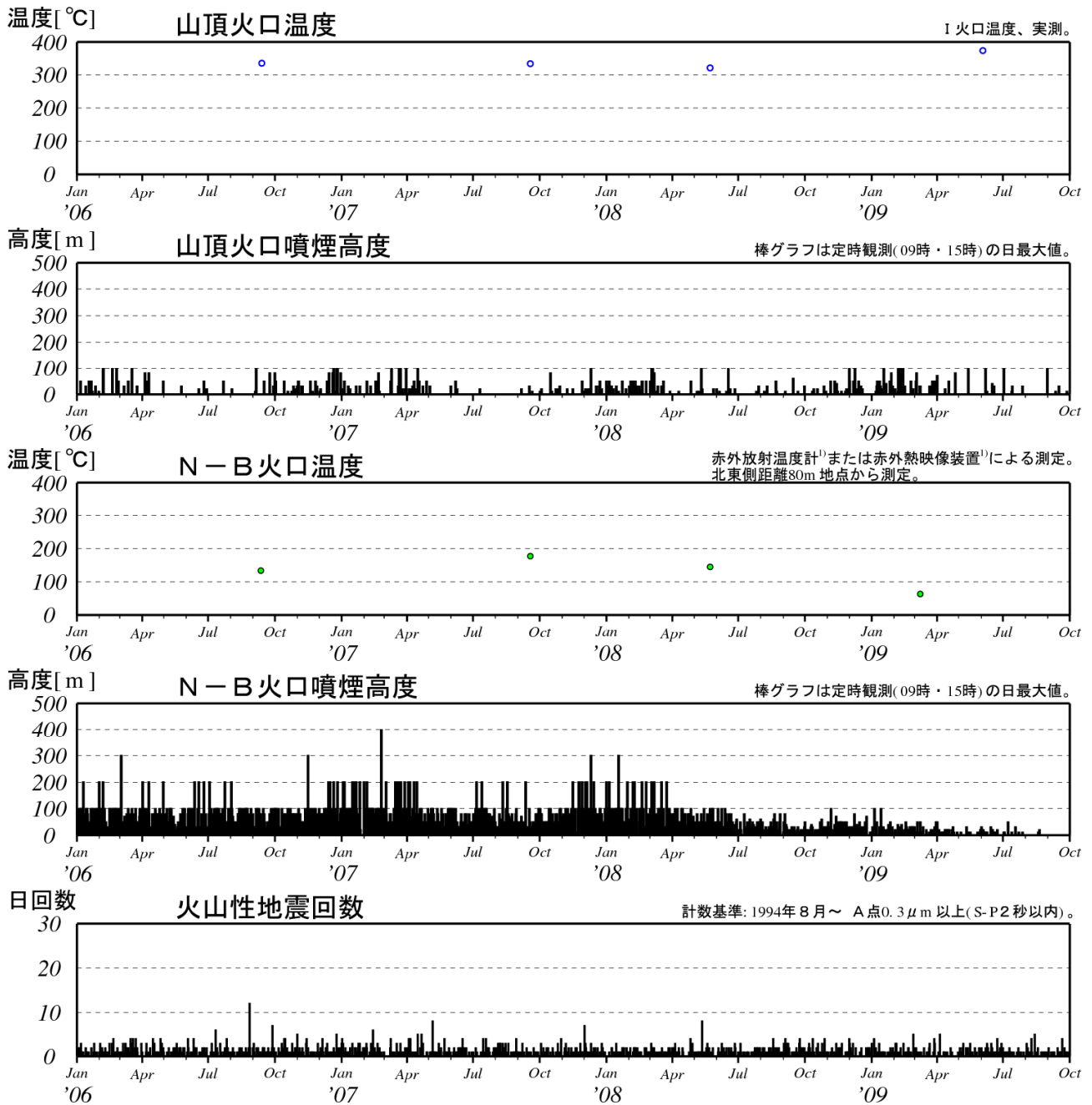
図3 有珠山 最近の火山活動経過図（2006年1月～2009年9月）
