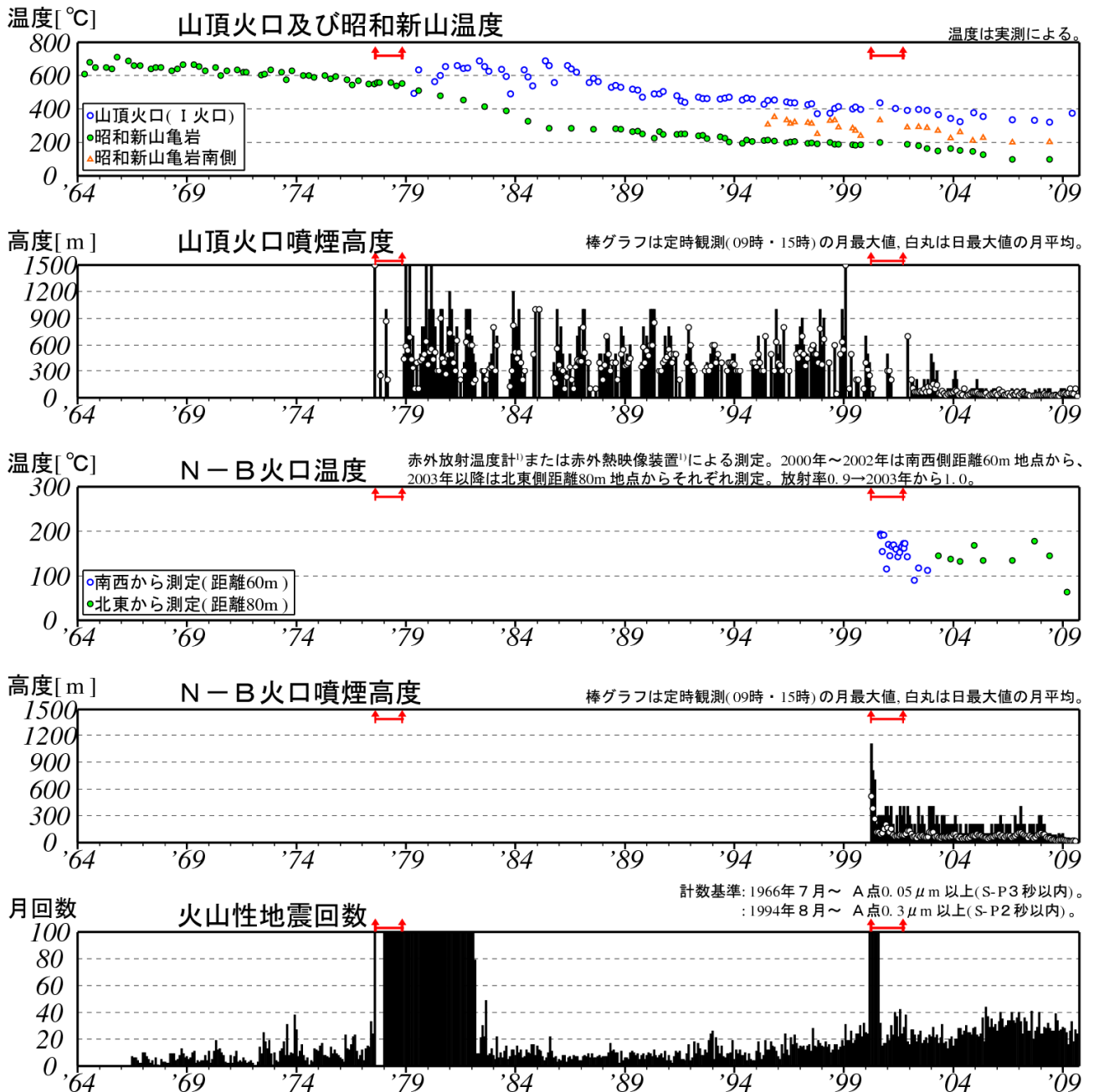
図 2 有珠山 長期の火山活動経過図（1964 年 1 月～2009 年 9 月）
