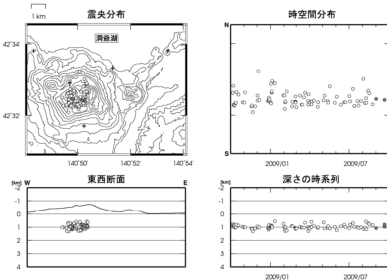
図 4 有珠山 震源分布図（2008 年 10 月～2009 年 9 月、+は地震観測点）
