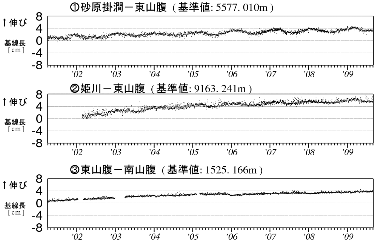
図 5 北海道駒ヶ岳 GPS 連続観測による基線長変化（2001 年 4 月～2009 年 8 月）
