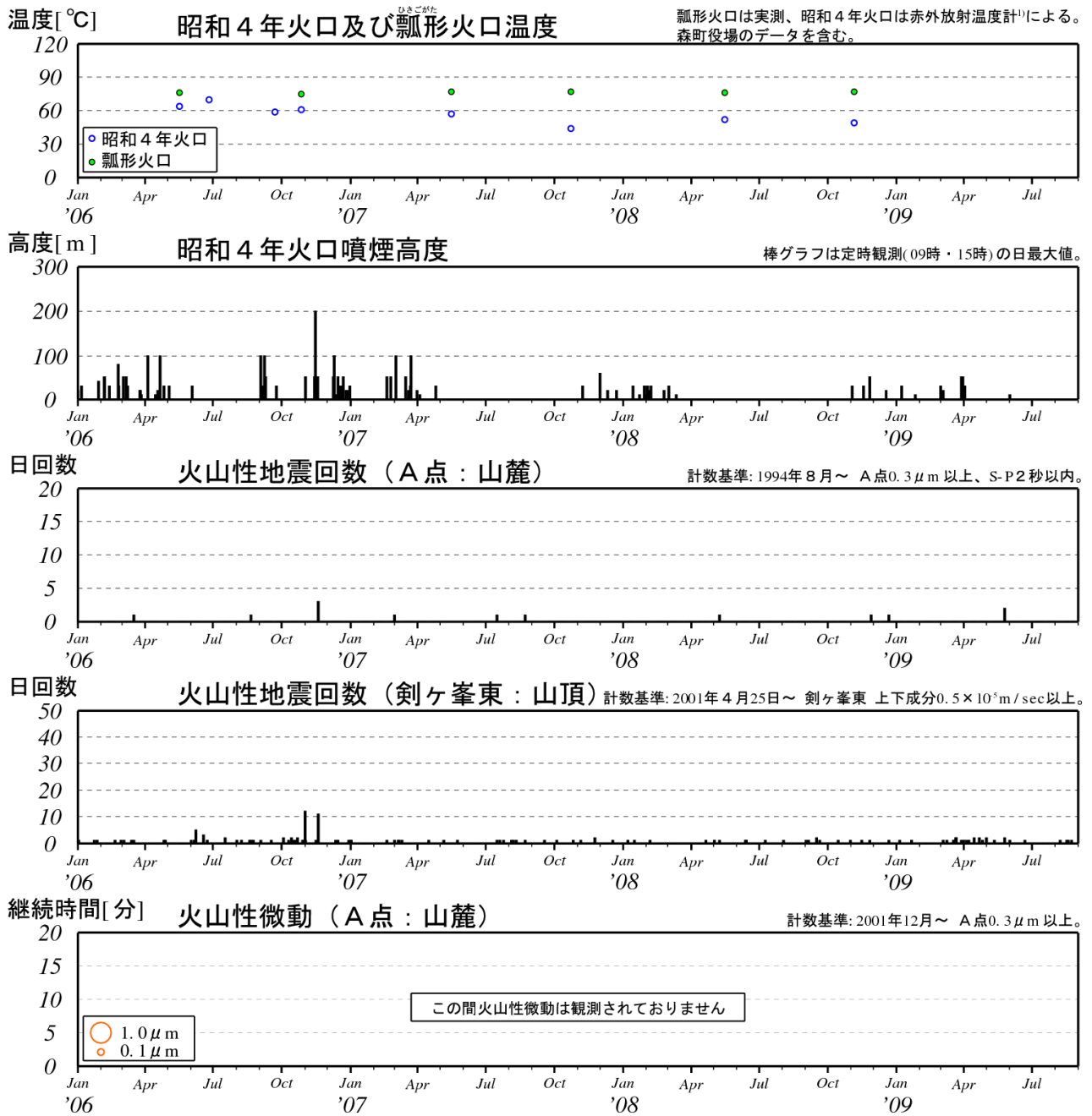
図 3※ 北海道駒ヶ岳 最近の火山活動経過図（2006 年 1 月～2009 年 8 月）
