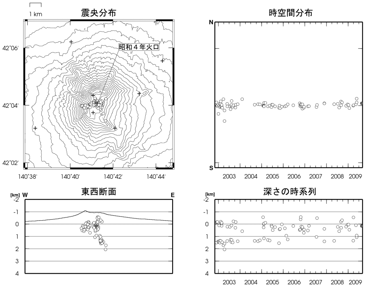
図 4 ※ 北海道駒ヶ岳 震源分布図（2002 年 11 月～2009 年 8 月、+は地震観測点）
