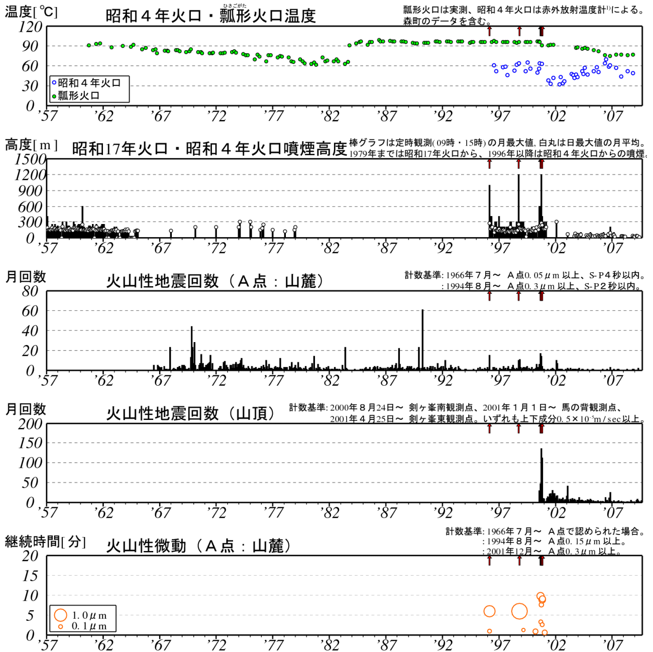
図 2 ※ 北海道駒ヶ岳 長期の火山活動経過図（1957 年 1 月～2009 年 8 月）↑印は噴火
