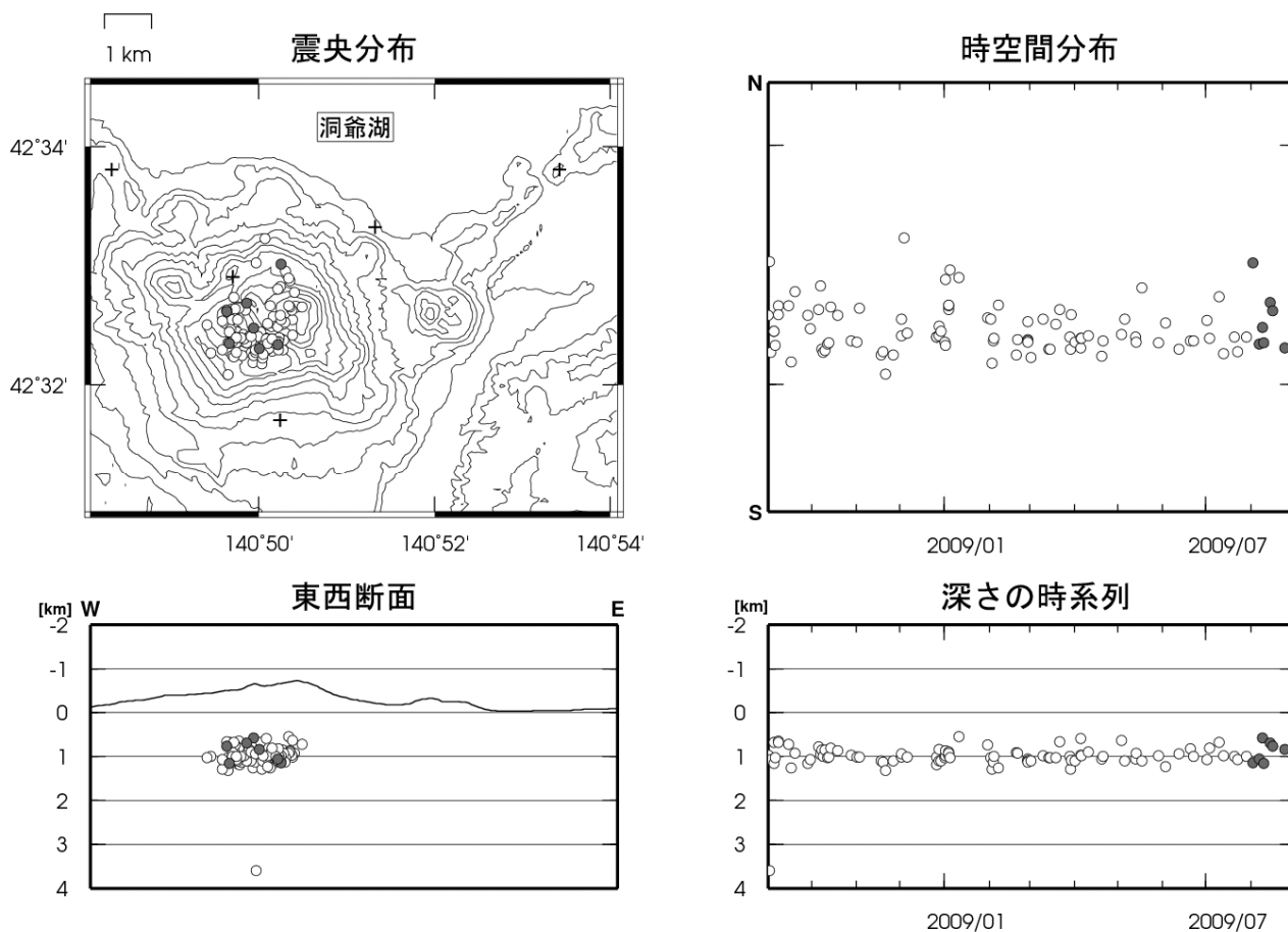
図 4 有珠山 震源分布図（2008 年 9 月～2009 年 8 月、+は地震観測点）
