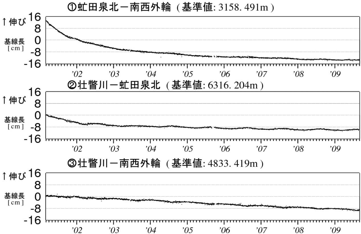
図5 有珠山 GPS 連続観測による基線長変化（2001年3月～2009年8月） グラフの空白部分は欠測 図5の①～③は、図6のGPS基線①～③に対応しています。
