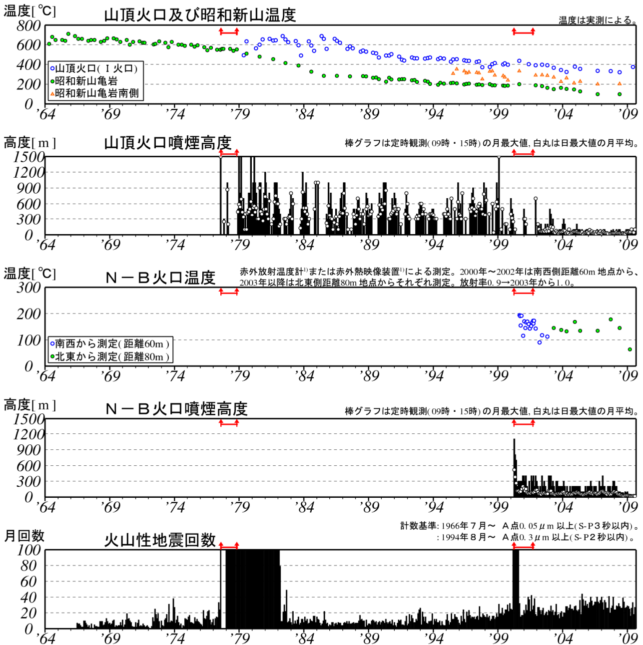
図 2 有珠山 長期の火山活動経過図（1964 年 1 月～2009 年 8 月）
