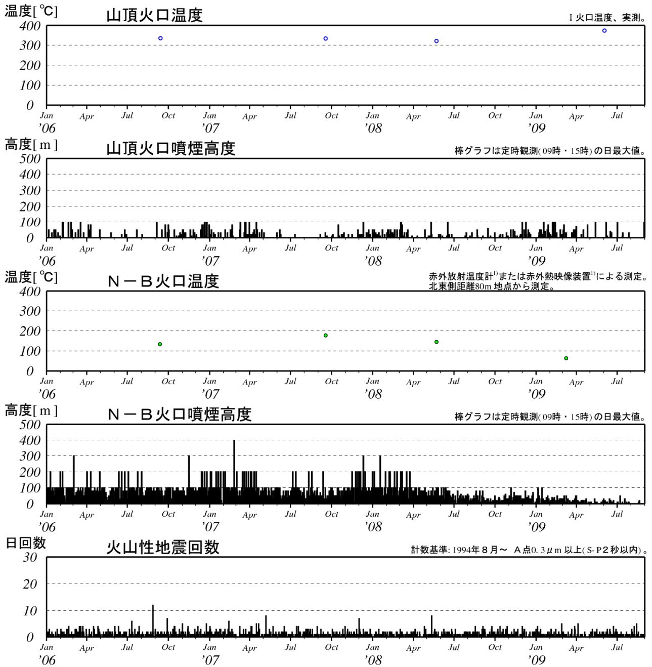
図3 有珠山 最近の火山活動経過図（2006年1月～2009年8月）
