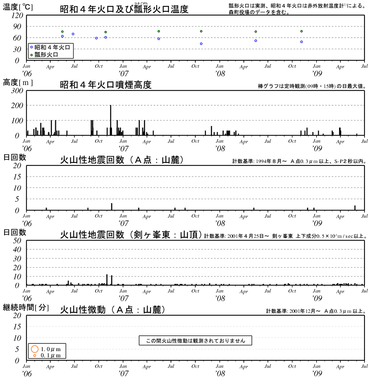
図 3※ 北海道駒ヶ岳 最近の火山活動経過図（2006 年 1 月～2009 年 6 月）
