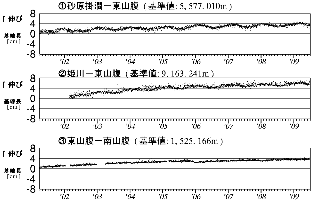
図5 北海道駒ヶ岳 GPS 連続観測による基線長変化（2001 年 4 月～2009 年 6 月）
