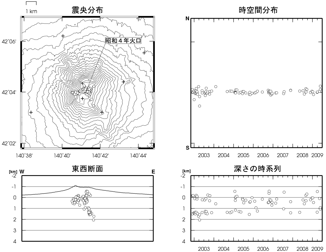
図 4 ※ 北海道駒ヶ岳 震源分布図（2002 年 11 月～2009 年 6 月、+は地震観測点）
