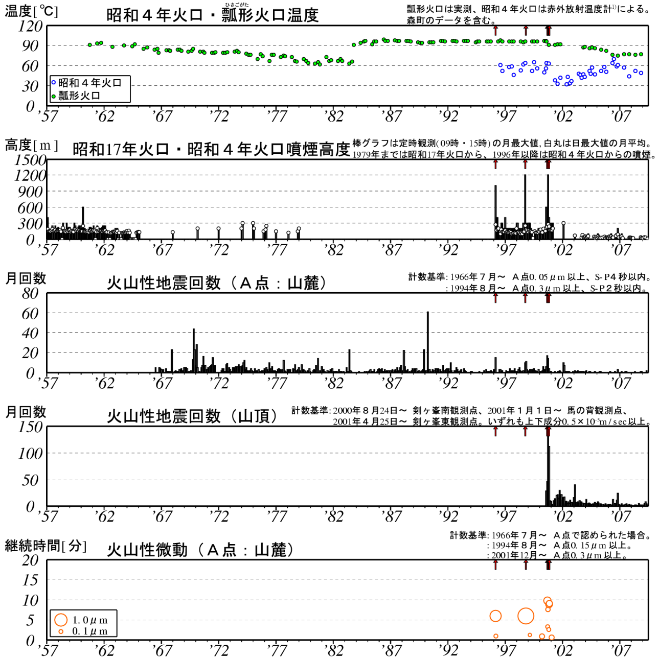
図 2 ※ 北海道駒ヶ岳 長期の火山活動経過図（1957 年 1 月～2009 年 6 月）↑印は噴火
