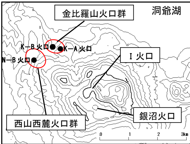
図 4 有珠山 火口周辺図
