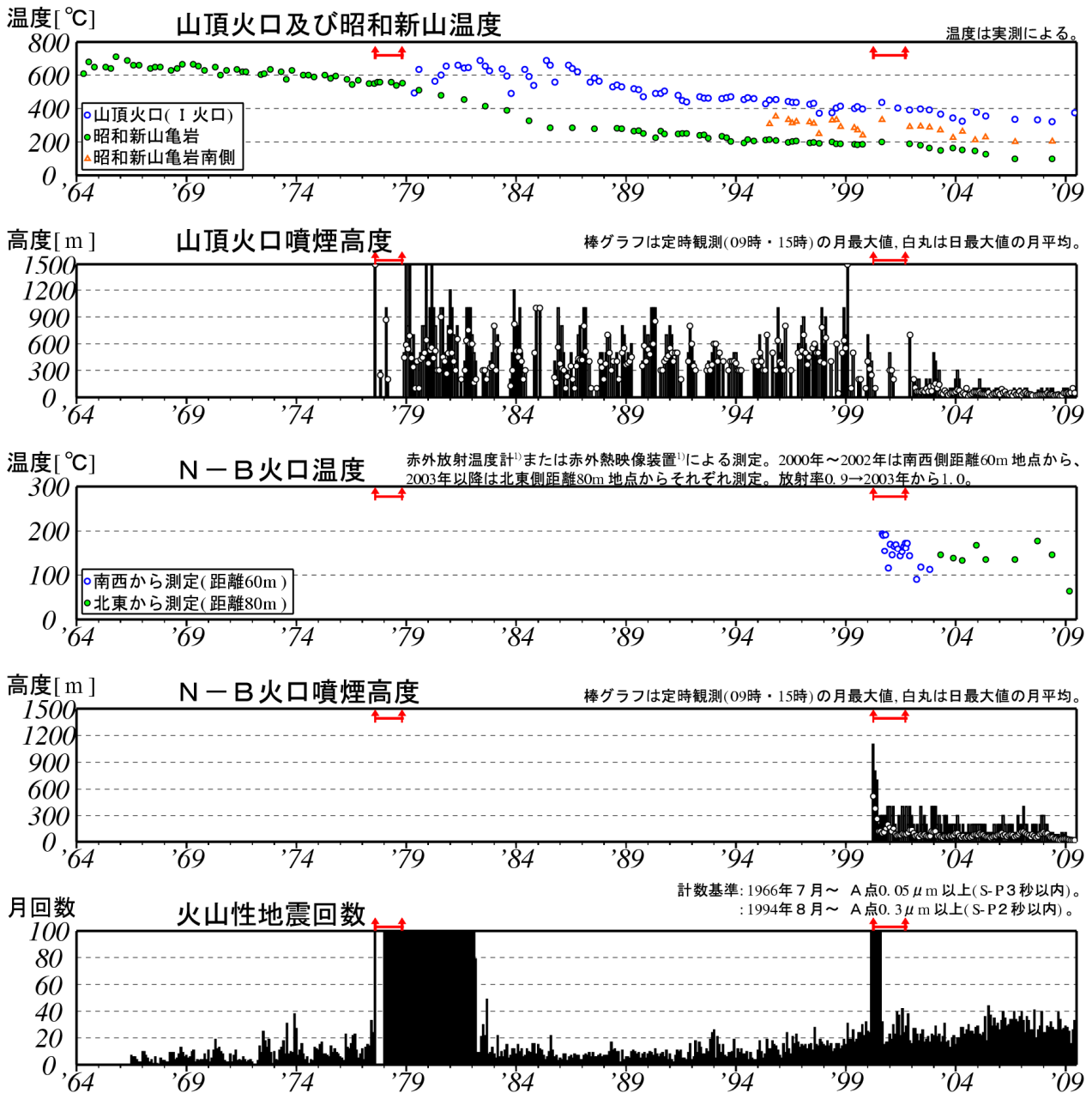
図2 有珠山 長期の火山活動経過図（1964年1月～2009年6月）
