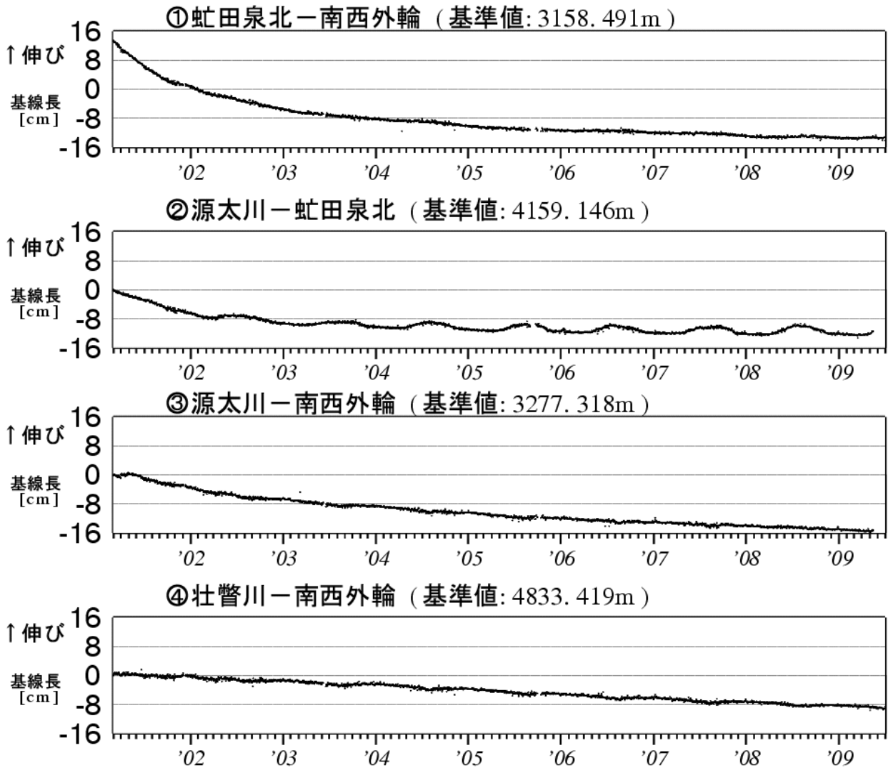
図9 有珠山 GPS 連続観測による基線長変化（2001年3月～2009年6月） グラフの空白部分は欠測 図9の①～④は、図10のGPS基線①～④に対応しています。
