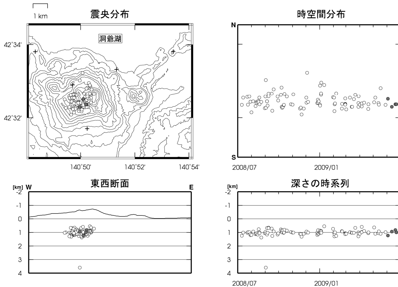
図 8 有珠山 震源分布図（2008 年 7 月～2009 年 6 月、+は地震観測点）
