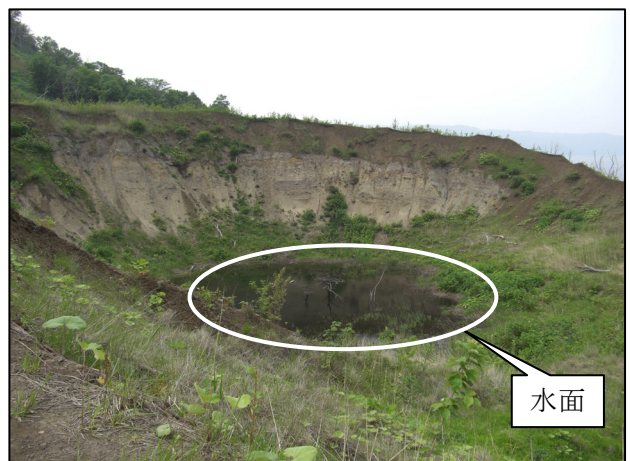
図 5 有珠山 N-B 火口の状況 (2009 年 6 月 3 日 南側より撮影)
