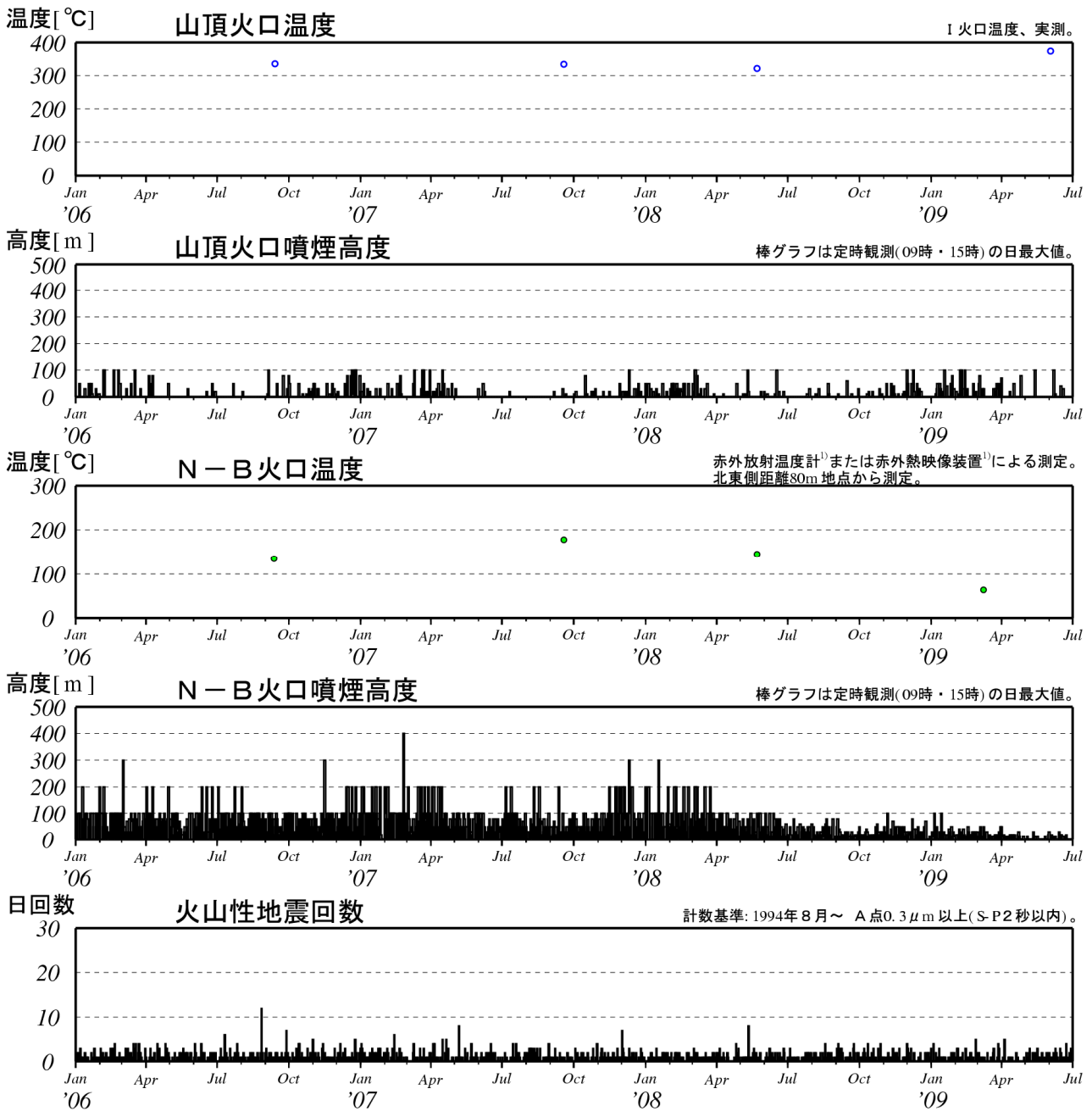
図3 有珠山 最近の火山活動経過図（2006年1月～2009年6月）
