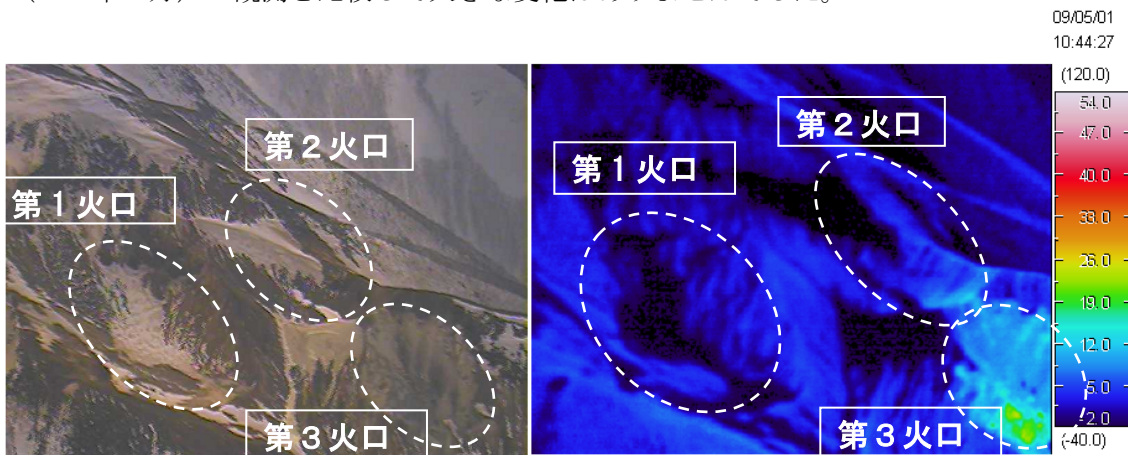
図 1 丸山 赤外熱映像装置 1) による北西斜面火口列の地表面温度分布 (5 月 1 日 図 2 の矢印方向から撮影 北海道開発局の協力による)
