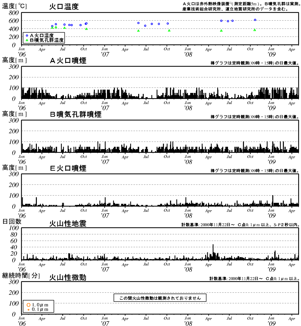
図 3※ 樽前山 最近の火山活動経過図 (2006 年 1 月～2009 年 4 月)
