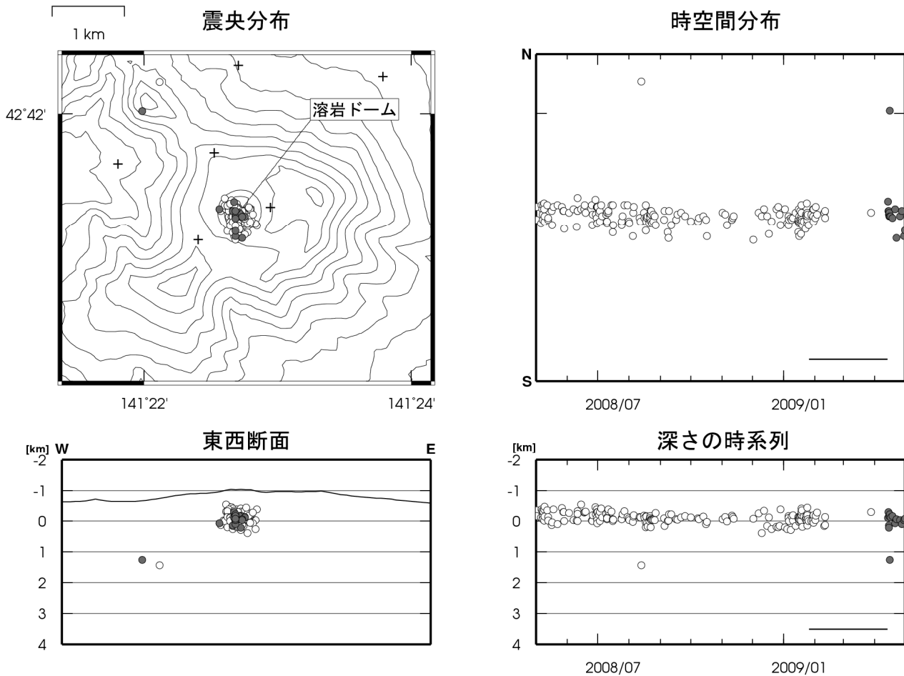
図 4※ 樽前山 震源分布図 (2008 年 5 月~2009 年 4 月、+は地震観測点)
