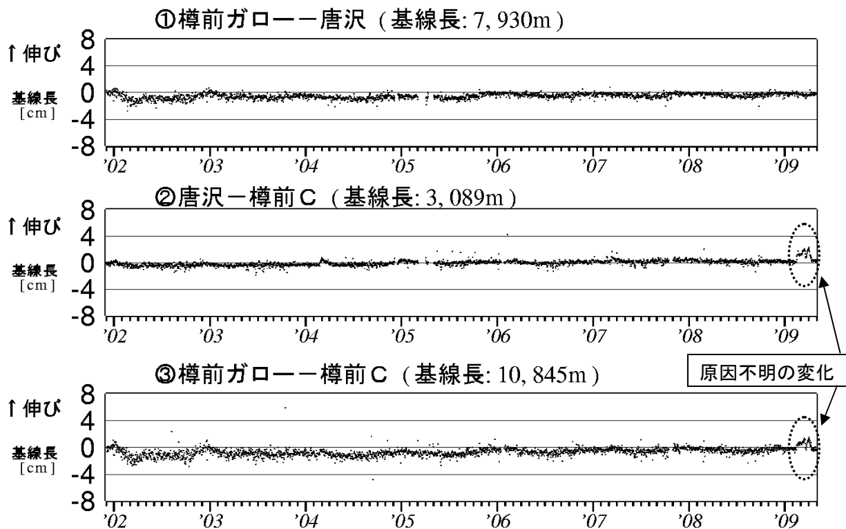
図5 樽前山 GPS 連続観測による基線長変化 (2001 年 12 月～2009 年 4 月) グラフの空白部分は欠測
