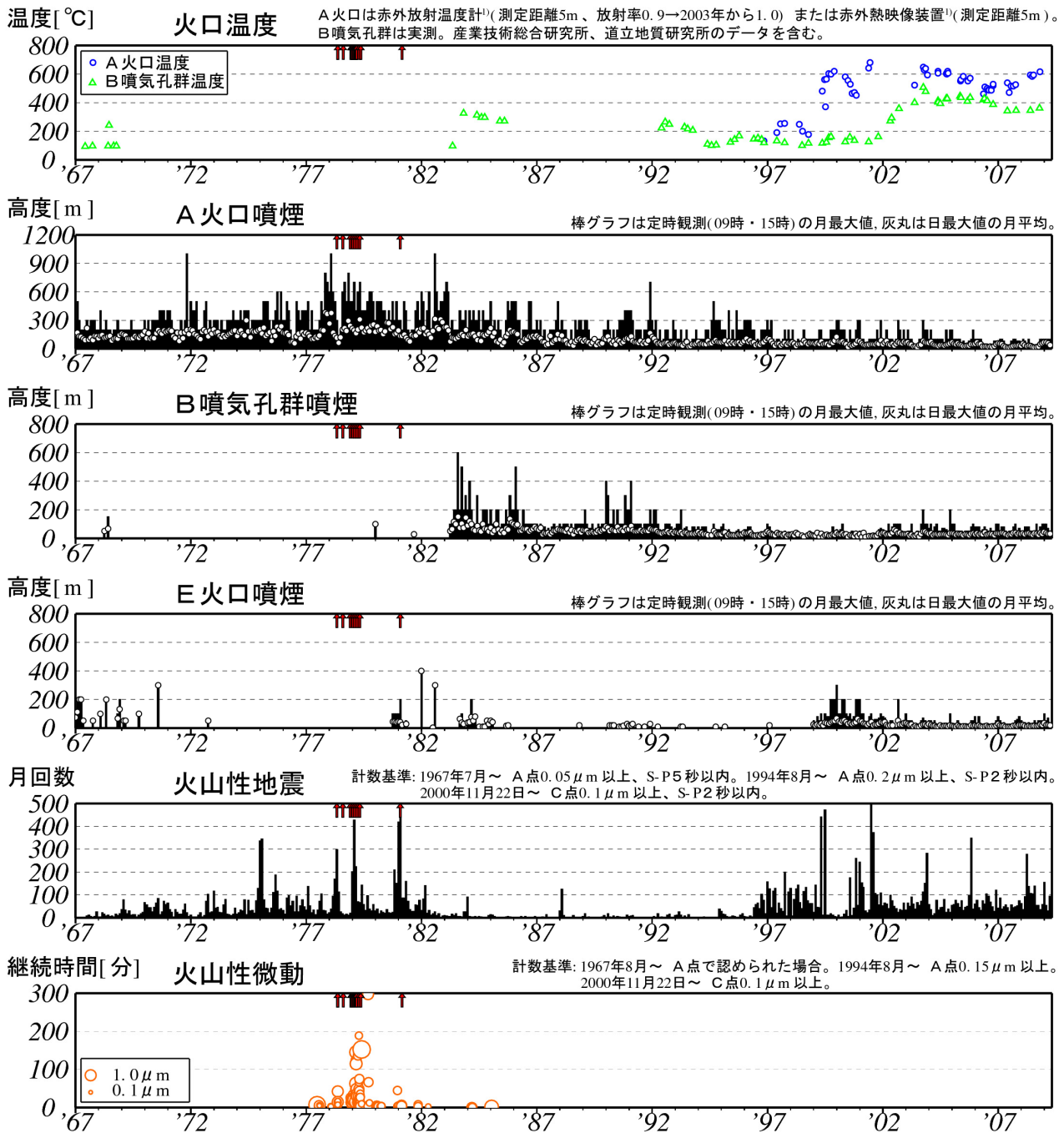
図 2※ 樽前山 長期の火山活動経過図（1967 年 1 月～2009 年 4 月） ↑印は噴火
