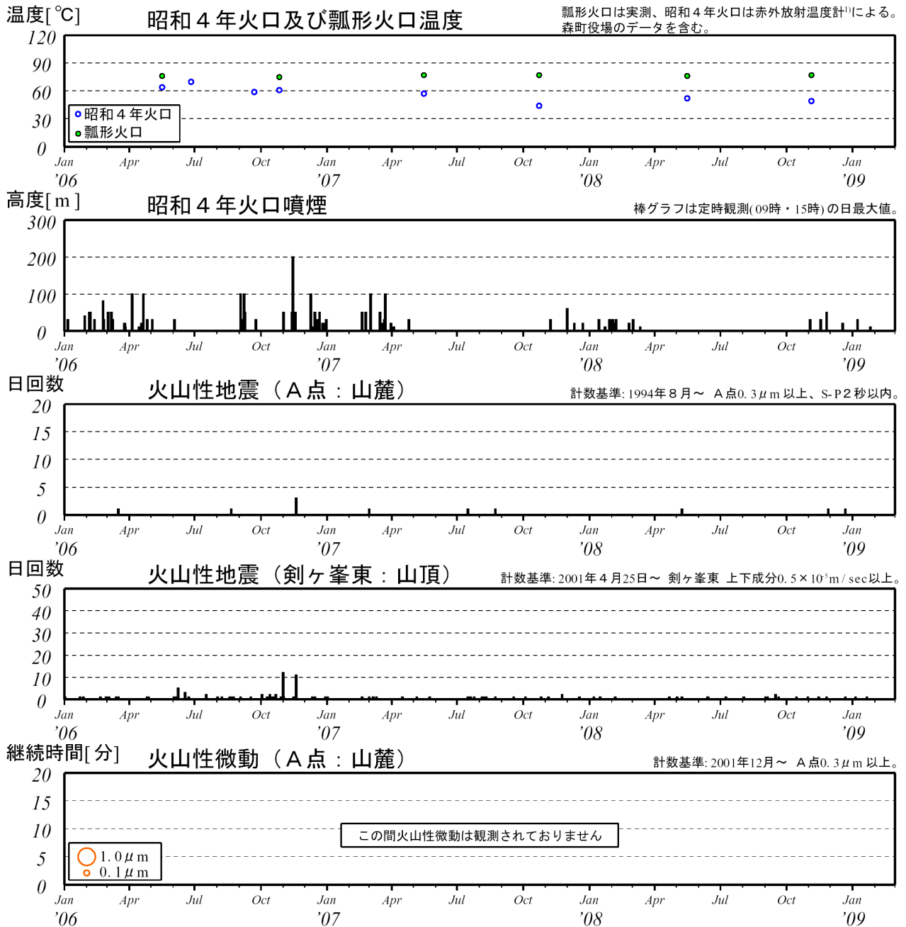
図 3※ 北海道駒ヶ岳 最近の火山活動経過図（2006 年 1 月～2009 年 2 月）
