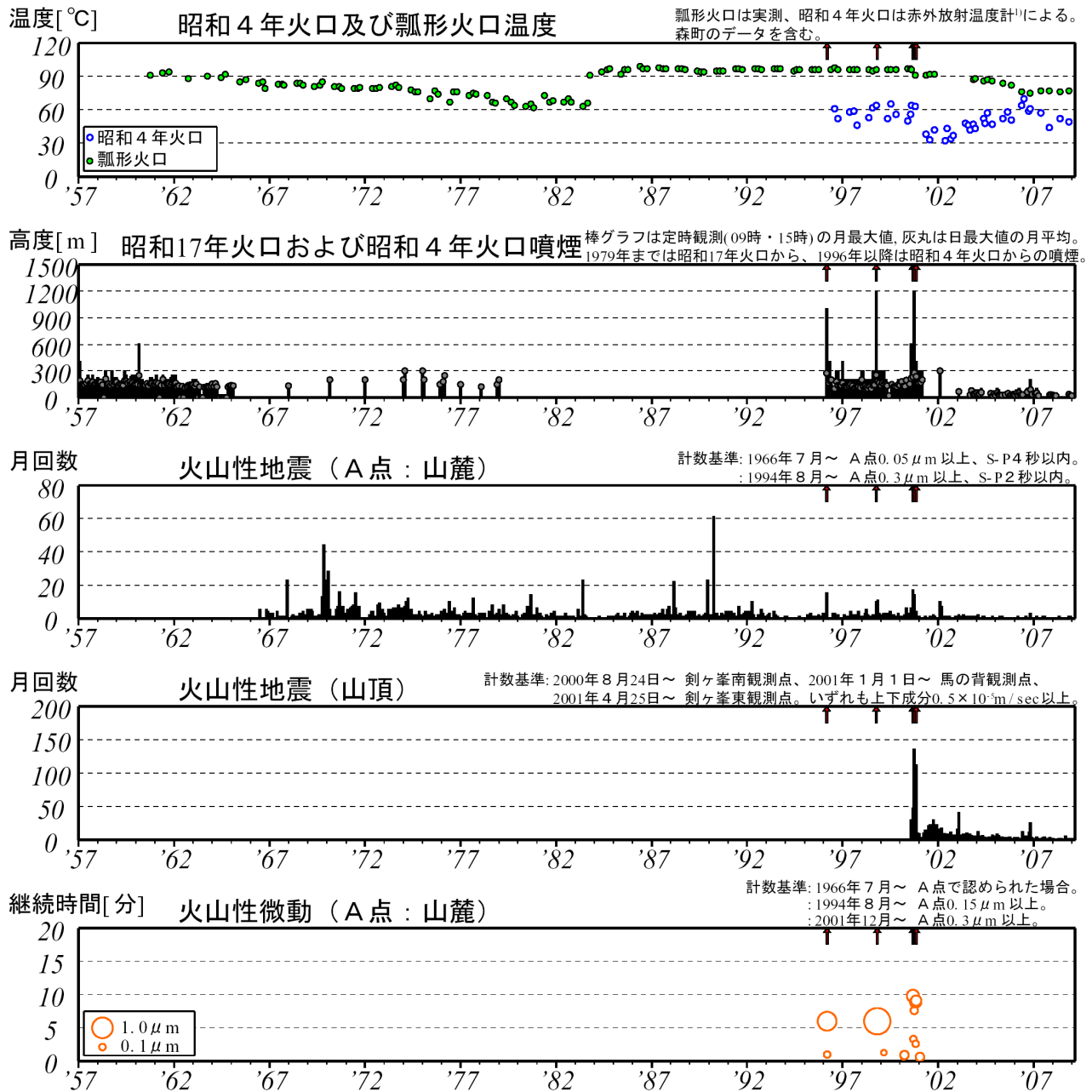
図2※ 北海道駒ヶ岳 長期の火山活動経過図（1957年1月～2009年2月）↑印は噴火
