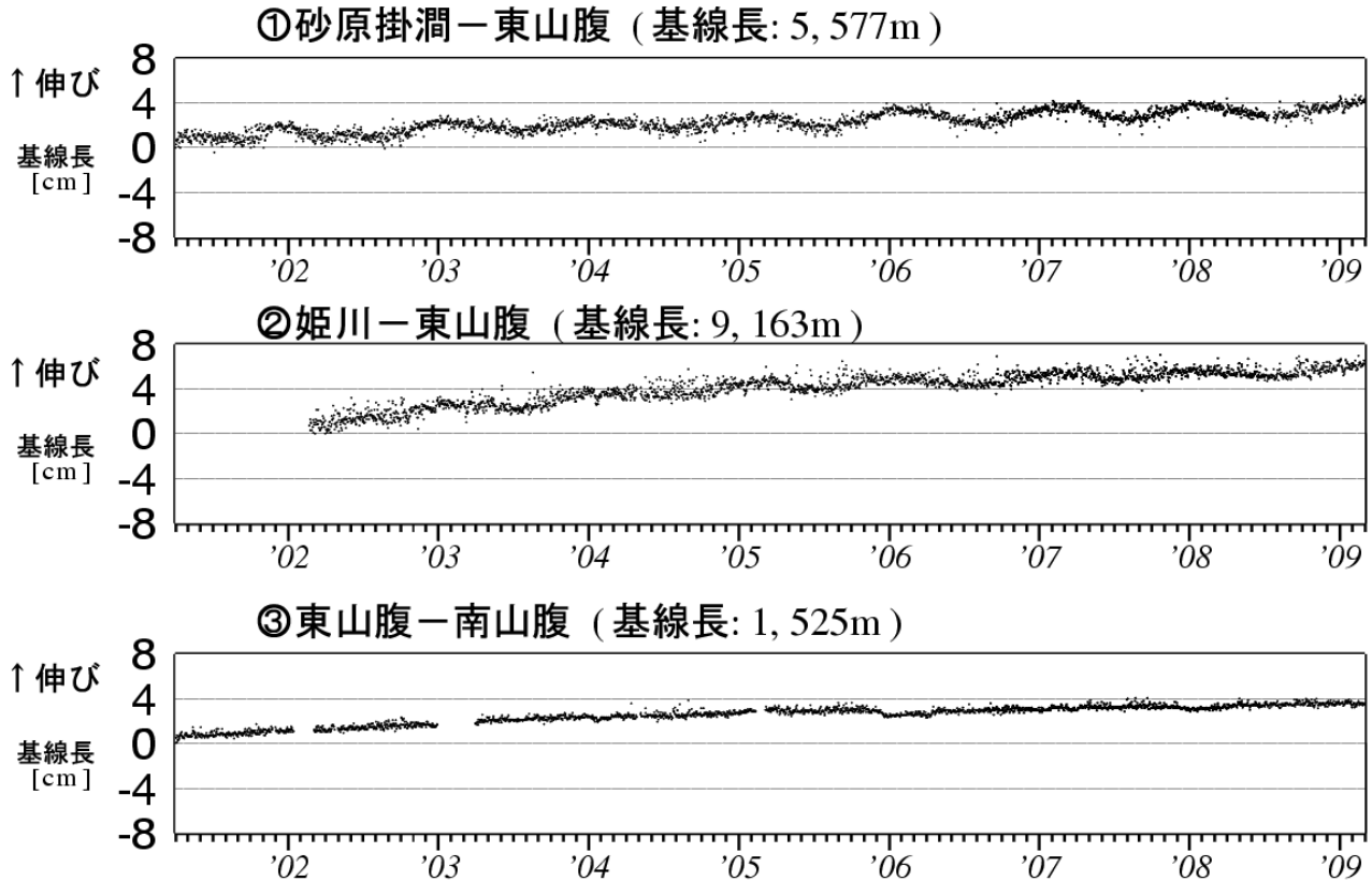
図 5 北海道駒ヶ岳 GPS 連続観測による基線長変化（2001 年 4 月～2009 年 2 月）
