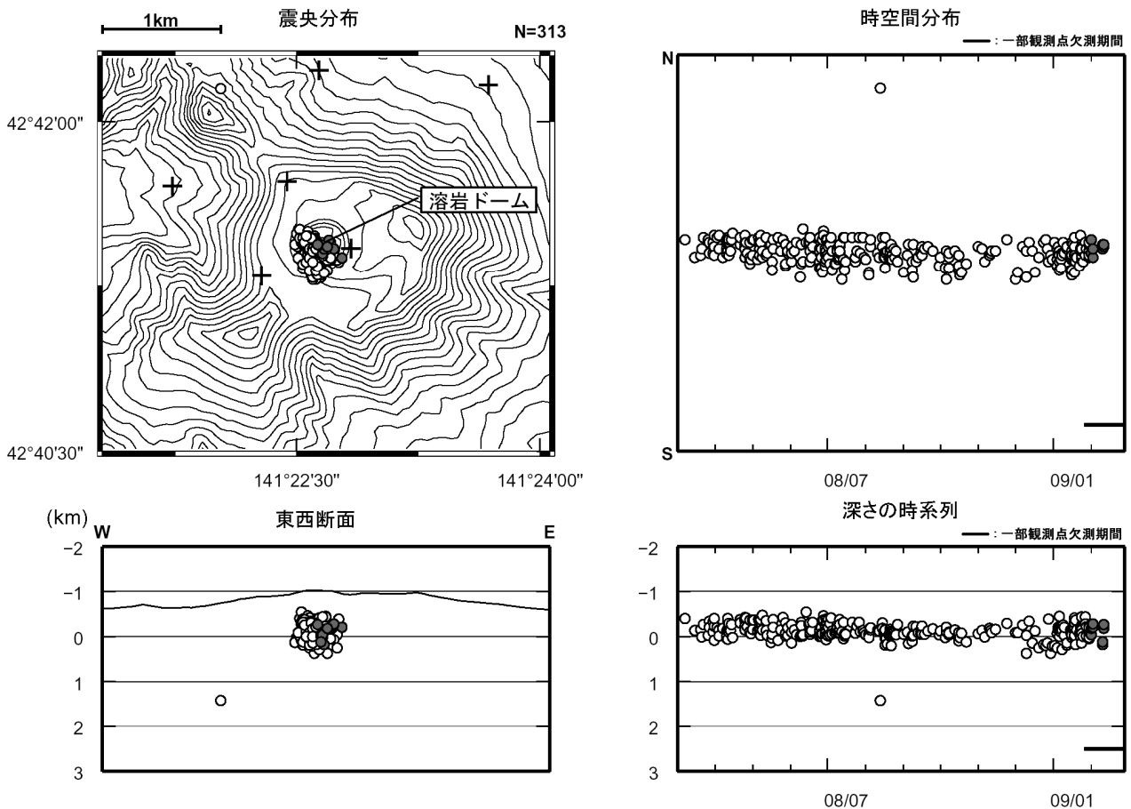
図 4※ 樽前山 震源分布図 (2008 年 3 月～2009 年 2 月、+は地震観測点)
