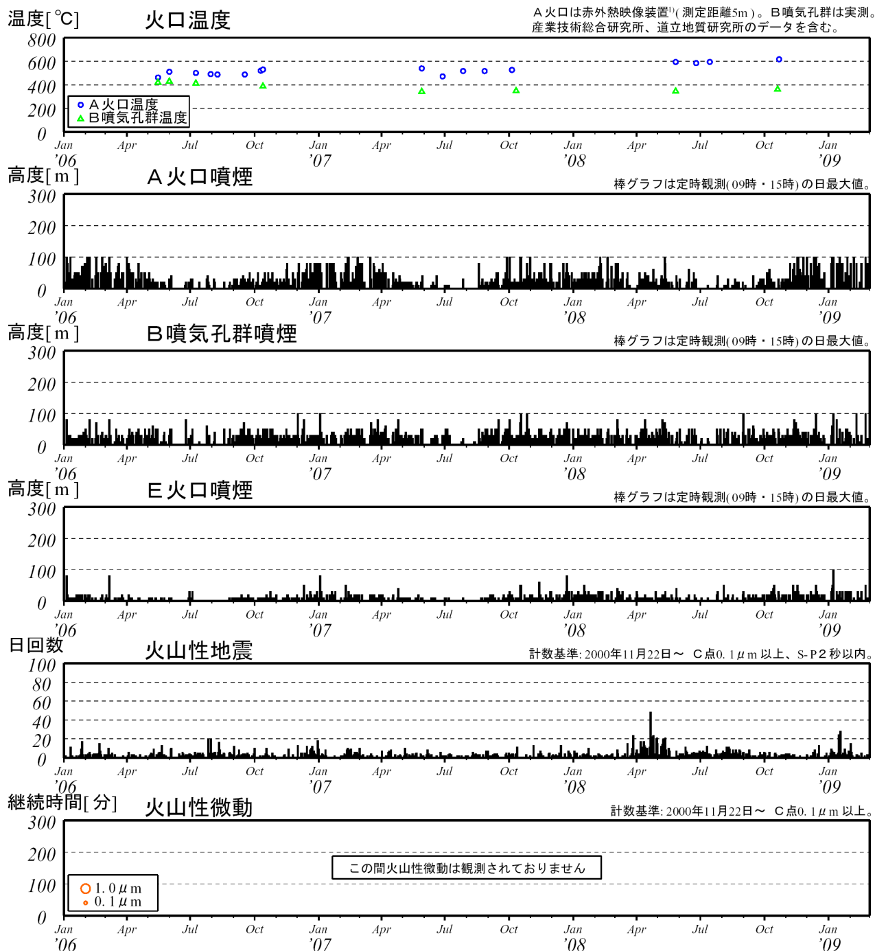
図 3※ 樽前山 最近の火山活動経過図 (2006 年 1 月～2009 年 2 月)
