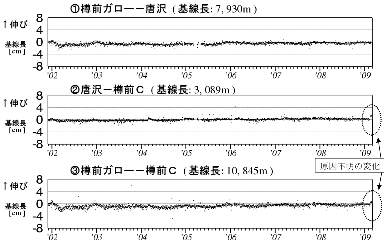
図5 樽前山 GPS 連続観測による基線長変化 (2001 年 12 月～2009 年 2 月) グラフの空白部分は欠測
