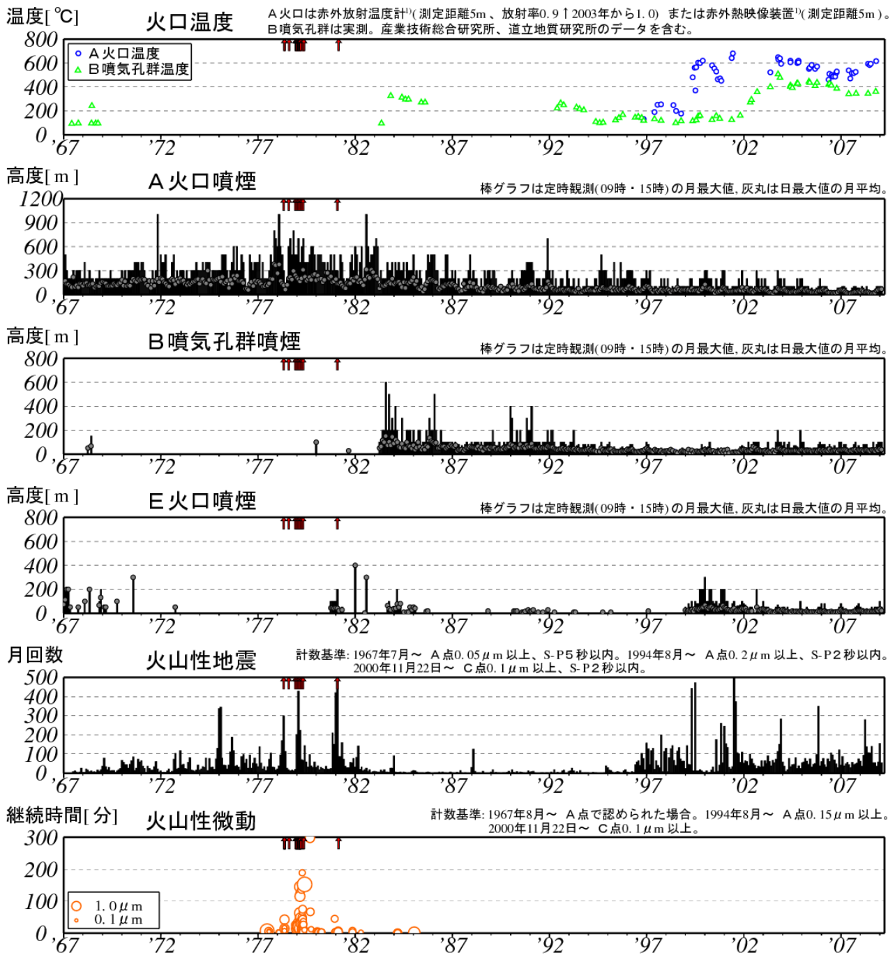
図2※ 樽前山 長期の火山活動経過図 (1967年1月～2009年2月) ↑印は噴火
