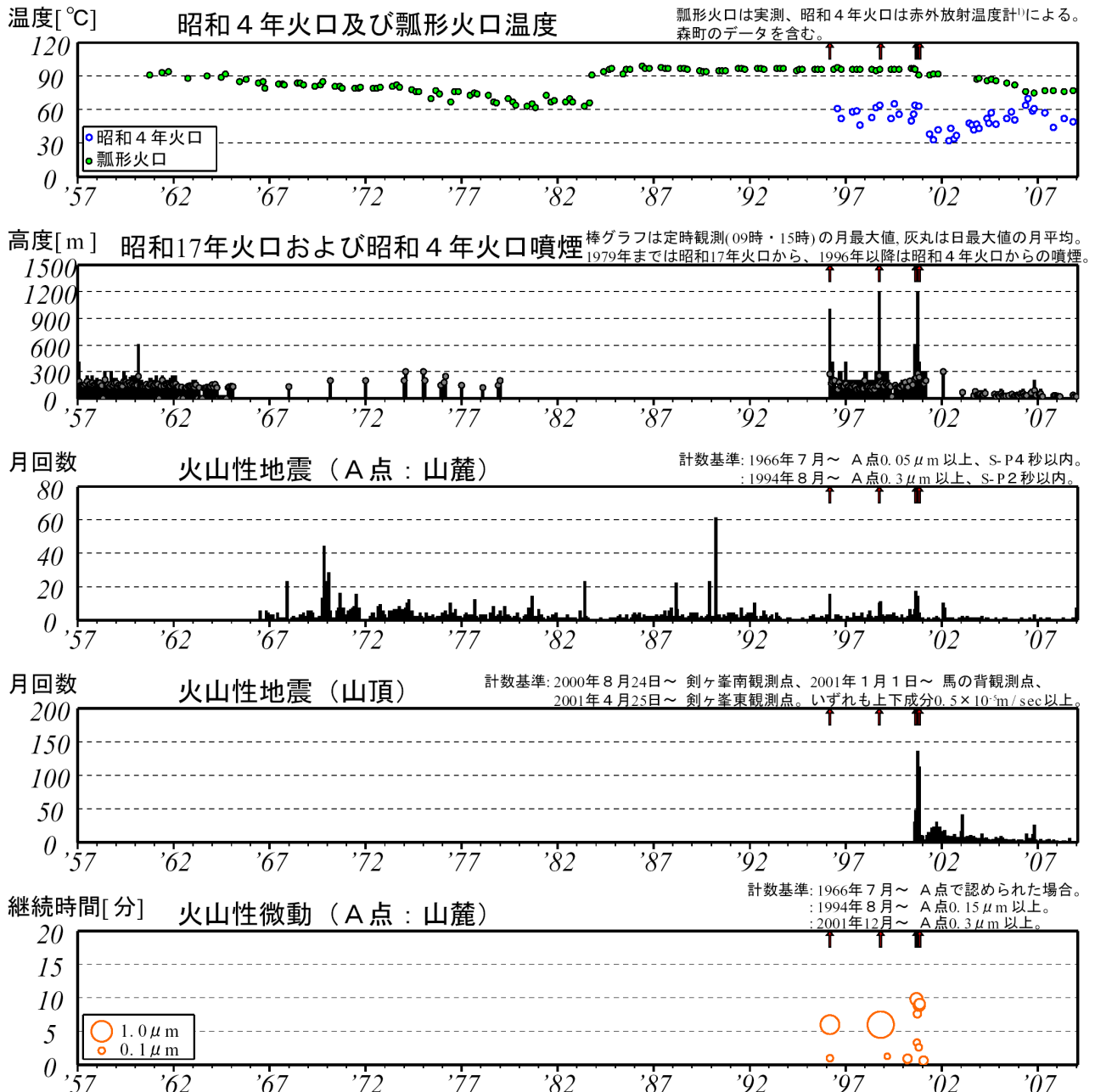
図2※ 北海道駒ヶ岳 長期の火山活動経過図（1957年1月～2009年1月） ↑印は噴火
