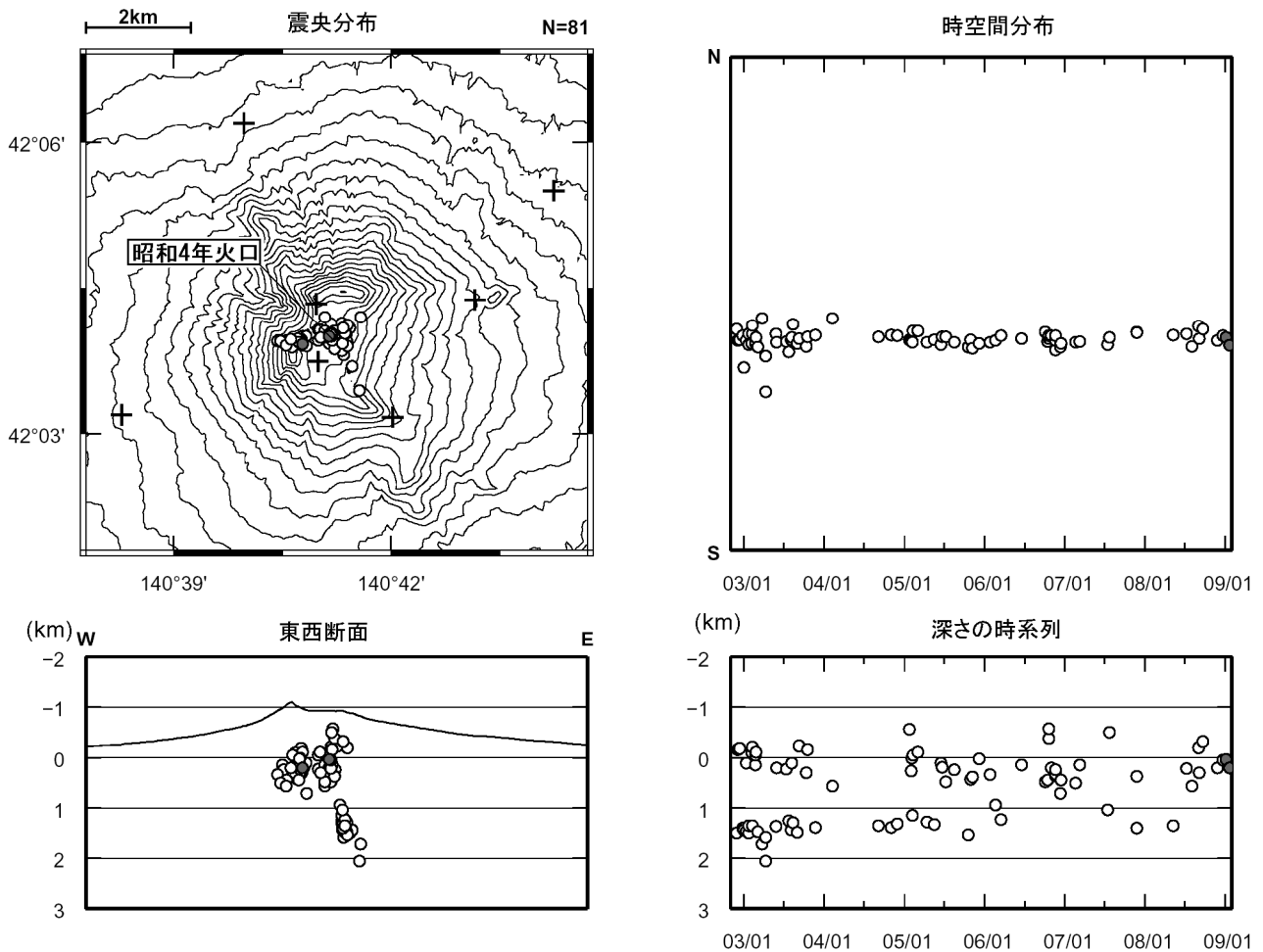
図 4※ 北海道駒ヶ岳 震源分布図（2002 年 11 月～2009 年 1 月、+は地震観測点）
