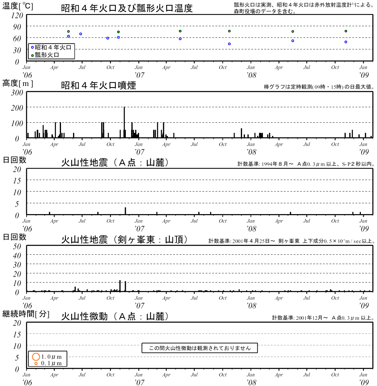
図 3※ 北海道駒ヶ岳 最近の火山活動経過図（2006 年 1 月～2009 年 1 月）
