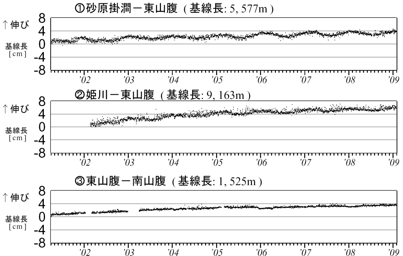
図5 北海道駒ヶ岳 GPS 連続観測による基線長変化（2001 年 4 月～2009 年 1 月）
