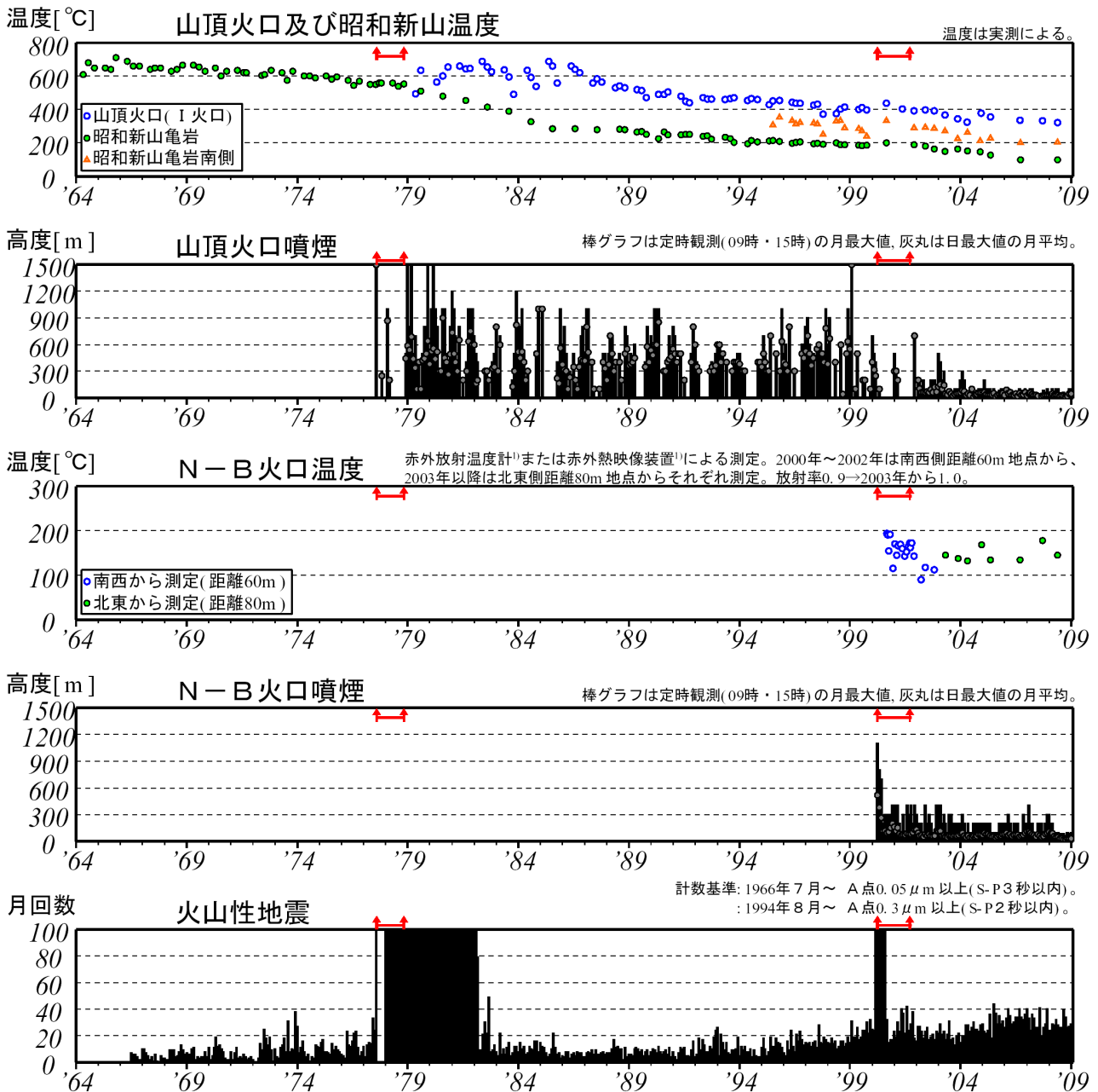
図2 有珠山 長期の火山活動経過図（1964年1月～2009年1月）
