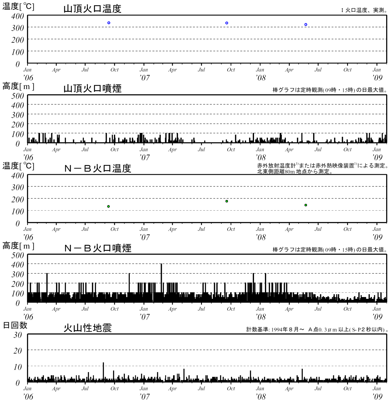
図3 有珠山 最近の火山活動経過図（2006年1月～2009年1月） ・2000年9月以降、地震回数は一日あたり概ね5回以下で推移しています。
