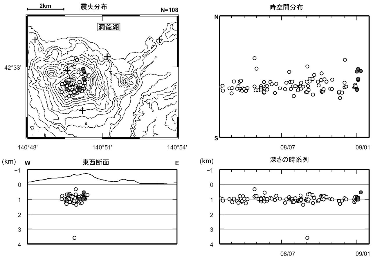
図 4 有珠山 震源分布図（2008 年 2 月～2009 年 1 月、+は地震観測点）
