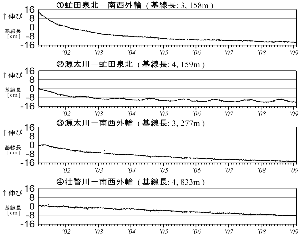
図 5 有珠山 GPS 連続観測による基線長変化（2001 年 3 月～2009 年 1 月） グラフの空白部分は欠測 図 5 の①～④は、図 6 の GPS 基線①～④に対応しています。
